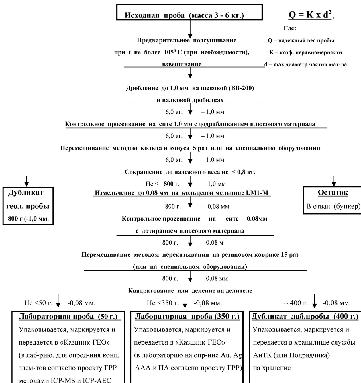
Рис. 5.3 Схема обработки проб №2
