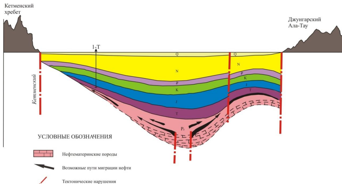
Рисунок 8. Разрез Восточно-Илийского прогиба
