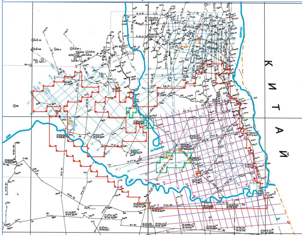
Рисунок 10. Схема размещения проектных 2Д сеймопрофилей
