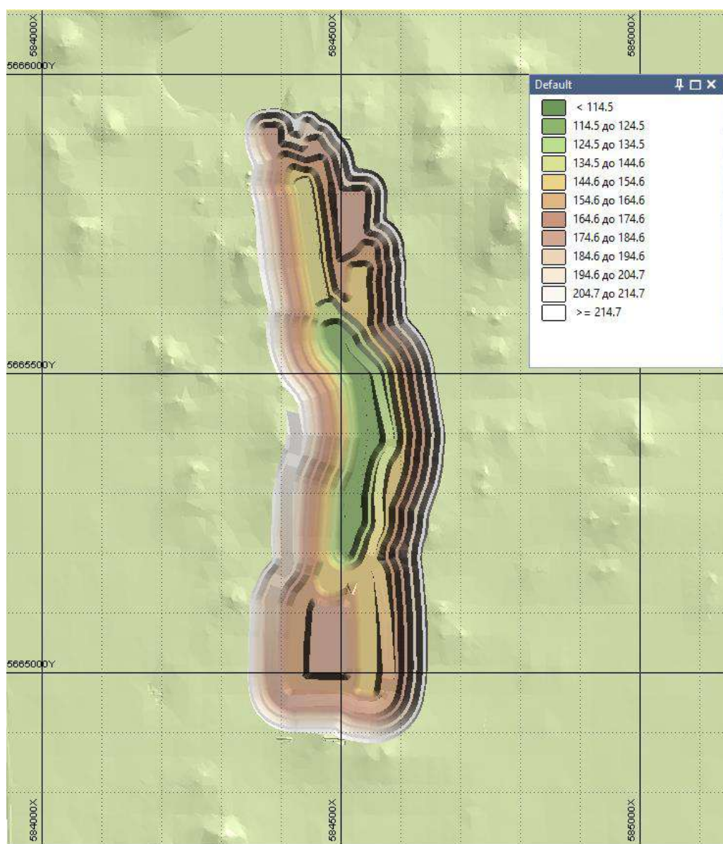
Рис. 1.8 – План Карьера на конец отработки
