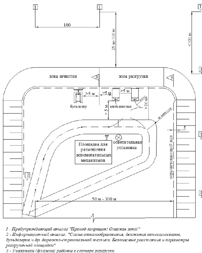
Рис. 1.9. – Схема бульдозерного отвалообразования
