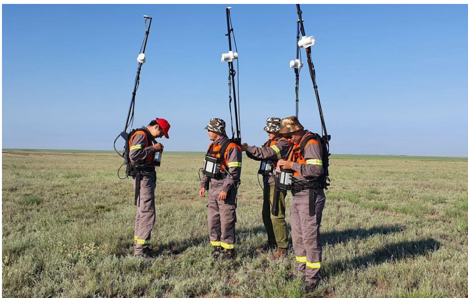
Рисунок 6.3 – Выполнение наземной магниторазведки с помощью модульного магнитометра GSM-19W (Канада)
