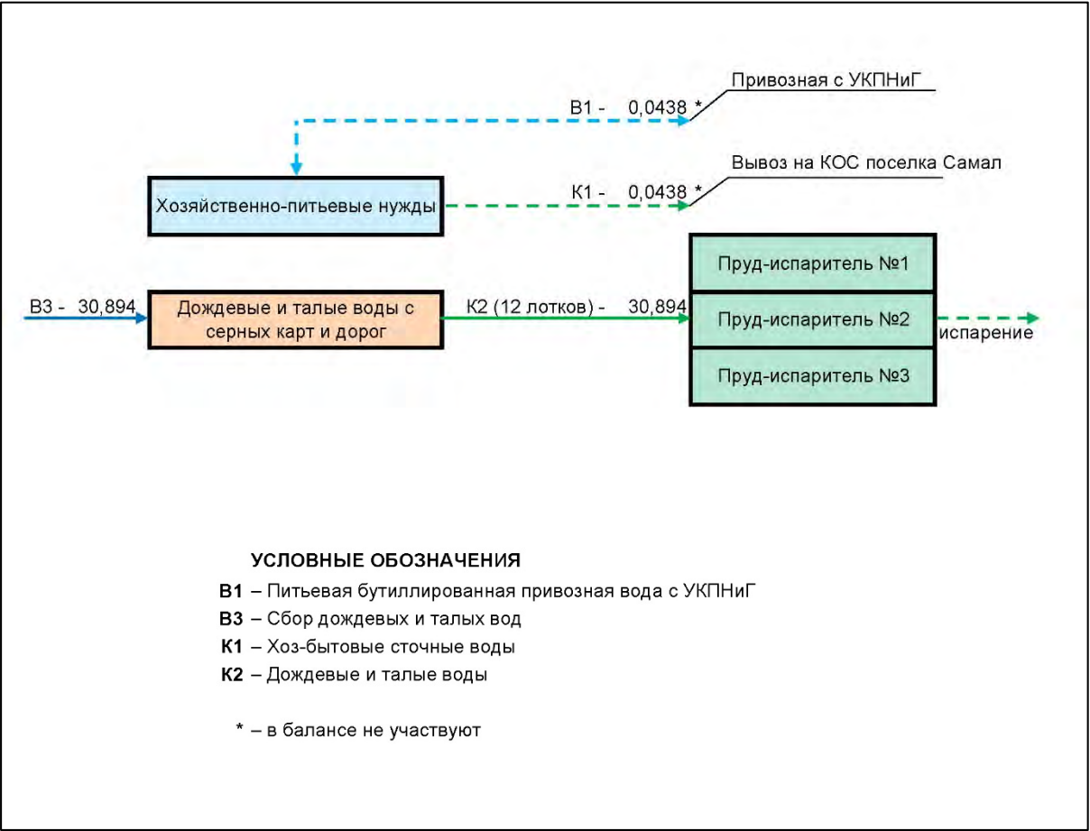
Рисунок 4.1 Балансовая схема водопотребления и водоотведения на 2026 г., тыс. м³/год
