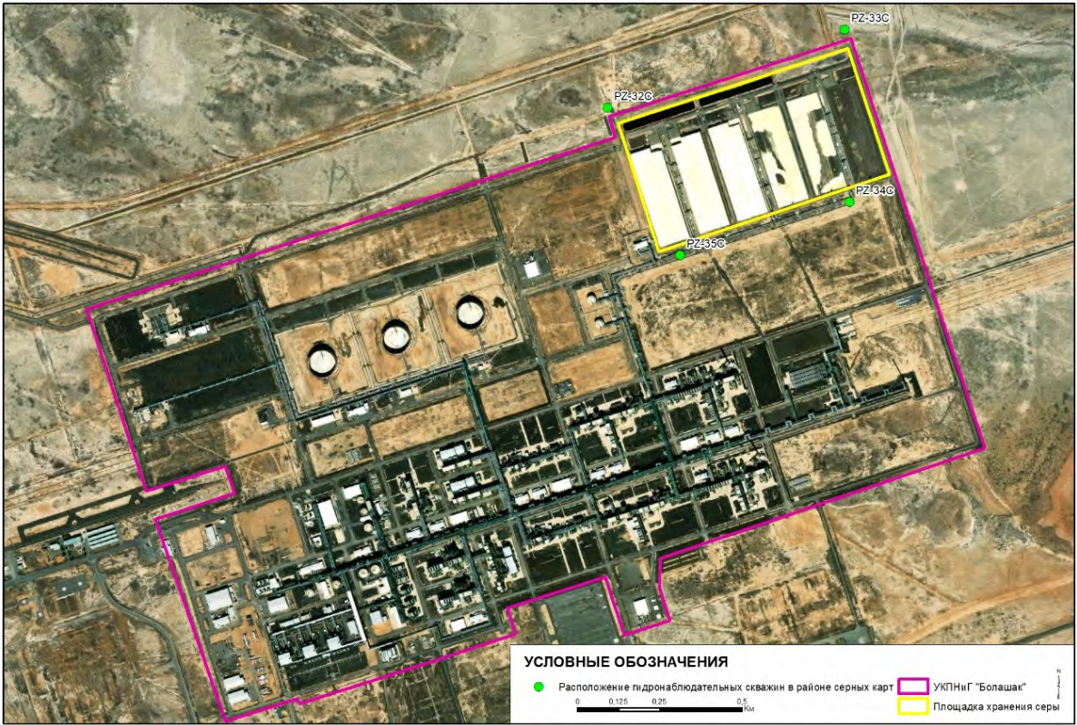
Рисунок 3.1 Карта - схема гидронаблюдательных скважин PZ-32C, PZ-33C, PZ-34C, PZ-35C в районе прудов-испарителей серных карт
