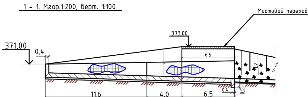
Рис.4- Расчетная схема сливных каналов
