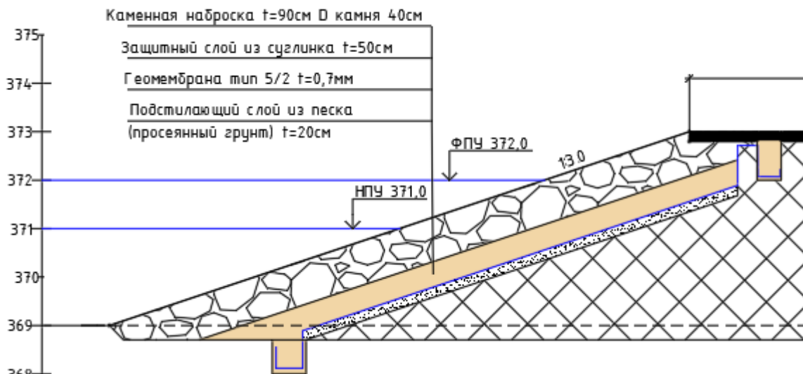
Рис. 5-Конструкция верхового откоса
