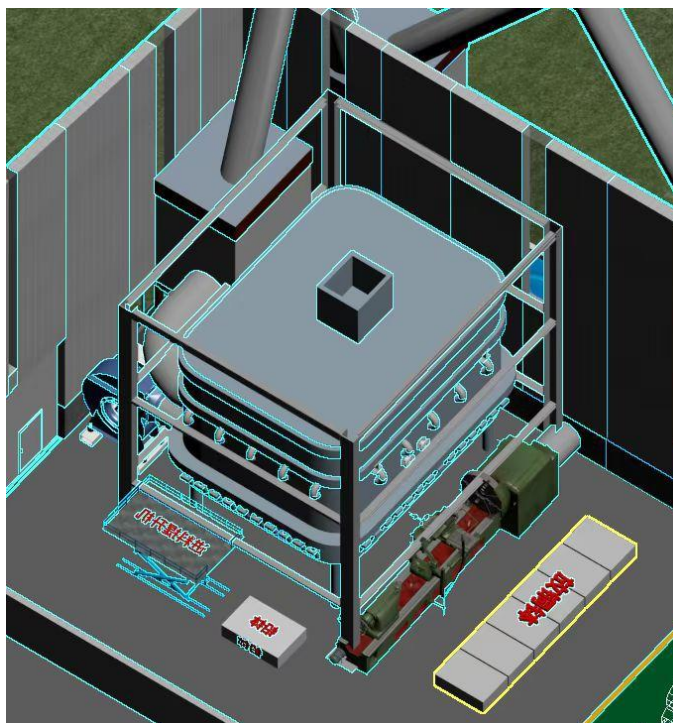
Рисунок 5.2 - Общий вид печи
