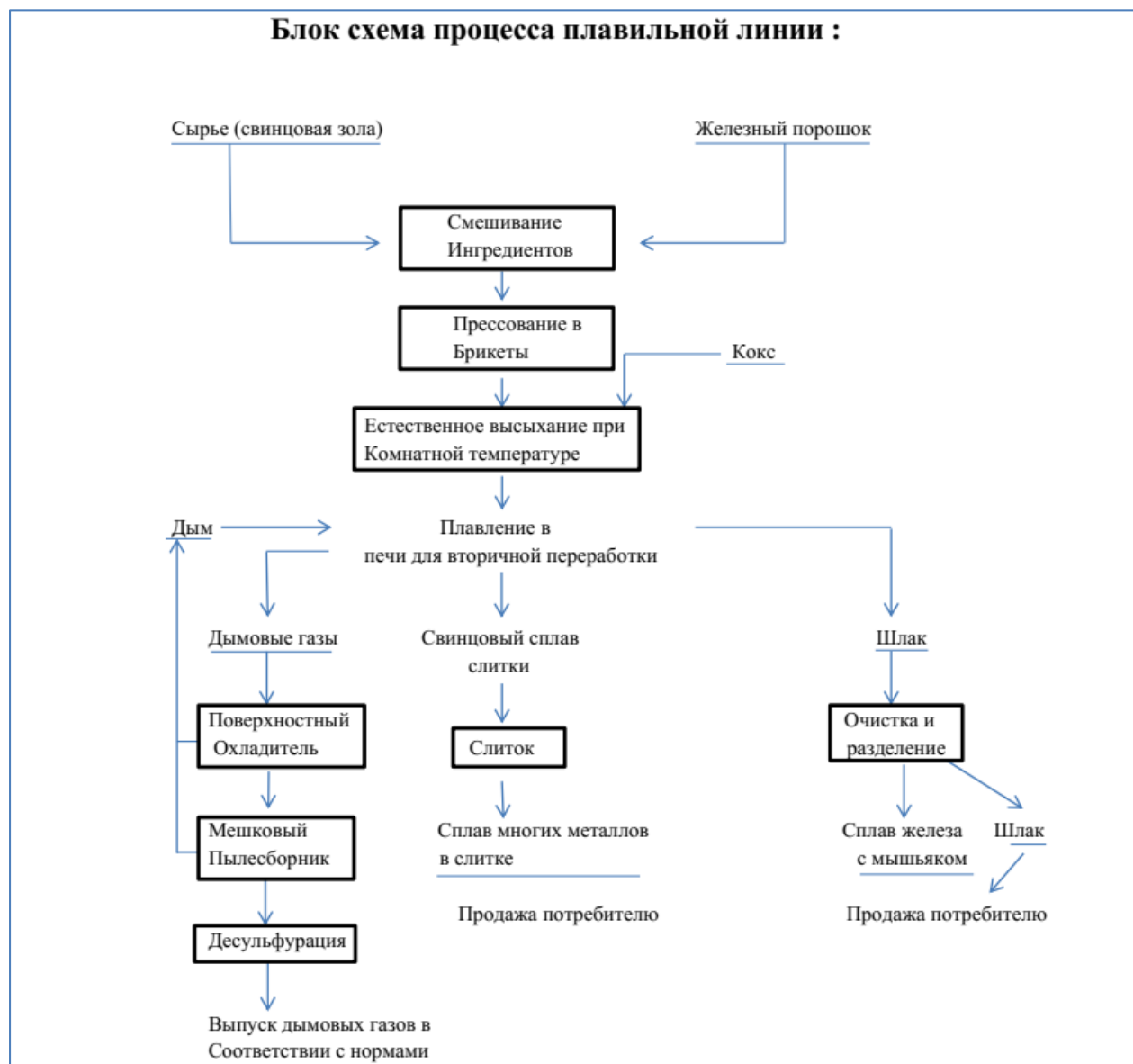
Рисунок 5.3 - Схема технологического оборудования и технологии
