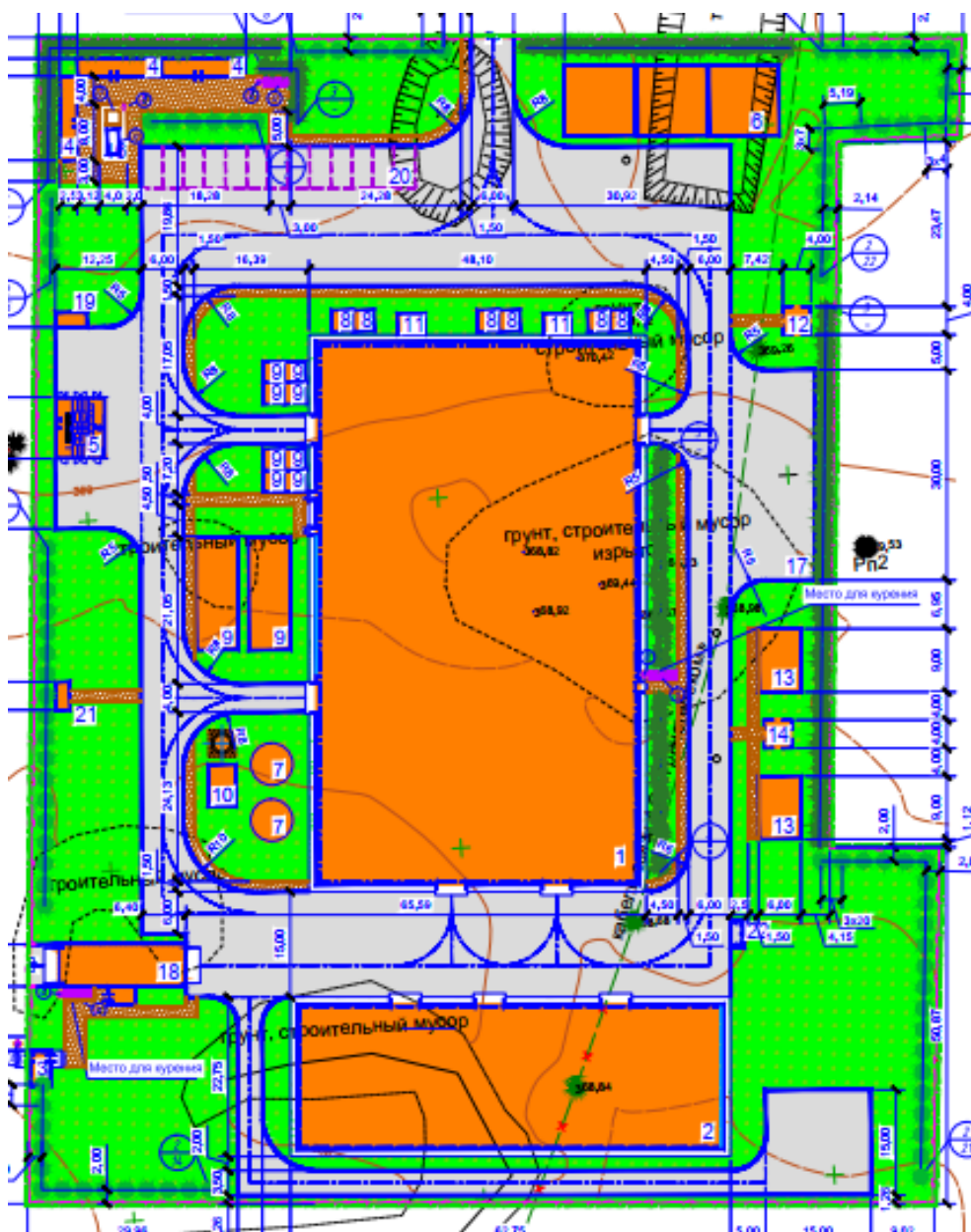
Рисунок 8.1.2.- Схема озеленения территории промплощадки
