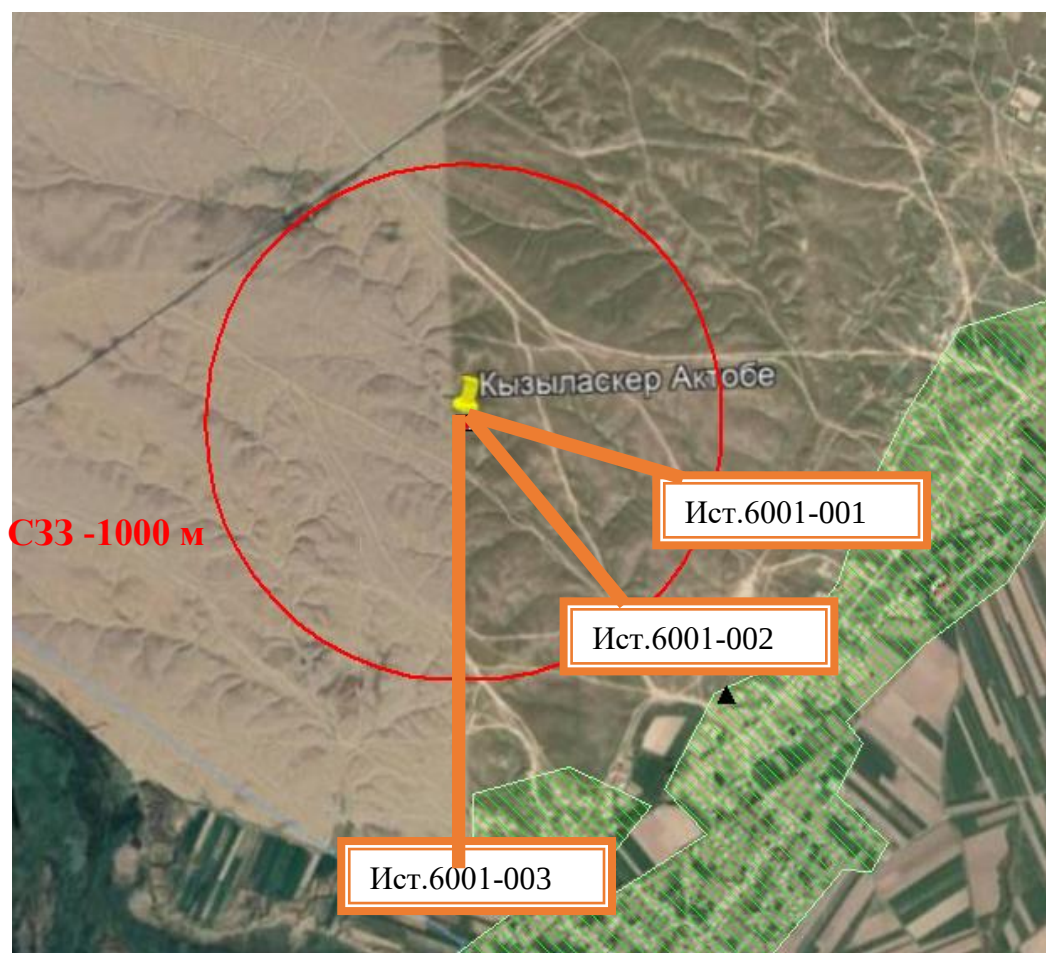
Рис.3 Полигон ТБО с.Кызыласкер
