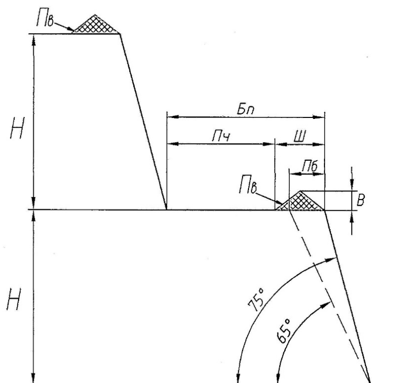
Рис.3.5.2 Схема уступа для строительного камня
