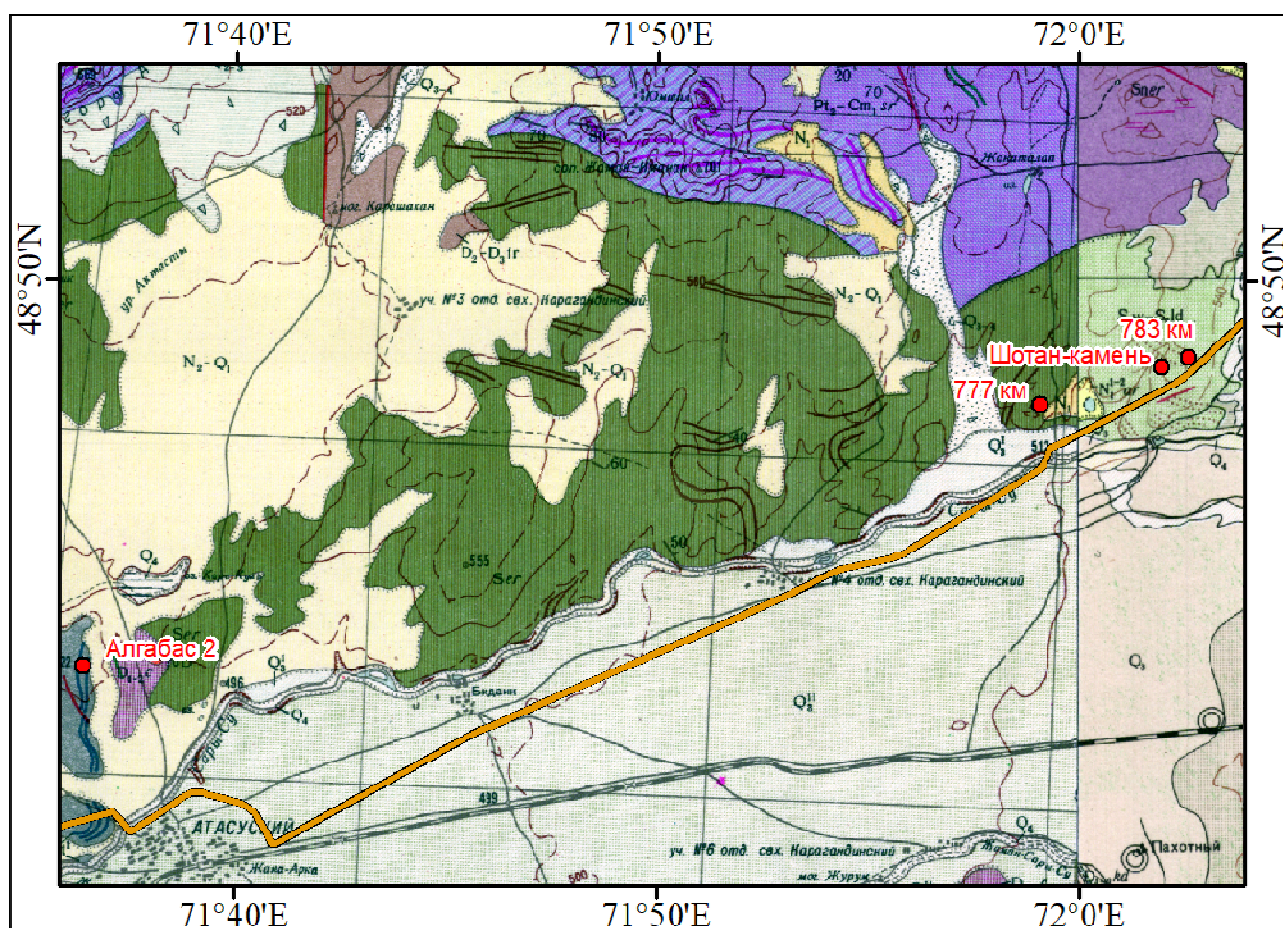
Рис.2.1 Геологическая карта расположения участка «Шотан-камень» (выкопировка из геологической карты листа М-42-XXX и М 43-XXV). Масштаб 1:200 000
