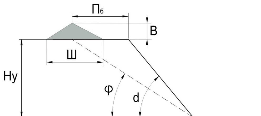
Рис.3.5.1Схема уступа при отработке грунтов
