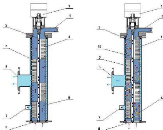
Рисунок 3-3-Процесс очистки в фильтрах ССФ
