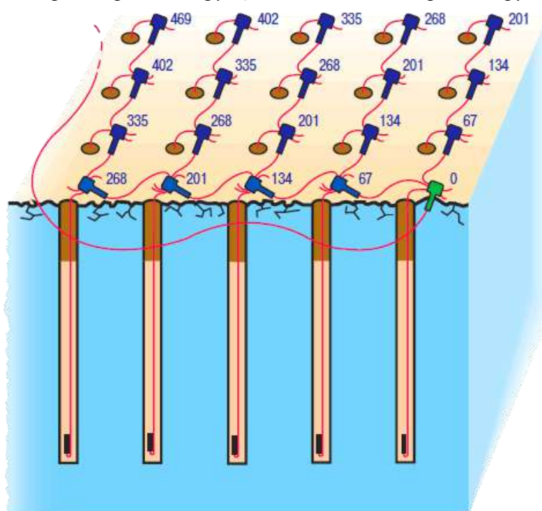
Рисунок 1.10 - Параметры конструкции скважинного заряда на рудных уступах.
