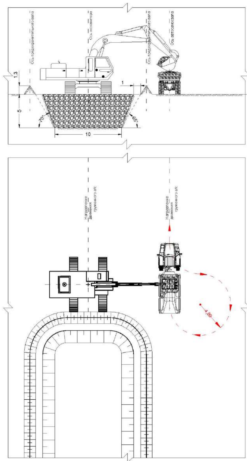
Рисунок 1.8 - Схема проходки траншеи (съезда) гидравлическим экскаватором (обратная лопата) с нижним черпанием и погрузкой в автосамосвалы на уровне стояния экскаватора, с петлевым разворотом
