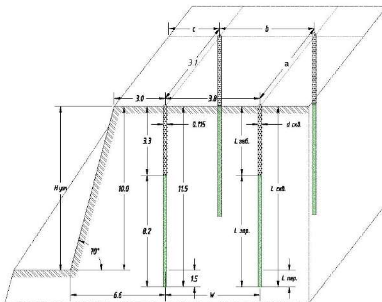
Рисунок 1.9 - Параметры конструкции скважинного заряда на вскрывше.
