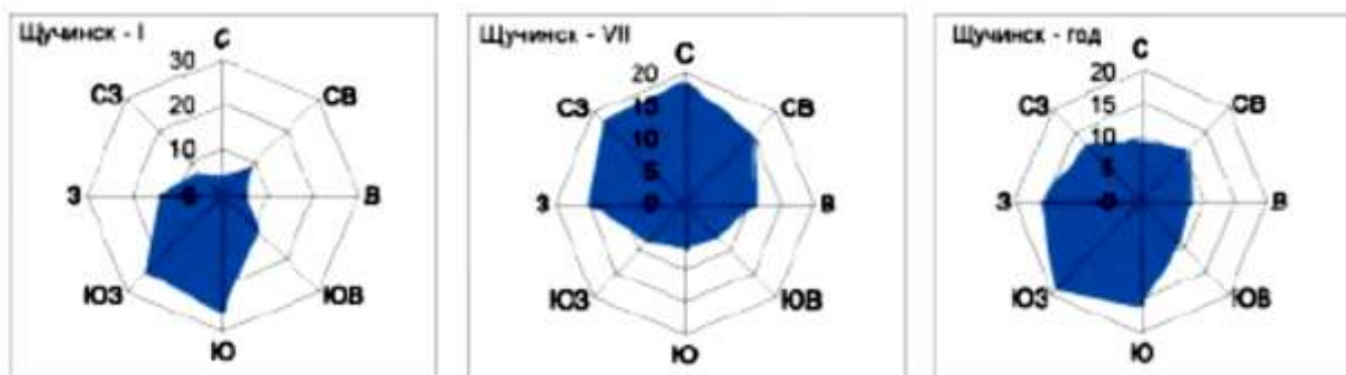
Рисунок 1.3 – Роза ветров на МС Щучинск
