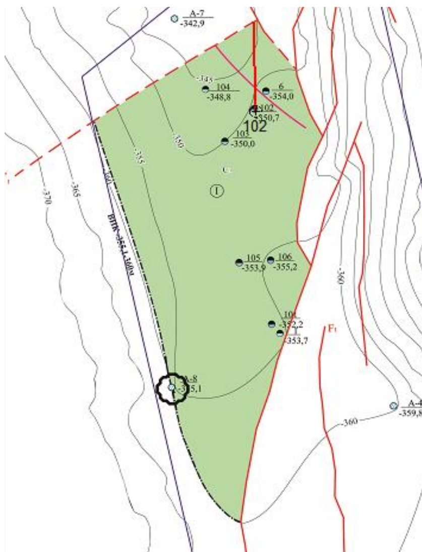
Рис 4.2 Структурная карта по кровле продуктивного горизонта М-І
