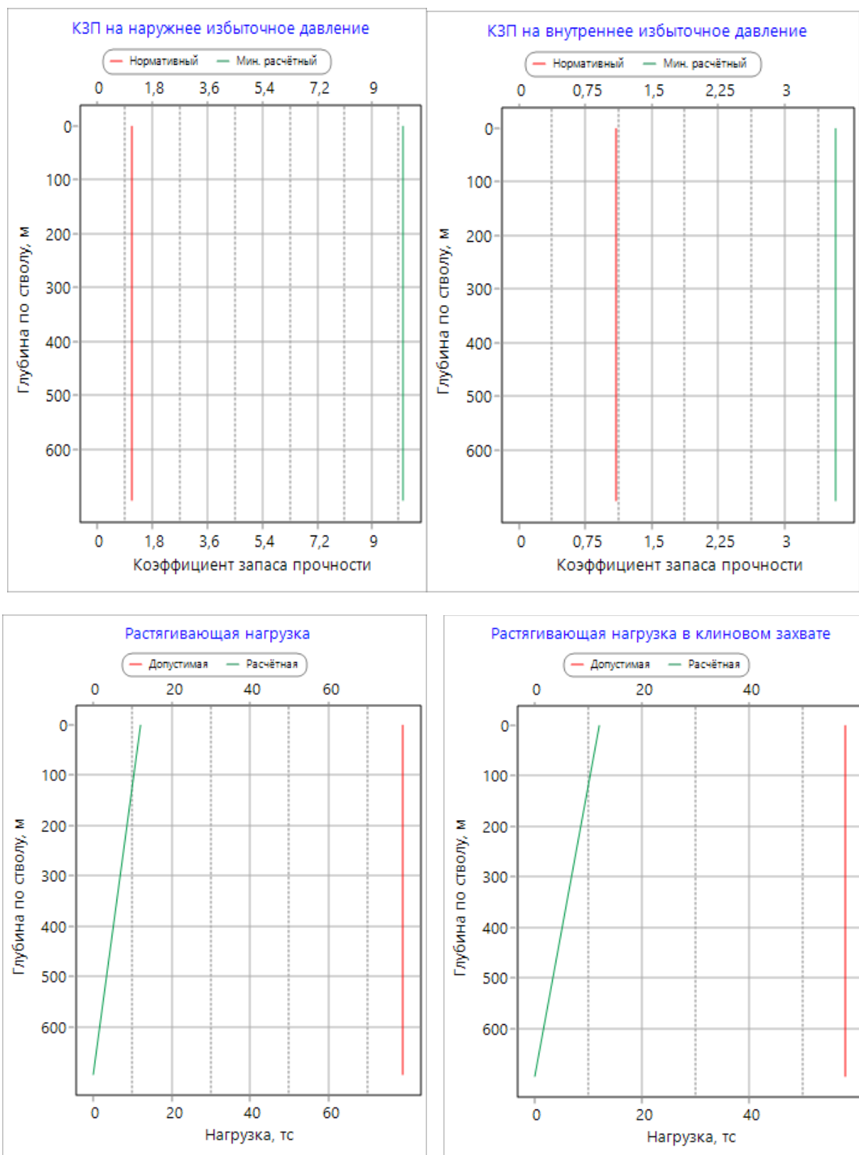
Рис. 9.1 - Эпюры избыточных давлений для колонны диаметром Ø114,3мм
