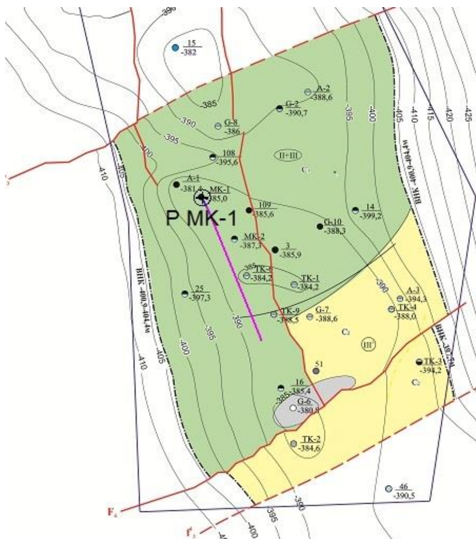
Рис 4.2 Структурная карта по кровле продуктивного горизонта М-II
