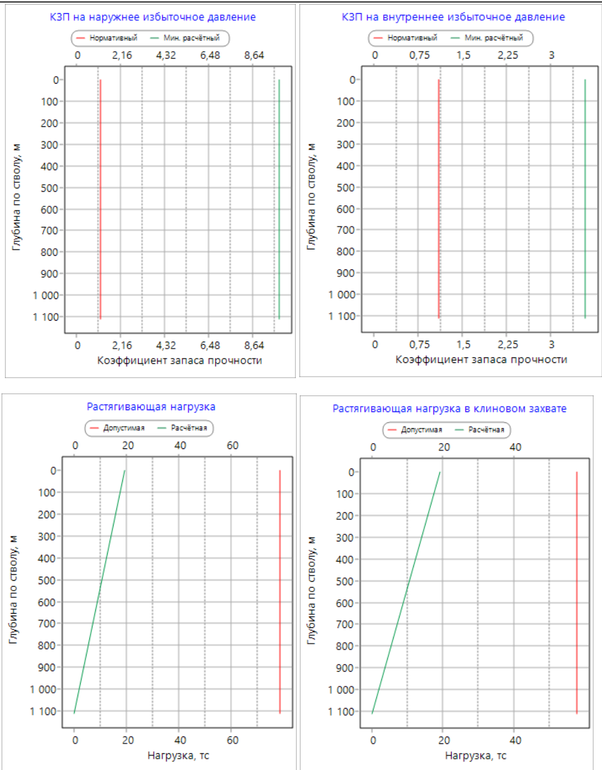
Рис. 9.1 - Эпюры избыточных давлений для колонны диаметром Ø114,3мм
