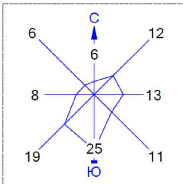
Рисунок 2.1.3 Среднегодовая роза ветров, г. Темиртау
