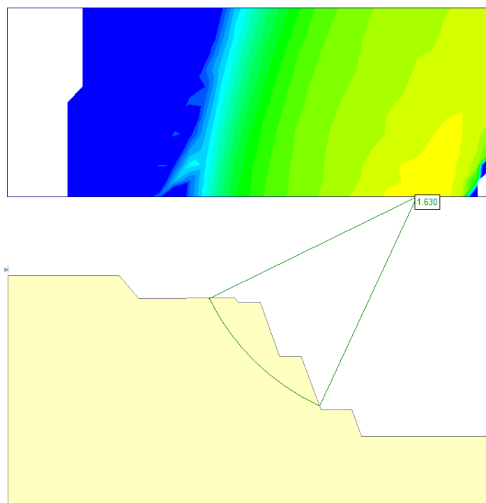
Рисунок 3.2. Результат расчета КЗУ в сечении по северному борту
