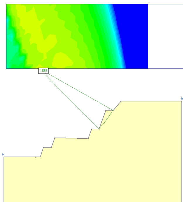
Рисунок 3.4. Результат расчета КЗУ в сечении по южному борту
