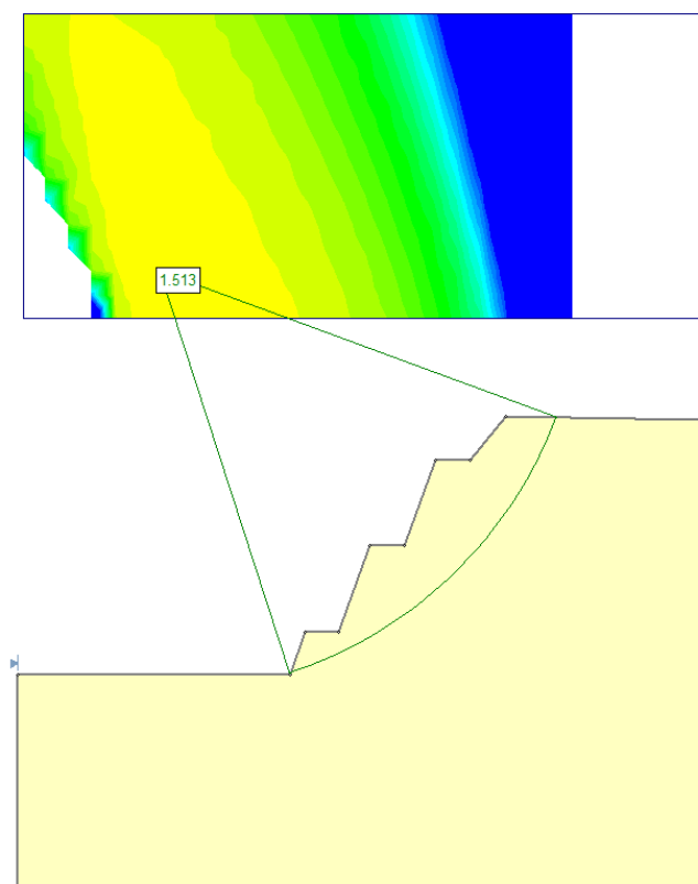
Рисунок 3.3. Результат расчета КЗУ в сечении по восточному борту
