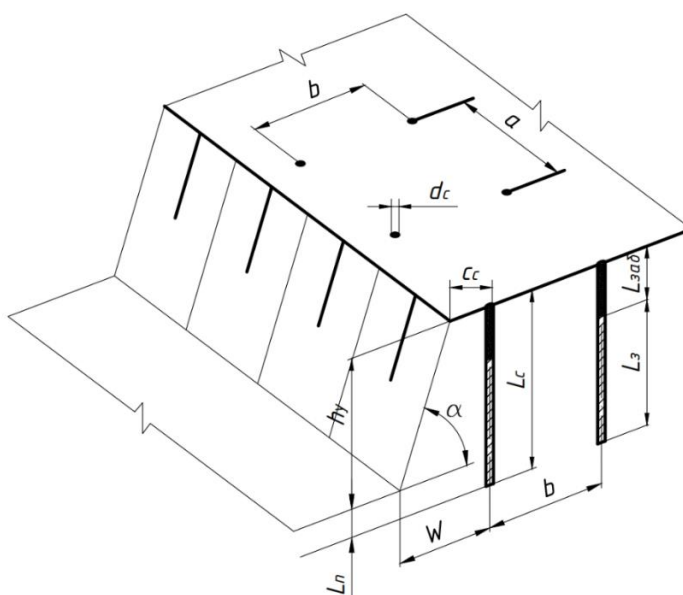
Рисунок 3.6. Схема расположения технологических скважин
