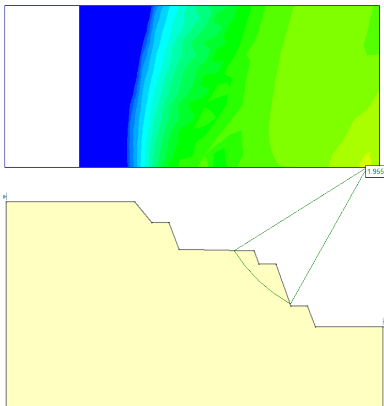
Рисунок 3.5. Результат расчета КЗУ в сечении по западному борту
