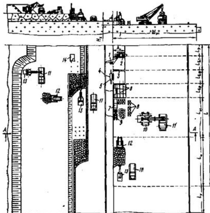
Рис. 2. Слойная панельно-пологая технологическая схема добычи облицовочного габбро при термоклинном способе подготовки их к выемке и разработке массивов:
