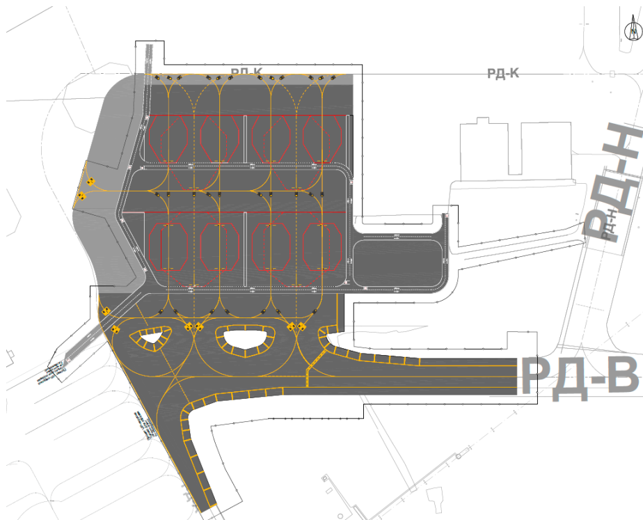
Схема расширения площадки по обработке Воздушных судов противообледенительной жидкостью
