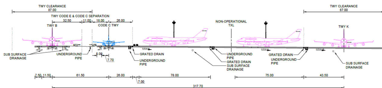
Поперечный разрез Площадки по обработке противообледенительной жидкостью при обслуживании ВС с кодовой буквой Е.
