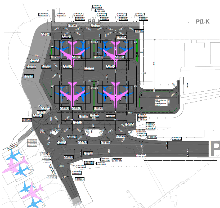
Схема расстановки ВС на площадке ПОЖ.
