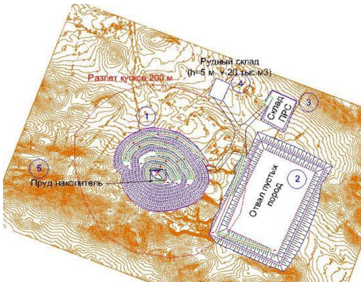
Рис. 10. Генплан месторождения Тасты-Биен
