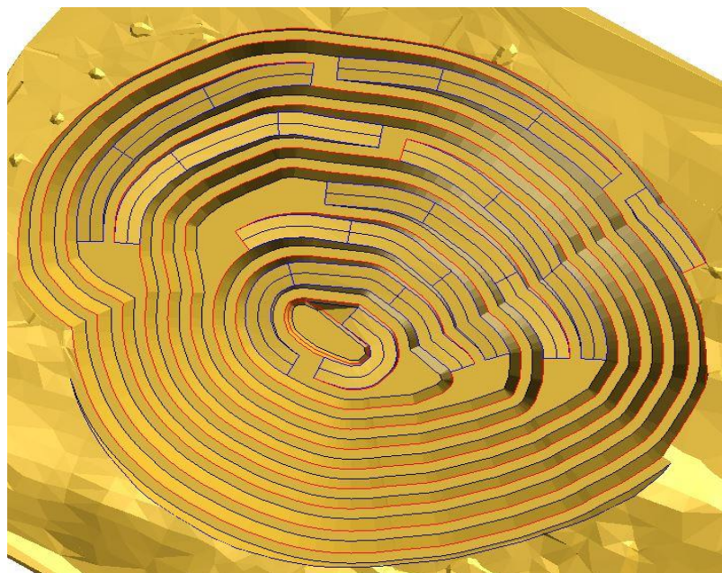
Рис. 5. План карьера месторождения Тасты-Биен
