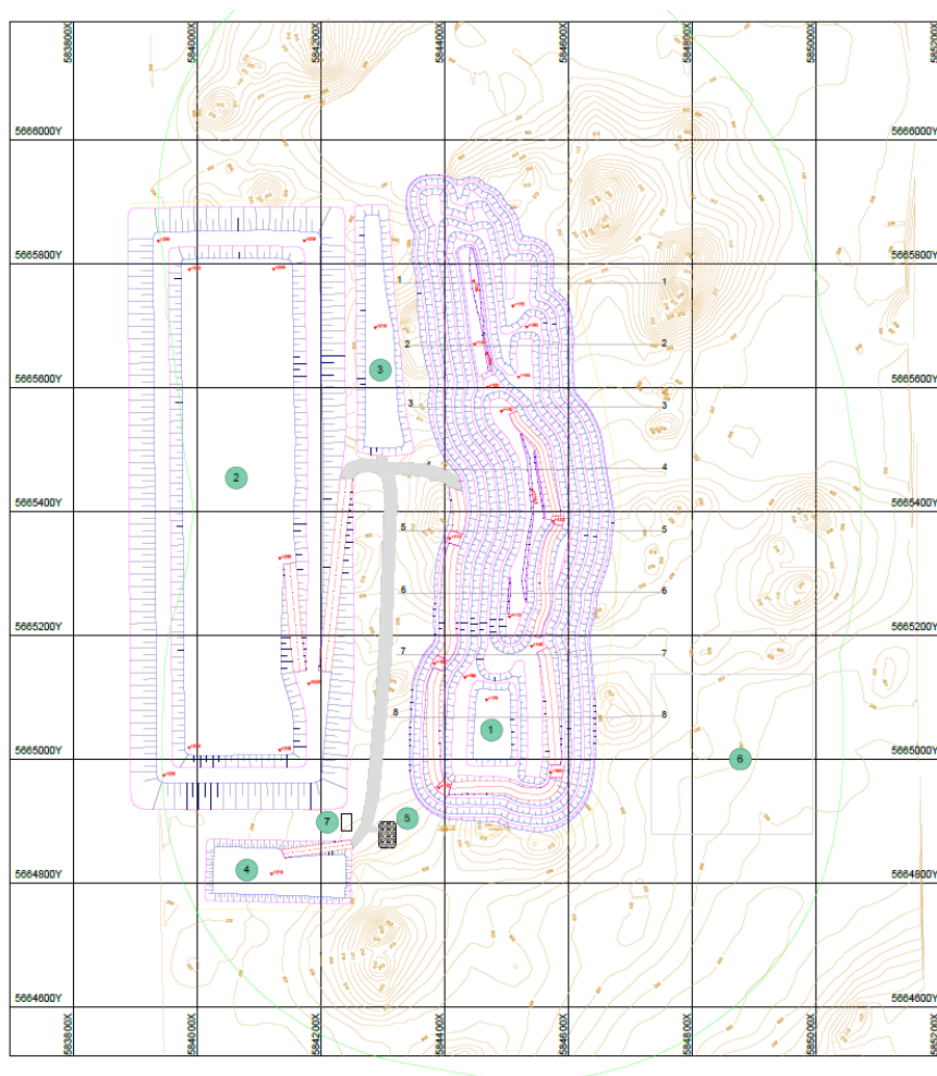
Рис. 1. - Генеральный план месторождения Жуантобе
