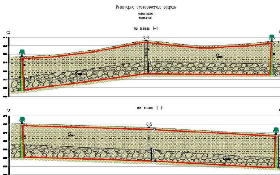
Рис. 2.16. Схема геологического строения участка «км 119»
