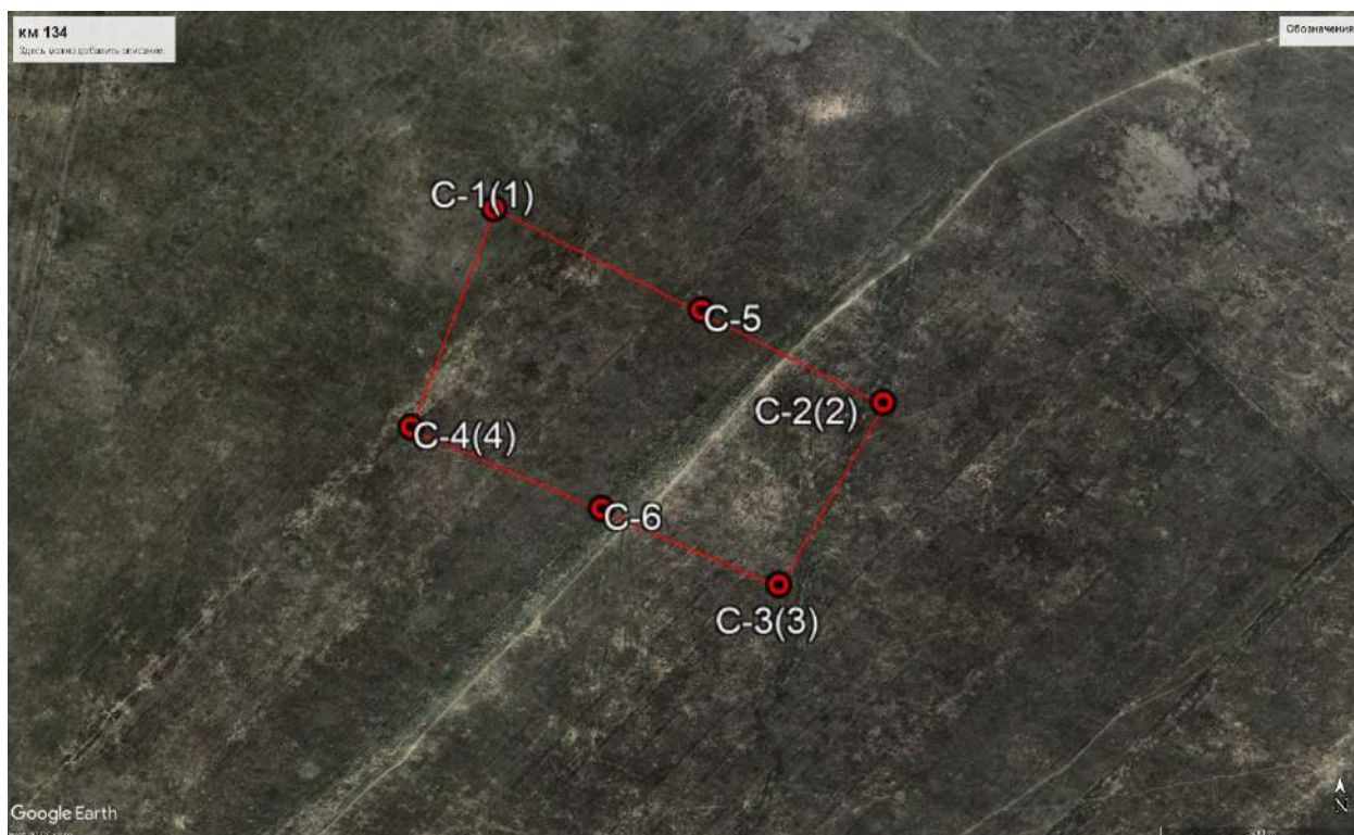
Рис 1.21 Схема участка «км 134» с расположением скважин (на основе космоснимка)
