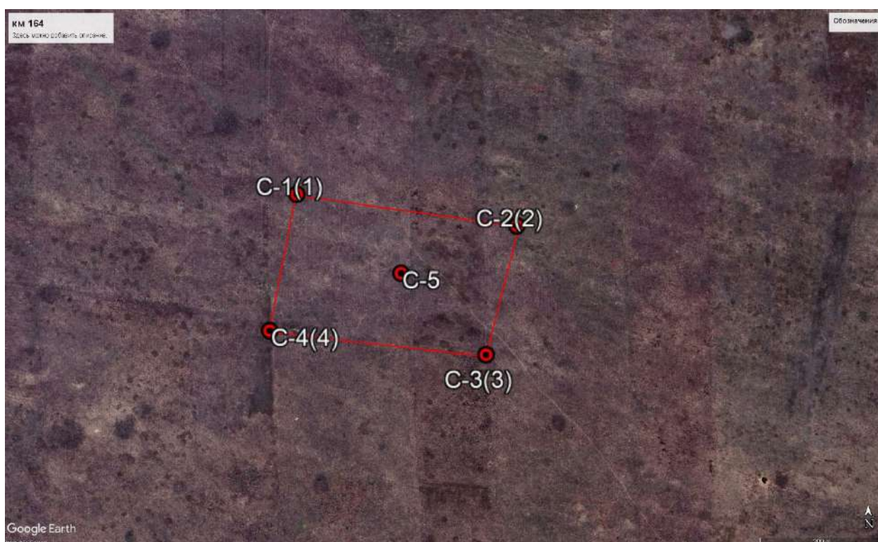
● С-1(1) -местоположение и номер скважины, в скобках - угловой точки Рис 1.25 Схема участка «км 164» с расположением скважин (на основе космоснимка)
