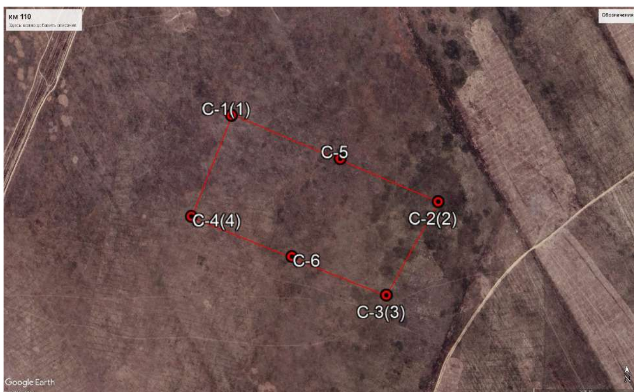
● C-1(1) -местоположение и номер скважины, в скобках - угловой точки Рис 1.17 Схема участка «км 110» с расположением скважин (на основе космоснимка)
