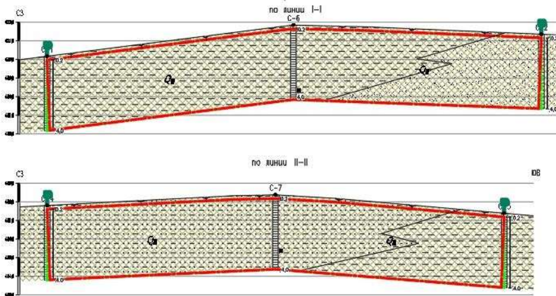
Рис. 2.20. Схема геологического строения участка «км 144»
