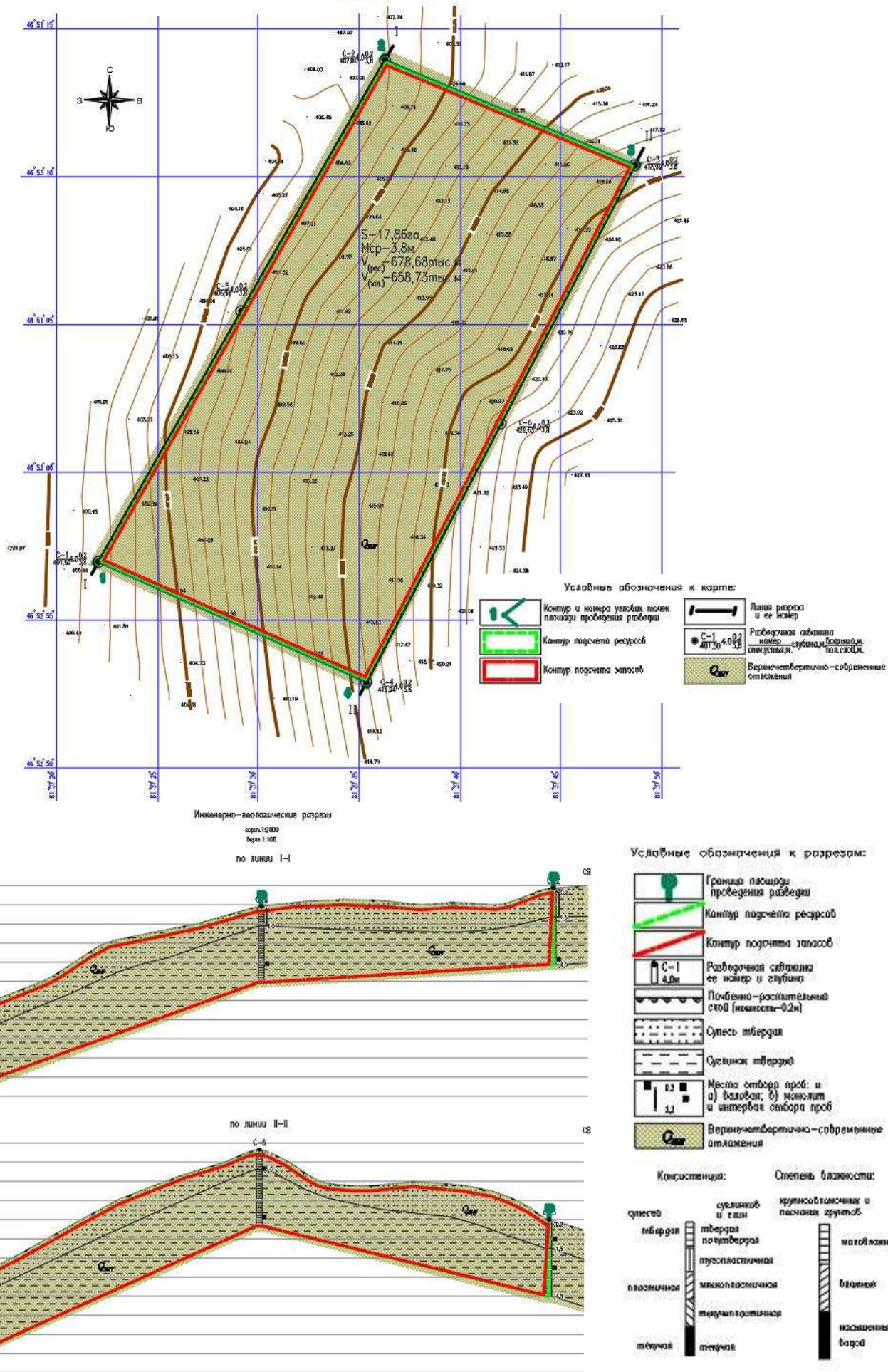
Рис. 2.26. Схема геологического строения участка «км 184»
