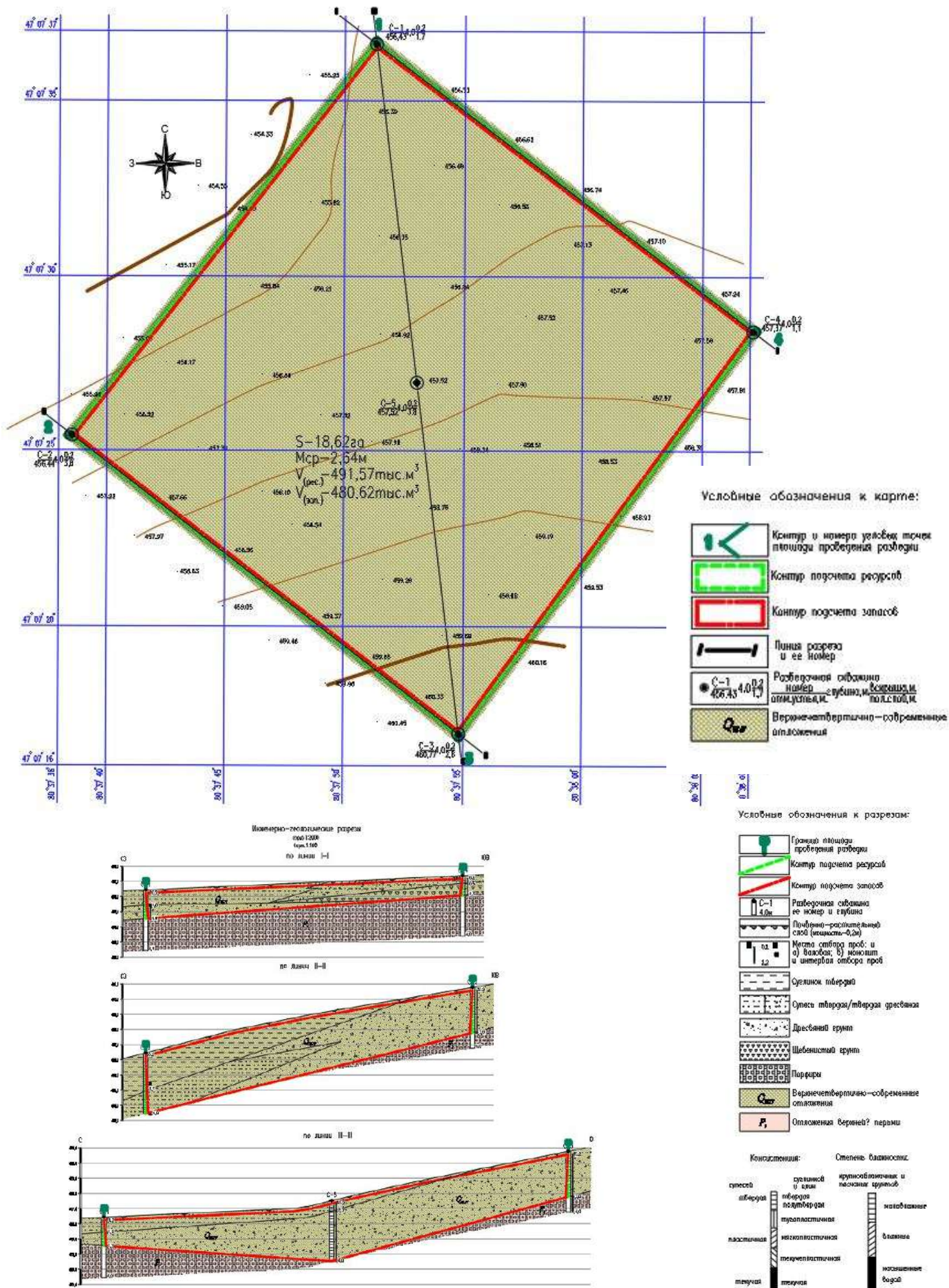
Рис. 2.13. Схема геологического строения участка «км 99»
