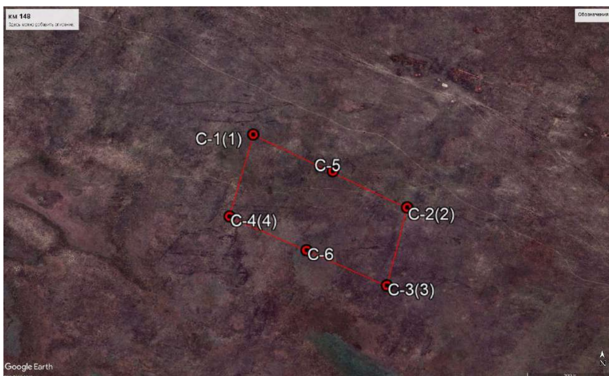
Рис 1.23 Схема участка «км 148» с расположением скважин (на основе космоснимка)
