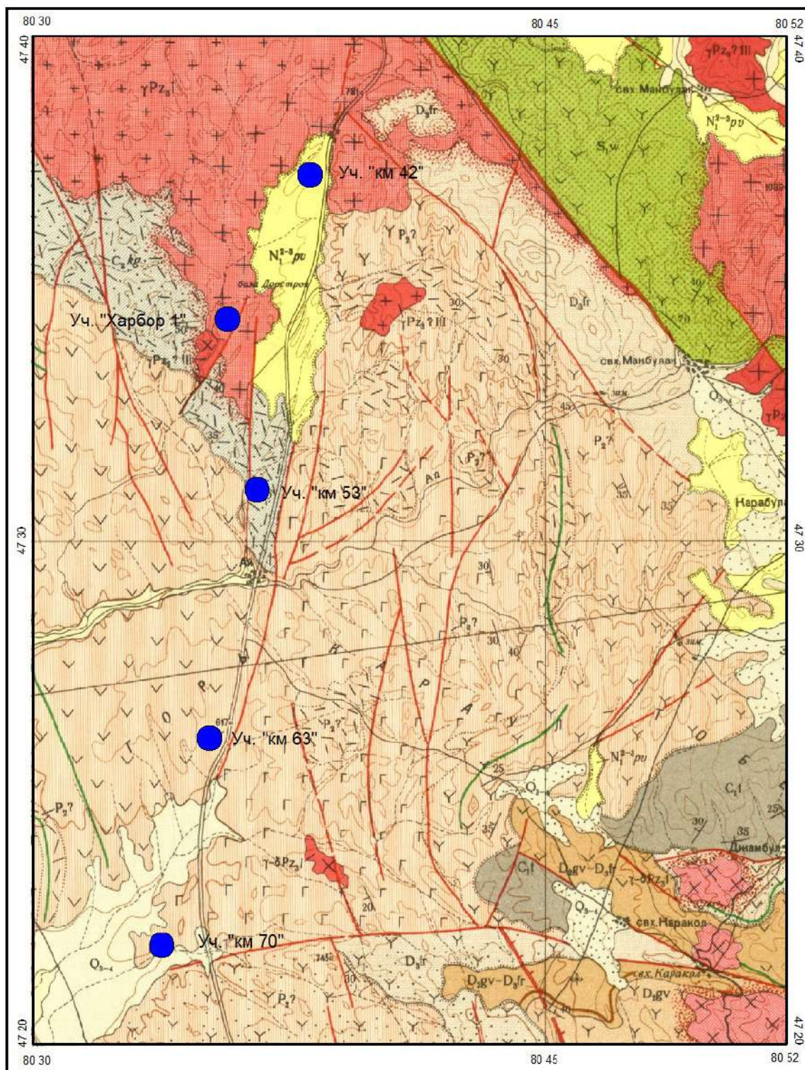
Рис.2. Геологическая карта района работ с расположением участка «км 70» (выкопировка из геологической карты листа L-44-III). Лист 1
