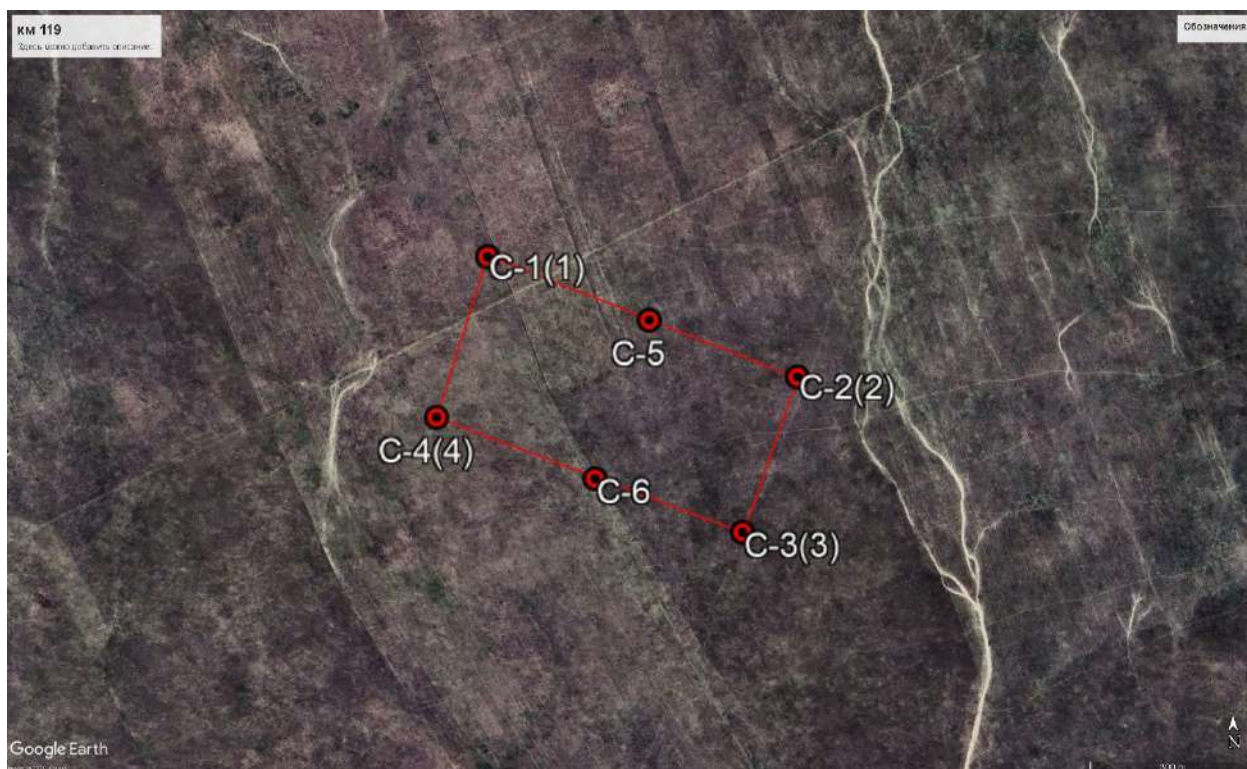
● C-1(1) -местоположение и номер скважины, в скобках - угловой точки Рис 1.18 Схема участка «119» с расположением скважин (на основе космоснимка)
