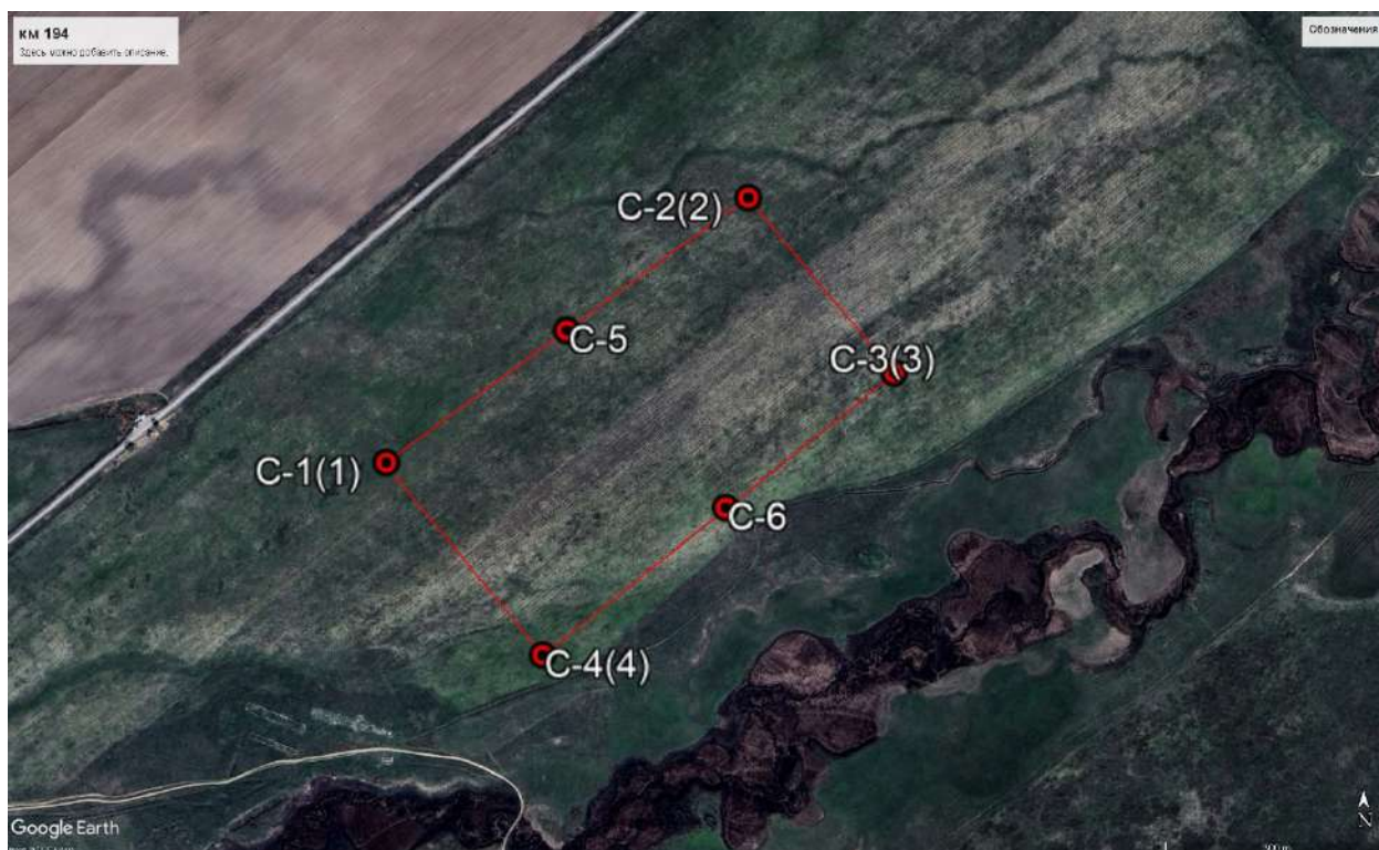
● C-1(1) -местоположение и номер скважины, в скобках - угловой точки Рис 1.29 Схема участка «км 194» с расположением скважин (на основе космоснимка)
