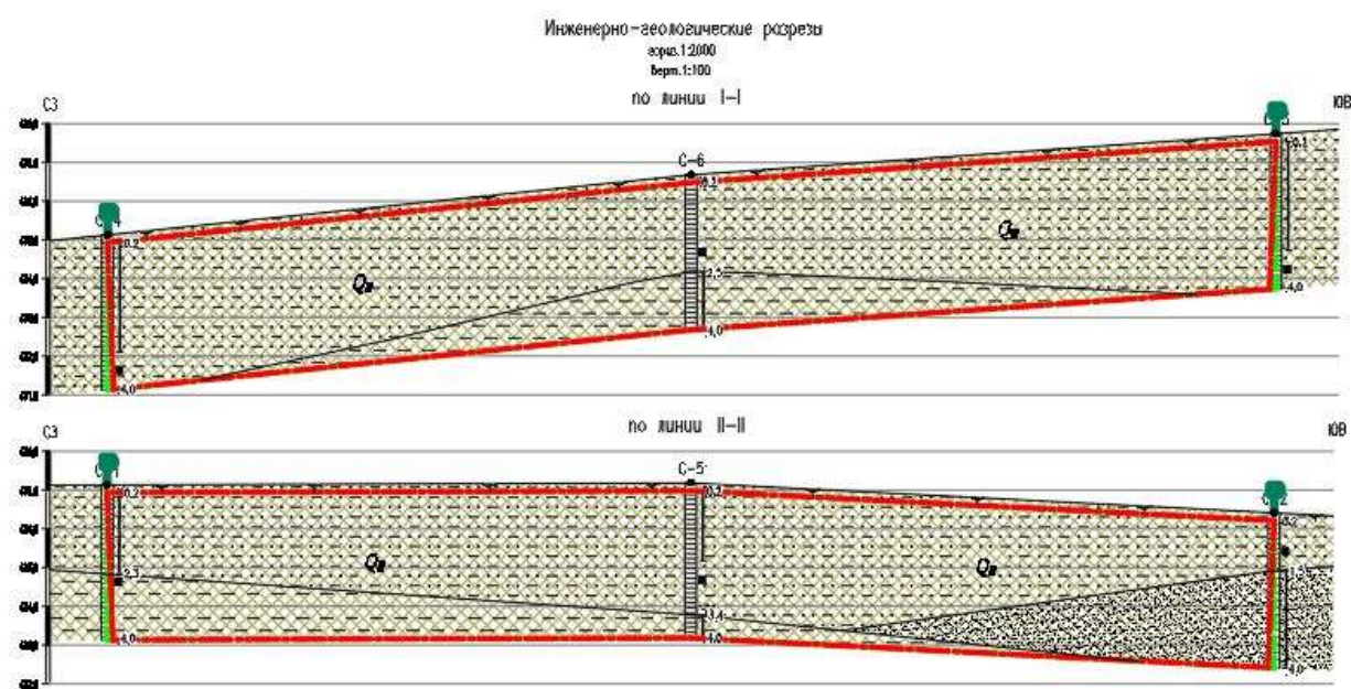
Рис. 2.22. Схема геологического строения участка «км 158»
