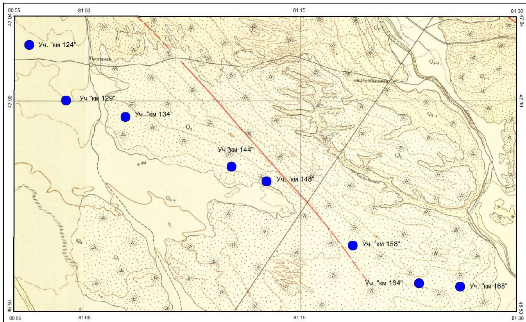
Рис.2.3 Геологическая карта района с расположением участков работ «км 124», «км 129», «км 134», «км 144», «км 148», «км 158», «км 164», «км 168» (выкопировка из геологических картлистов L-44-IX, X). Лист 3
