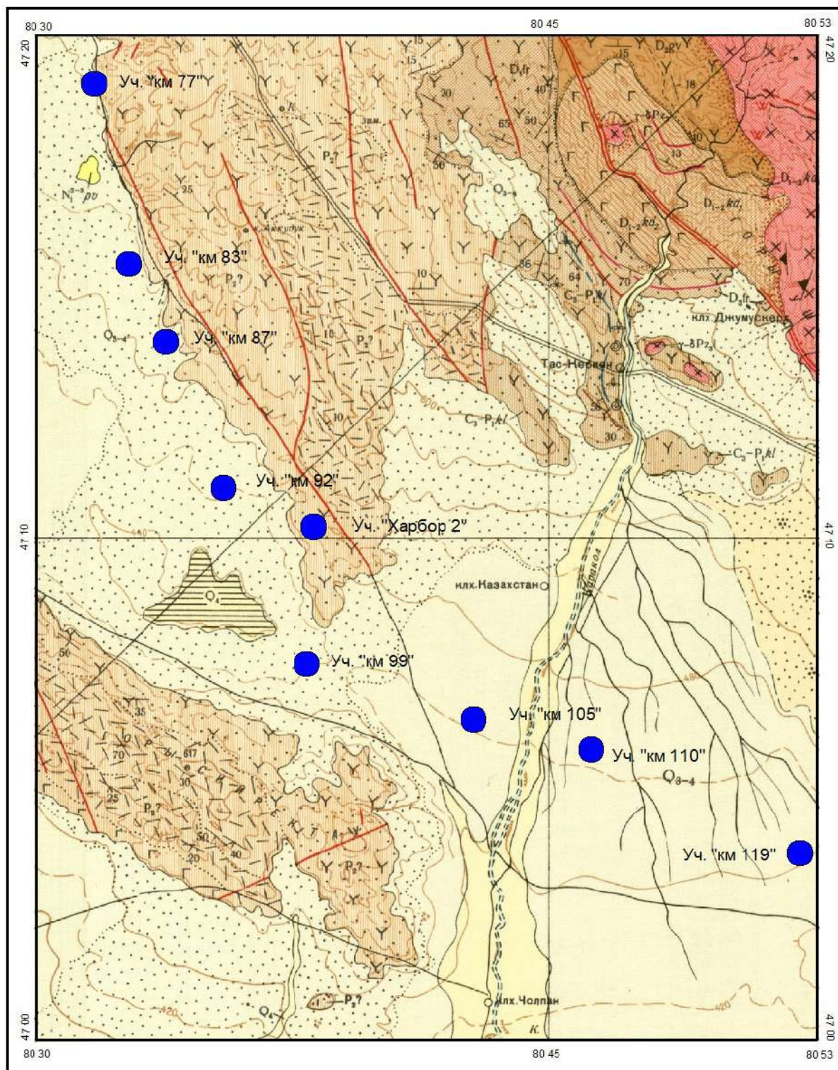
Рис.2.2 Геологическая карта района работ с расположением участков «км 77», «км 83», «км 87», «км 92», «км 99», «км 105», «км 110», «км 119» (выкопировка из геологической карты листа L-44-IX). Лист 2
