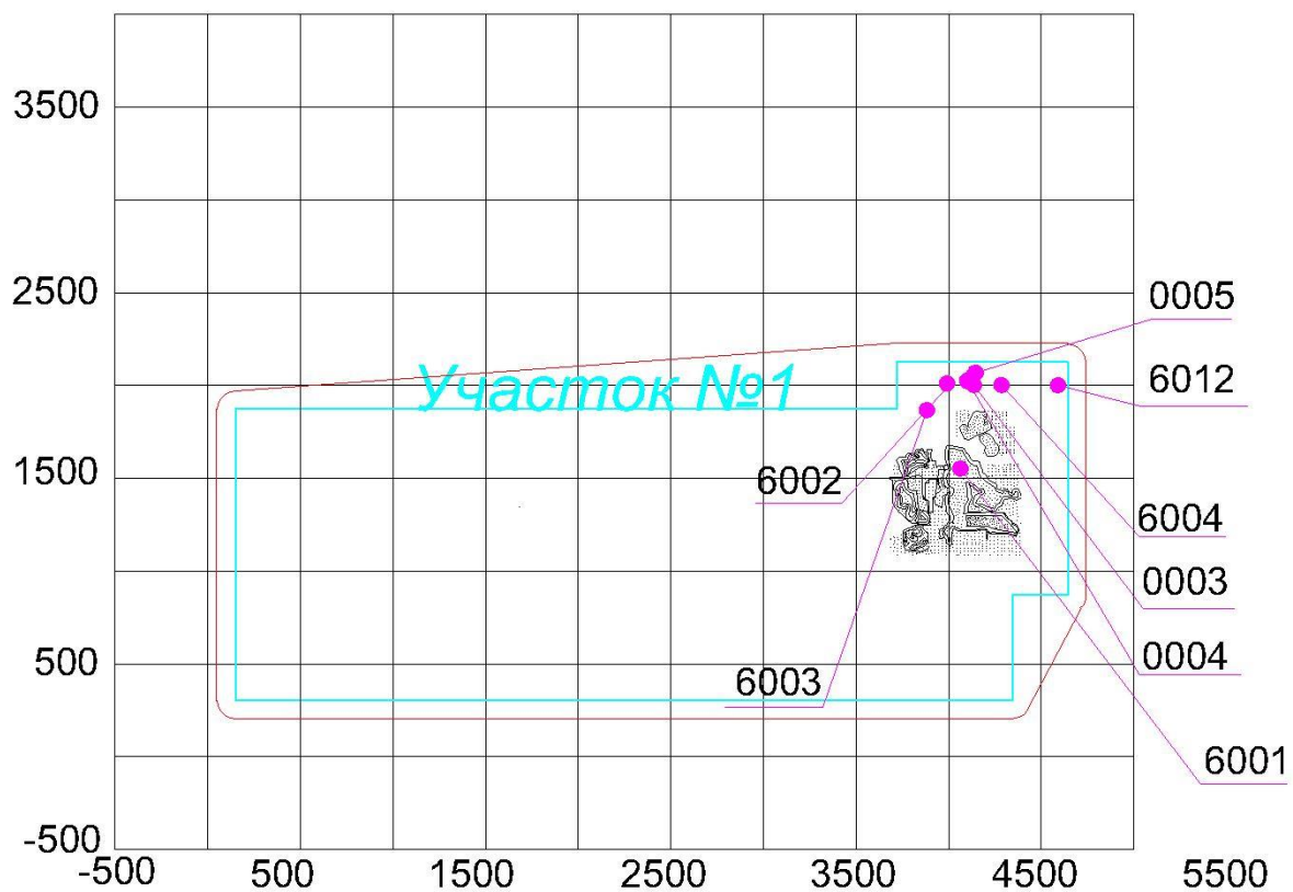
Карта-схема участка №1, с нанесенными на нее источниками выбросов в атмосферу
