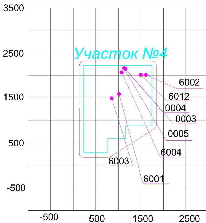
Карта-схема участка №4, с нанесенными на нее источниками выбросов в атмосферу
