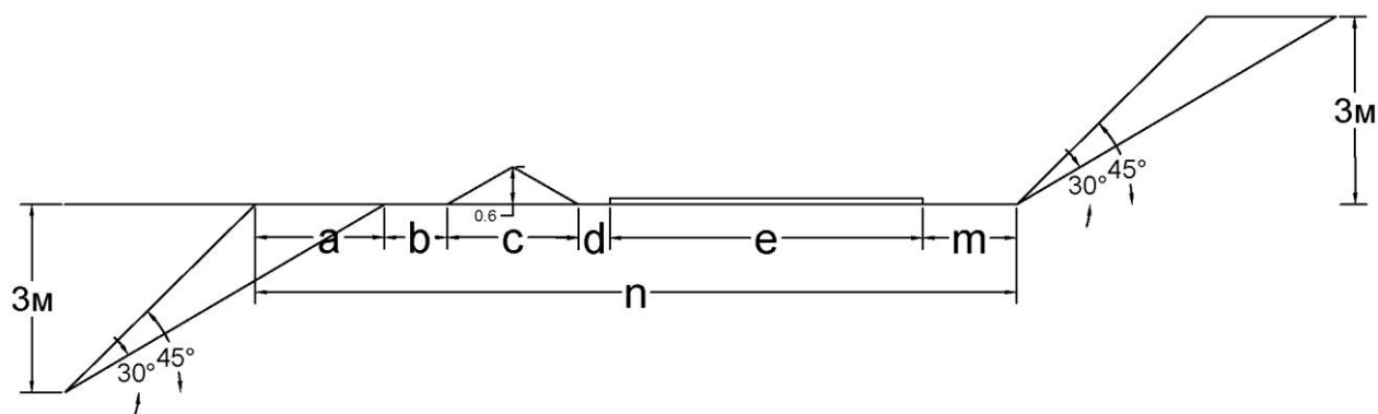
Рис. 1.2 - Расчет ширины транспортного съезда
