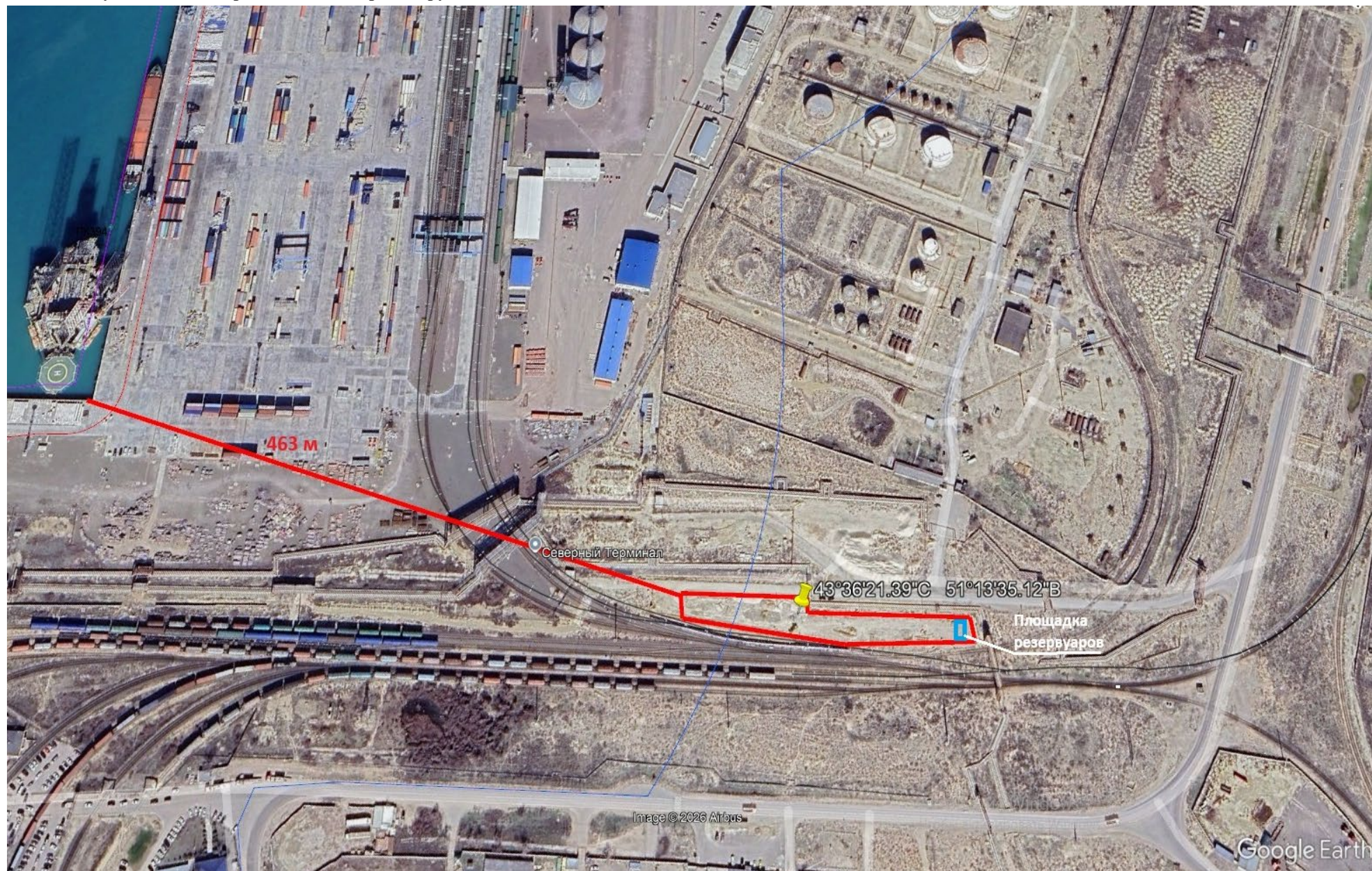
Рисунок 1 – Схема расположения проектируемого объекта.
