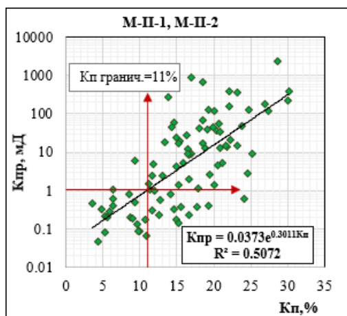
Рисунок 2.2.5 – Зависимость коэффициента проницаемости от коэффициента пористости (М-П-1, М-П-2)
