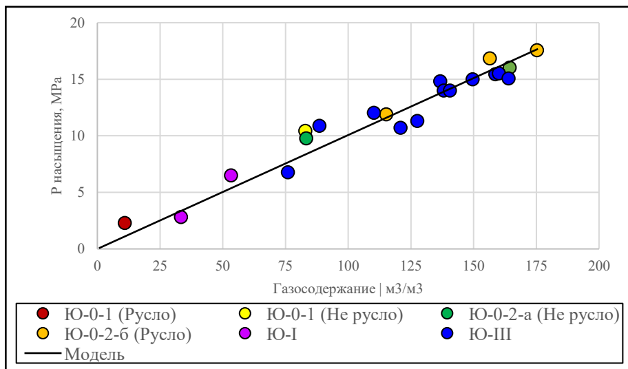
Рисунок 2.3.1 – Зависимость давления насыщения от газосодержания
