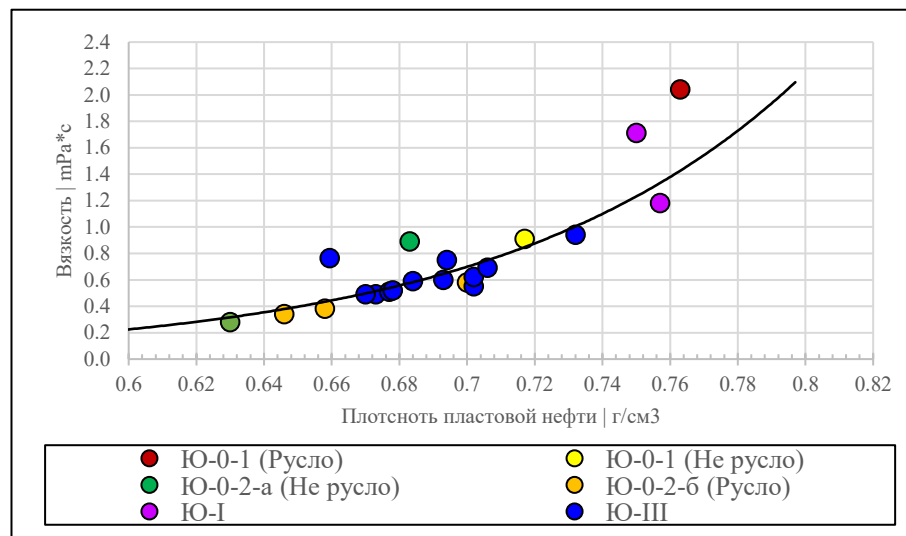
Рисунок 2.3.4 – Зависимость вязкости от плотности пластовой нефти
