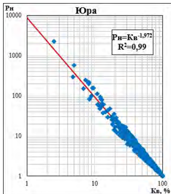
Рисунок 2.2.12 – Зависимость параметра насыщения от коэффициента водонасыщенности для юрских отложений
