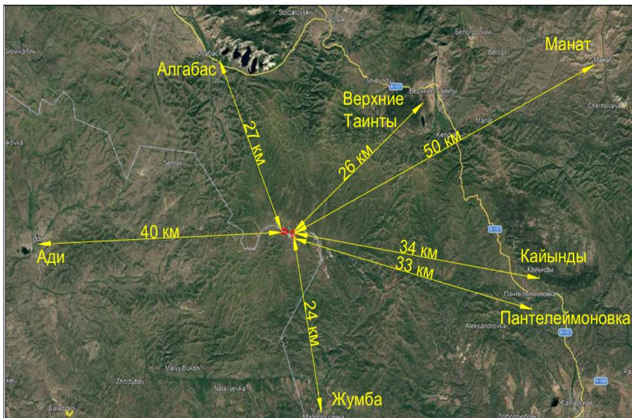
Ситуационная карта-схема района расположения месторождения "Большая Буконь". Масштаб 1:50000
