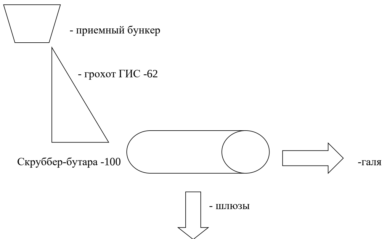
Рис 3.1.– Схема промывочной установки
