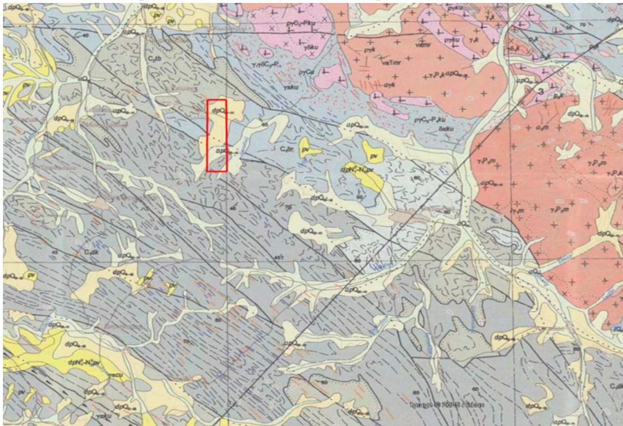
Рис. 3.2 Геологическая карта участка «Мажера 1» Масштаб: 200:000
