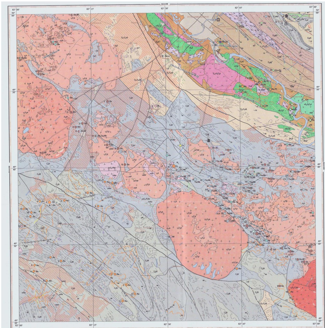
Рисунок 3.5. Карта полезных ископаемых уч. «Мажера 1»
