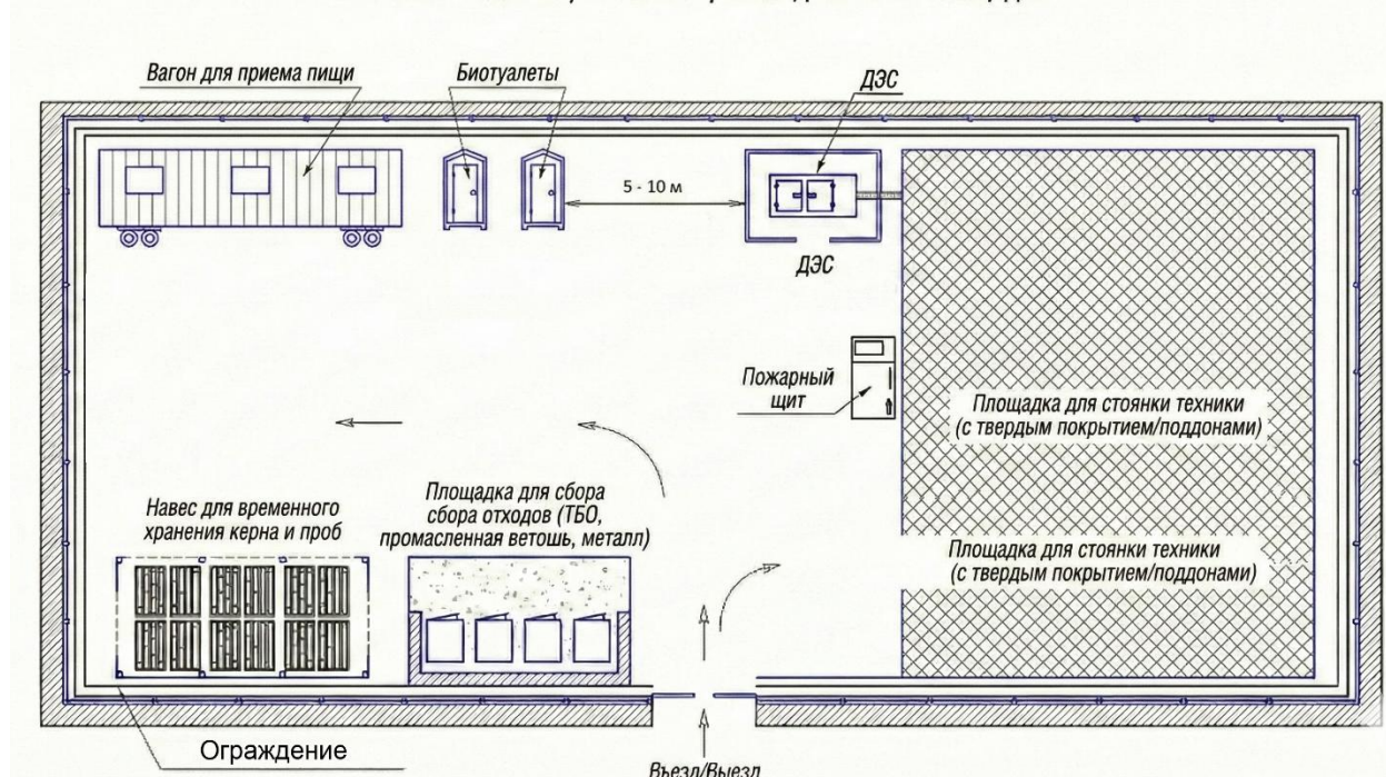
Схема мобильной временной производственной площадки
