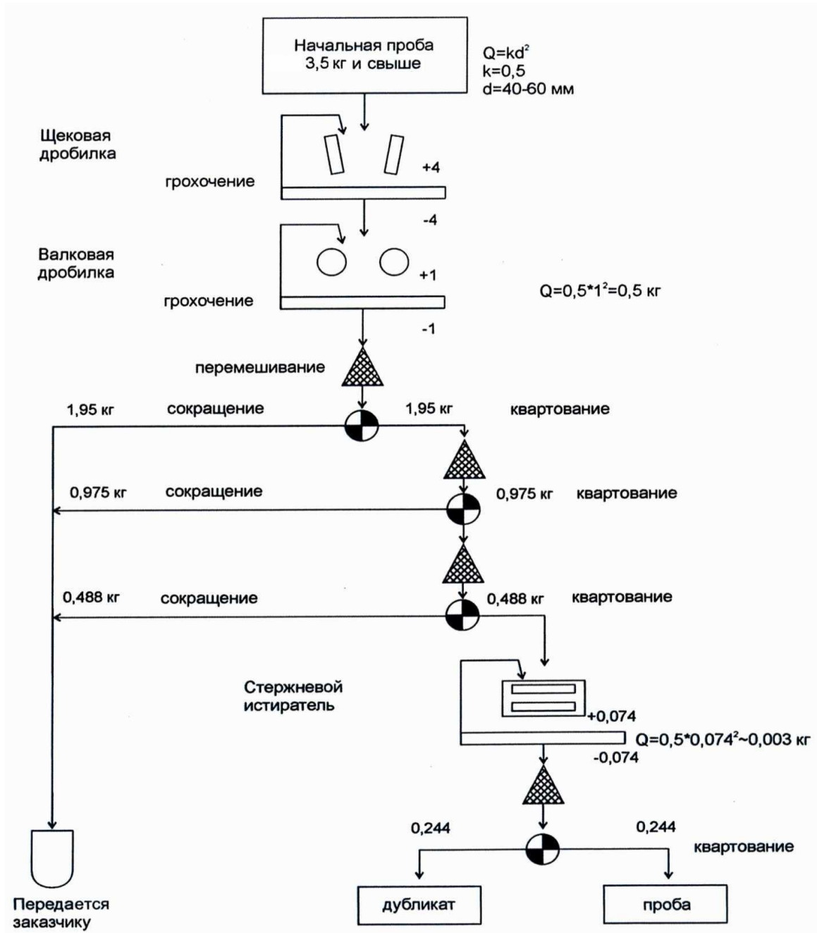
Рисунок 4.1. Схема обработки керновых проб
