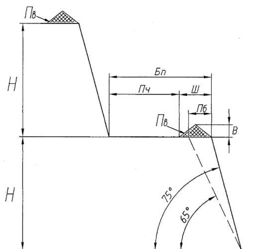
Рис.3.5.2 Схема уступа для строительного камня
