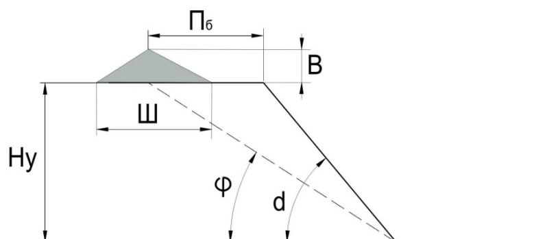
Рис.3.5.1 Схема уступа для слоя грунта
