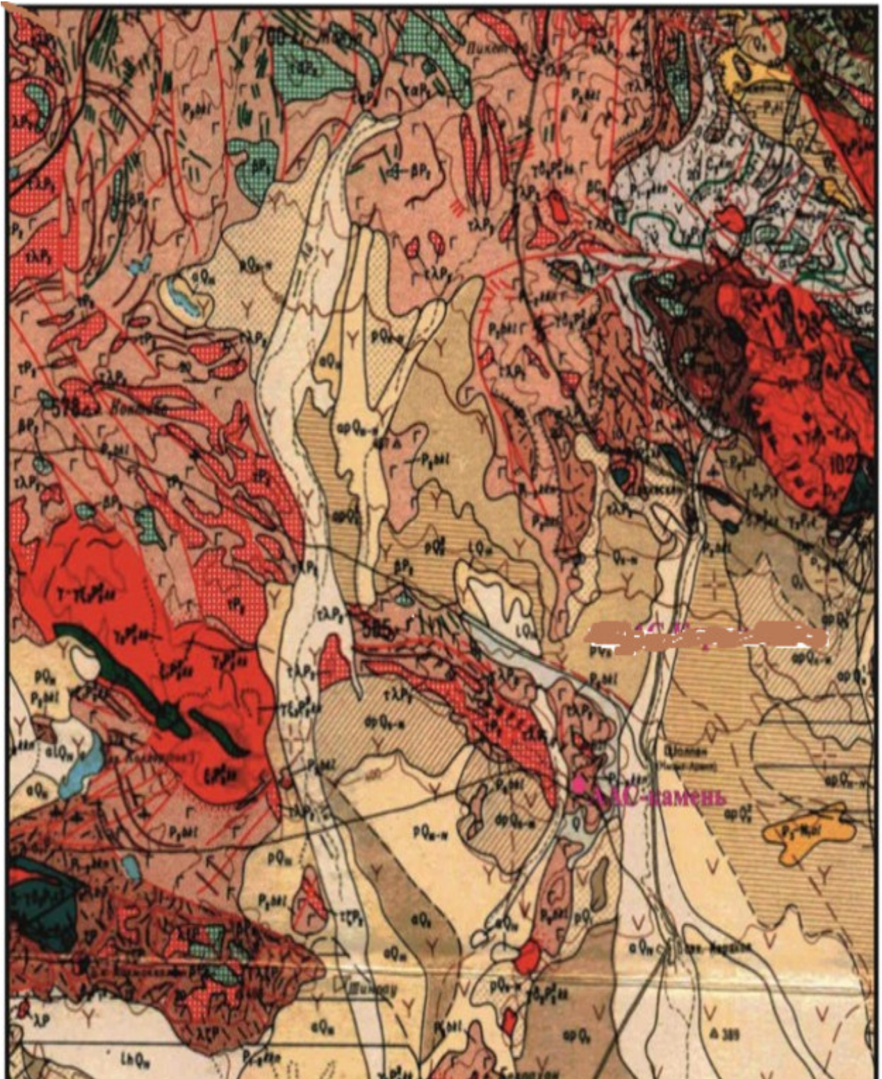
Рис.2.1 Геологическая карта района работ (выкопировка с геологической карты листа L-44-A исполнители А.К.Мясников, Л.К.Диденко-Кислицина и др.), Масштаб 1:500 000
