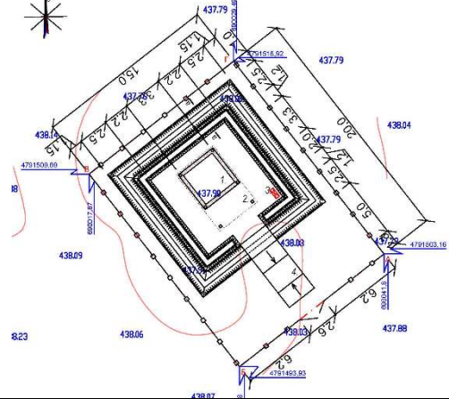
Разбивочный план
