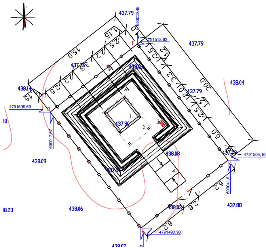
Разбивочный план
