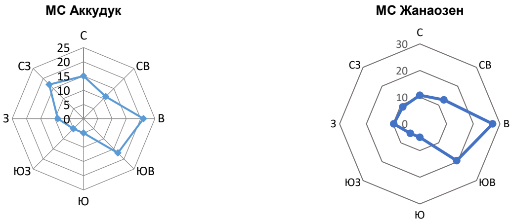
Рисунок 3.1.1 Розы ветров
