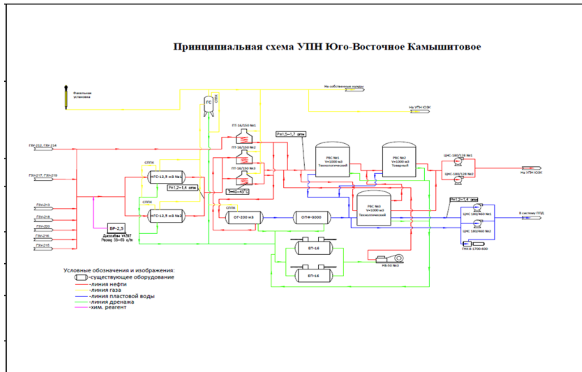
Рисунок 1.5.1 - Принципиальная схема УПН месторождения Юго-Восточное Камышитовое
