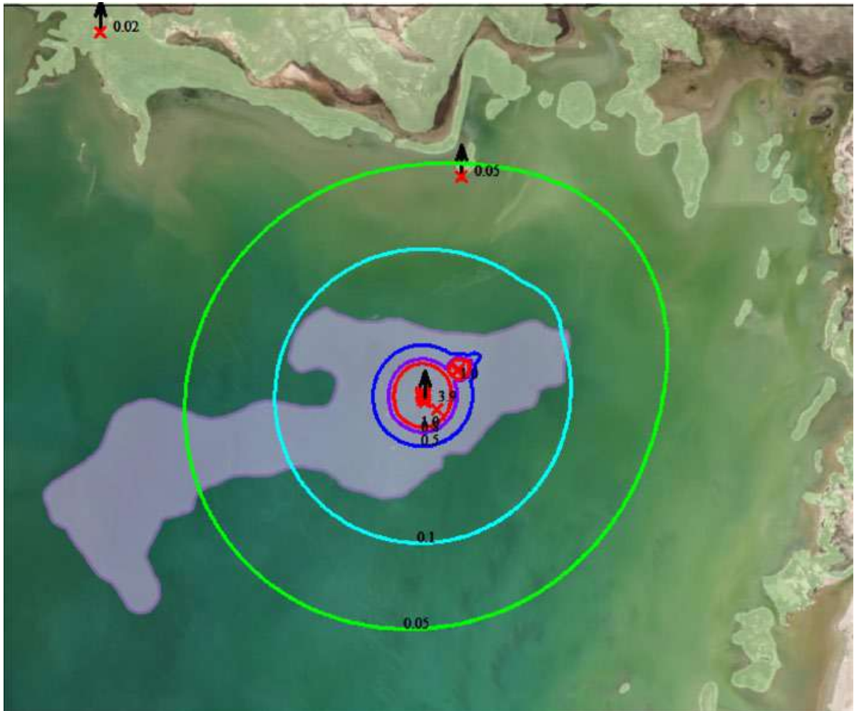
Рисунок 4.3.1 Результаты расчета рассеивания по группе суммации ( \text{NO}_2+\text{SO}_2 ) при штатном режиме работы
