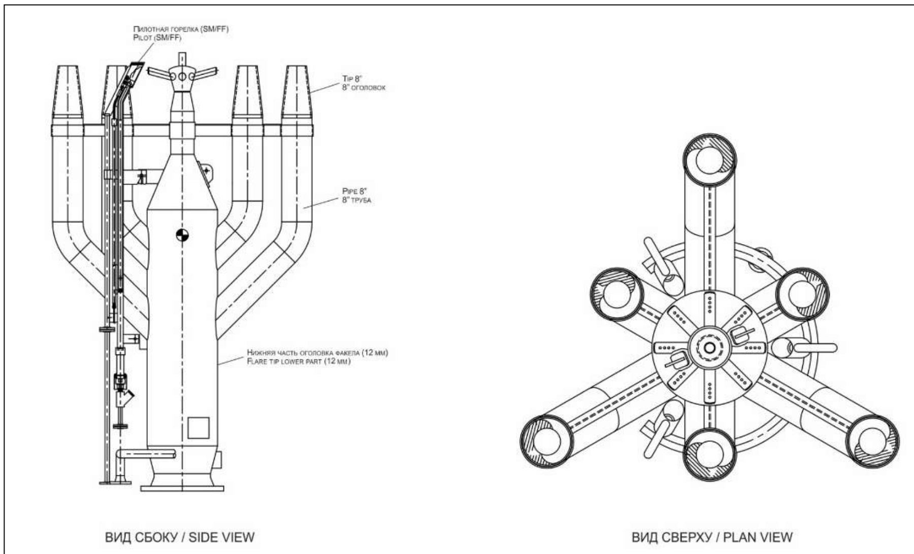
Рисунок 3.1.6 Остров А. Схема факельного оголовка ВД
