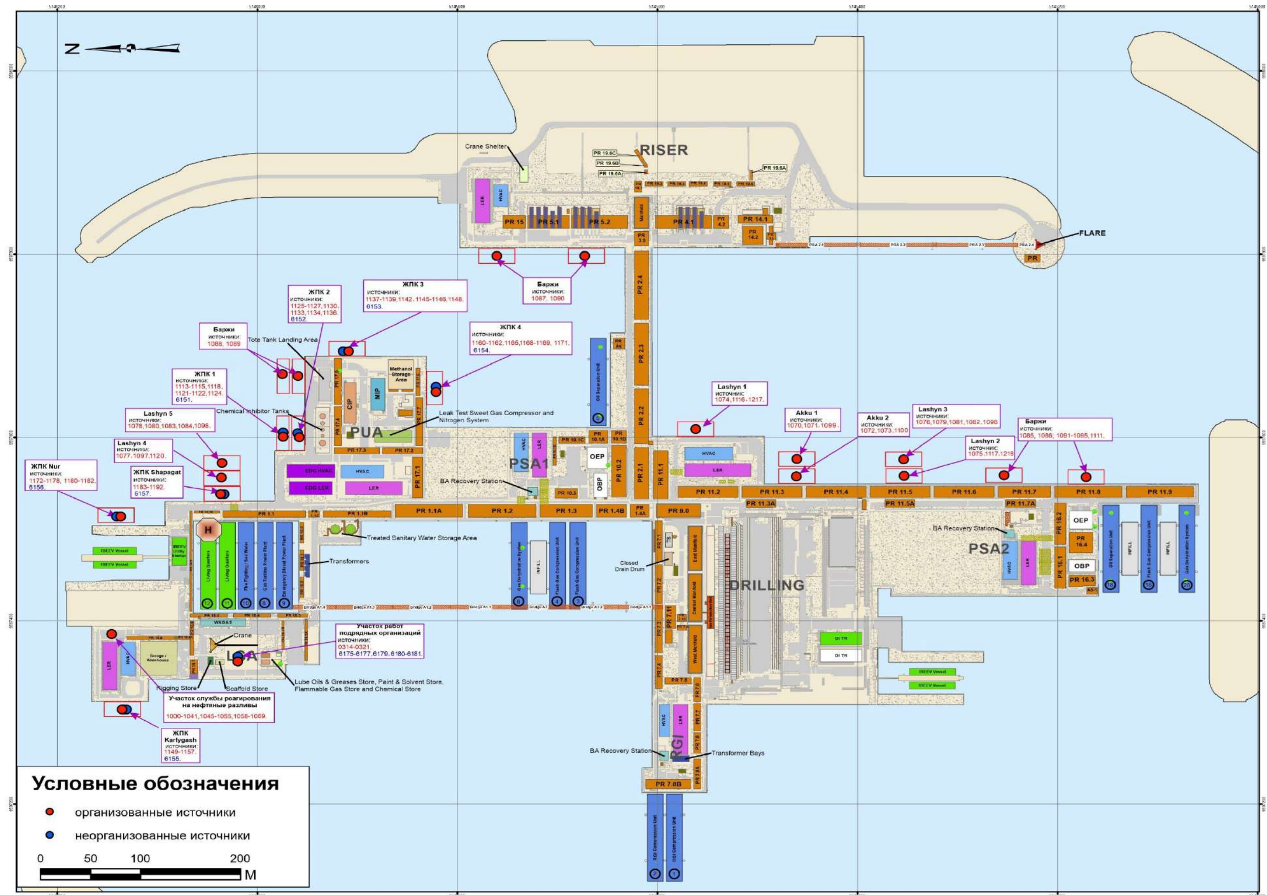
Рисунок 3.2.1 Остров Д. Схема расположения источников выбросов на участках вспомогательных работ, ЖПК и баржах
