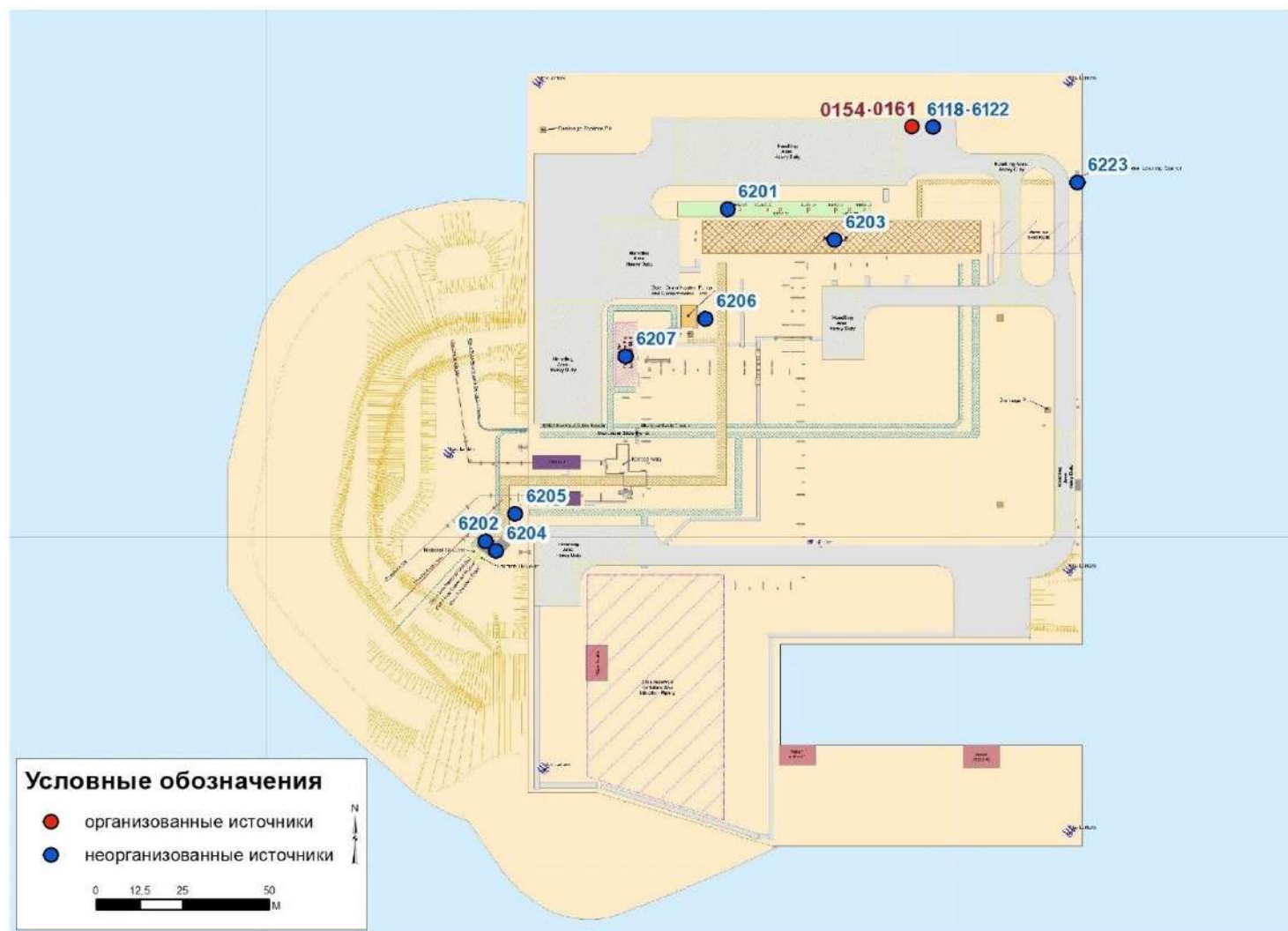
Рисунок 3.1.10 Остров EPC2. Схема расположения источников выбросов
