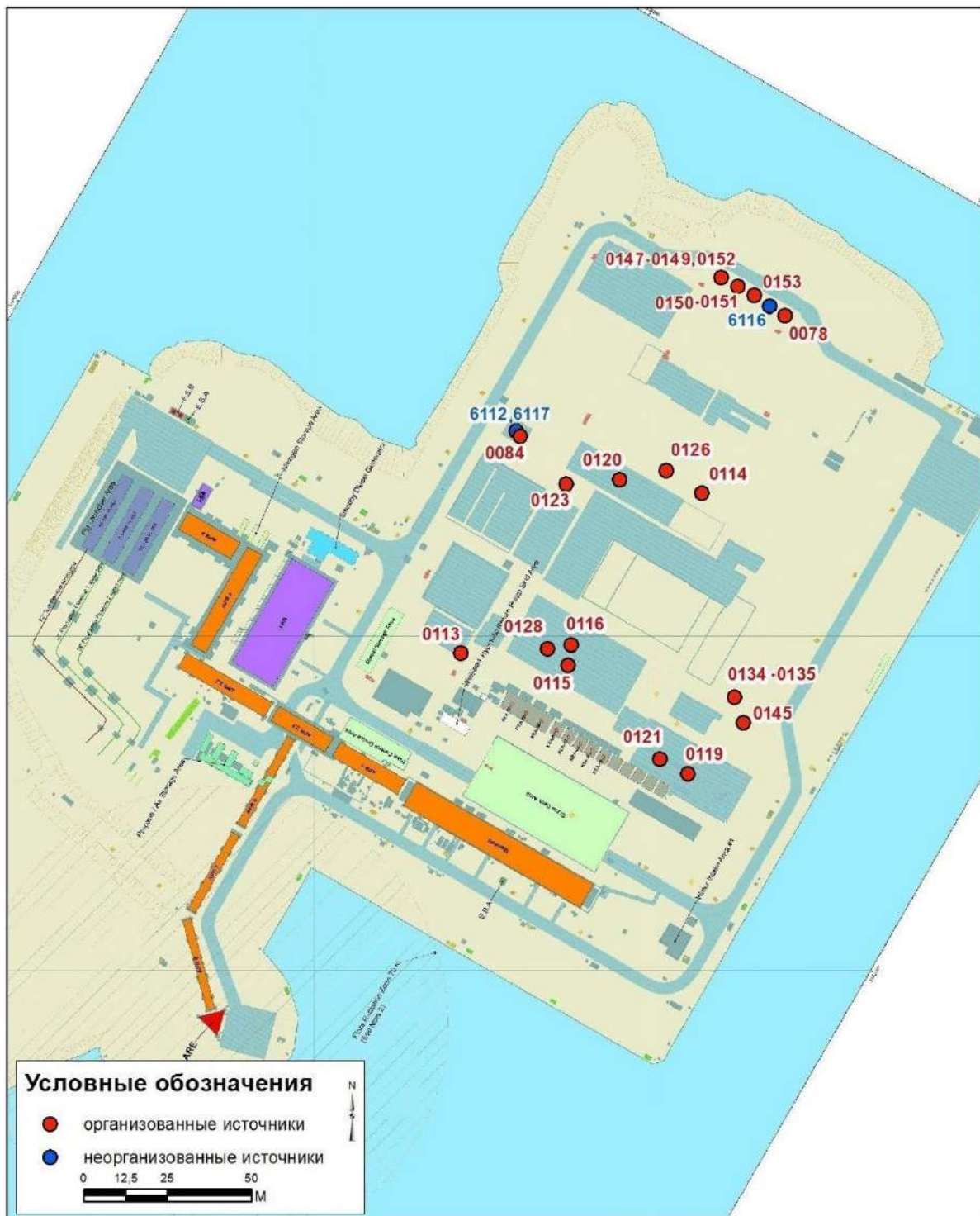
Рисунок 3.2.2 Остров А. Схема расположения источников выбросов ЗВ на участке сервисного обслуживания скважин
