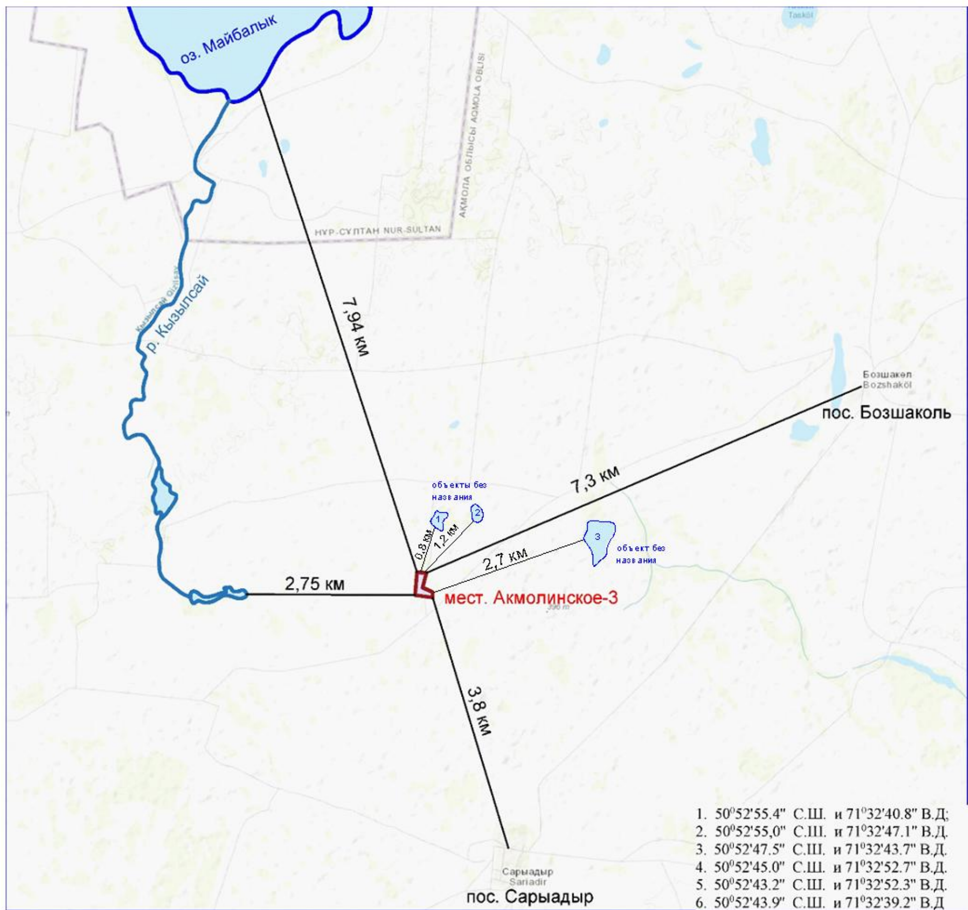
Картограмма расположения месторождения Акмолинское-3
