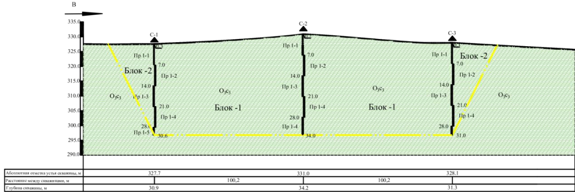
Геологический разрез по профилю I-I
