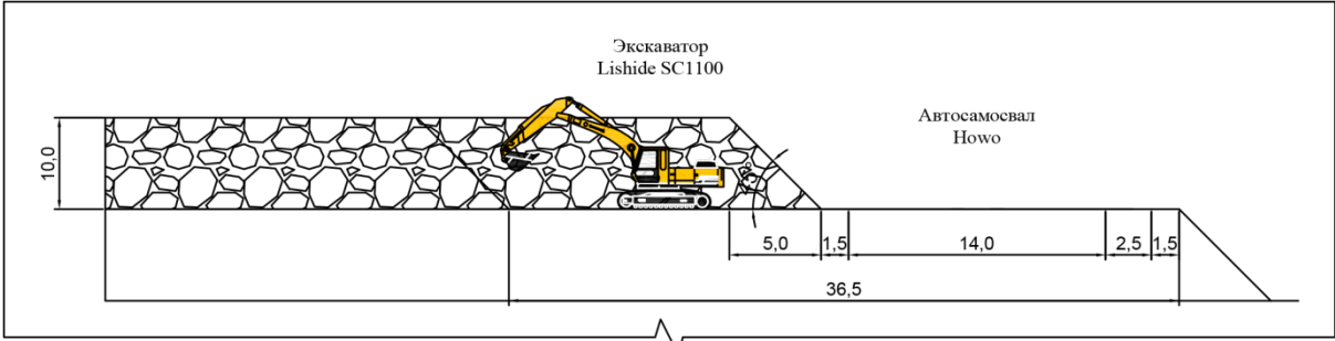
A-A Масштаб 1:200
