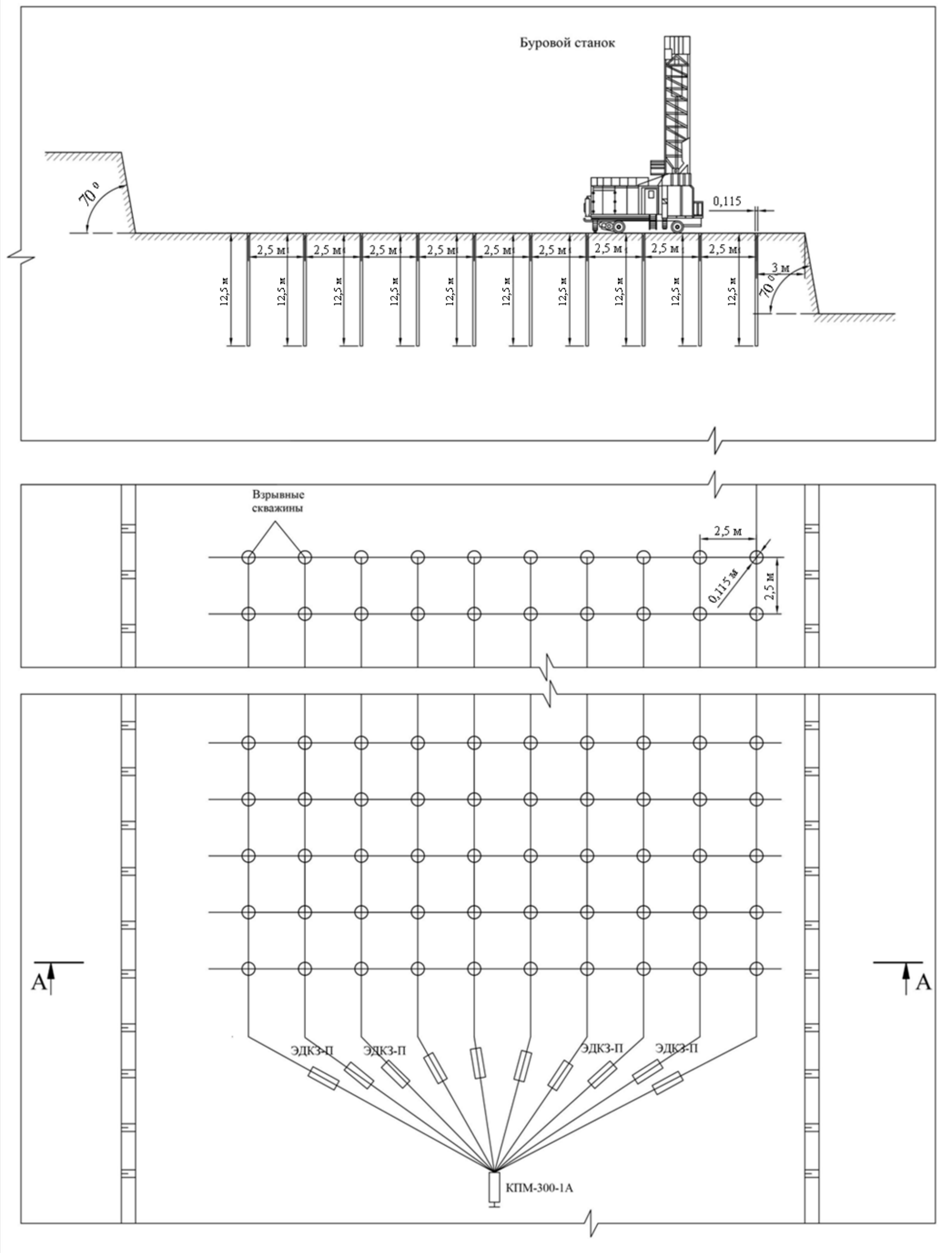
Рис.3. Схема монтажа взрывной сети при производстве БВР
