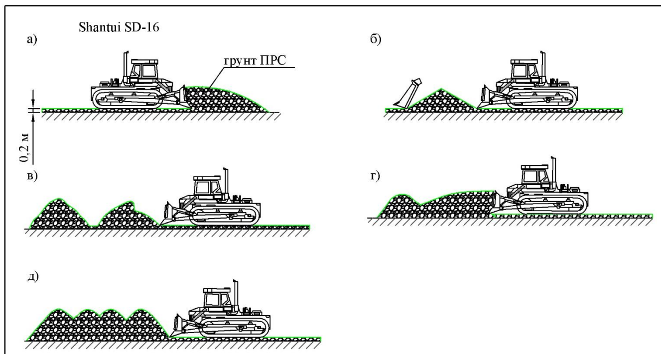
Рис. 7. Схема планировки и укладки ПРС на выположенные поверхности.
