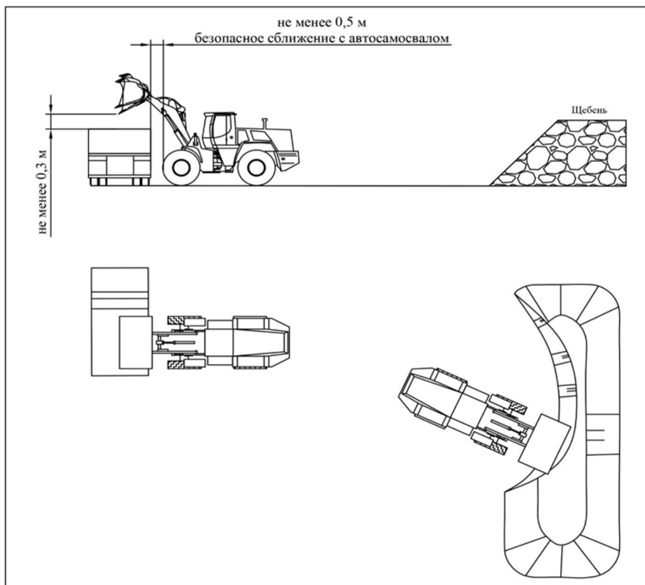
Рис. 5. Технология производства работ на складе известняка
