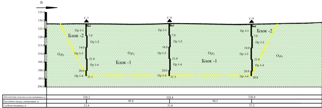
Геологический разрез по профилю III-III
