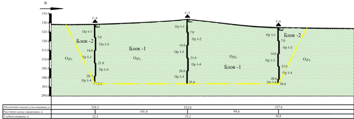
Геологический разрез по профилю II-II
