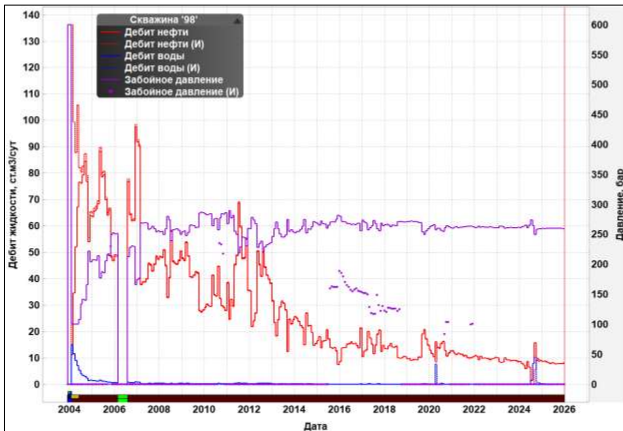
Рисунок 3.3.20 – Дебиты жидкости, нефти и забойное давление – скв №98
