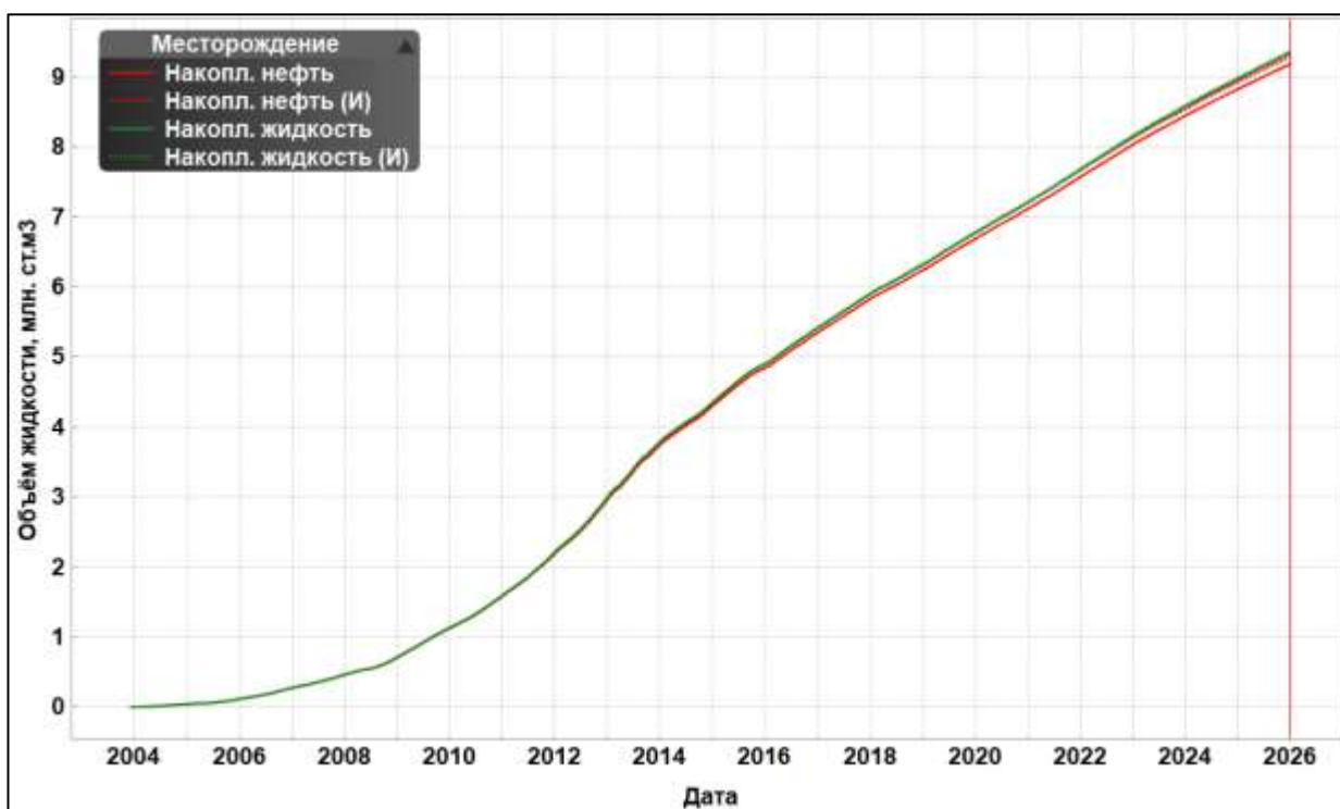
Рисунок 3.3.15 – График адаптации накопленной добычи нефти и жидкости (линии-расчет, точки-факт)
