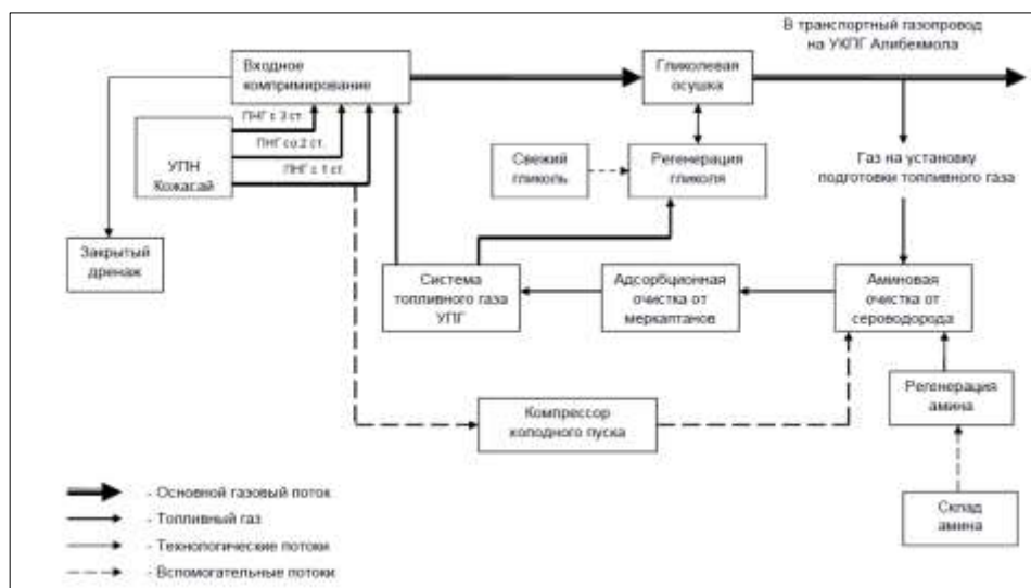
Рисунок 6.4.2 – Принципиальная схема технологического процесса на УПГ Кожасай
