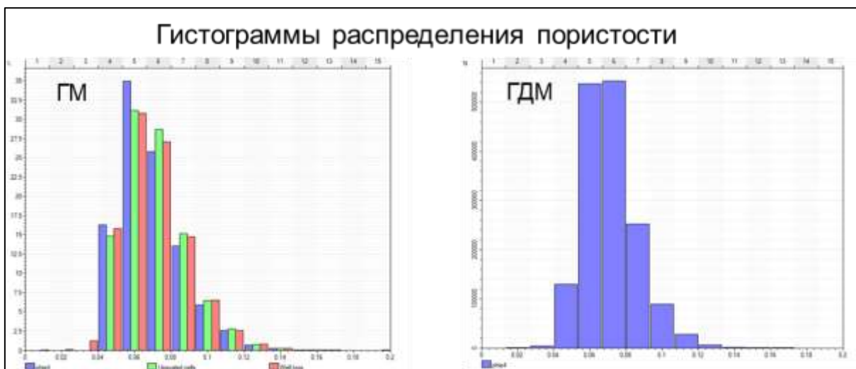
Рисунок 3.3.1 – Сопоставление гистограмм распределения пористости в ГМ и ГДМ
