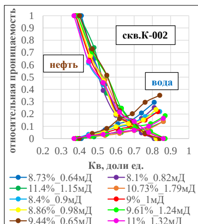
Рисунок 2.4.2 – Кривые относительной проницаемости для системы нефть-вода, толща КТ-II-II
