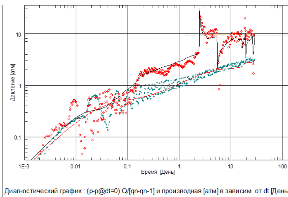
Рисунок 3.1.1 – График КСД в билогарифмических координатах. Скважина №K004
