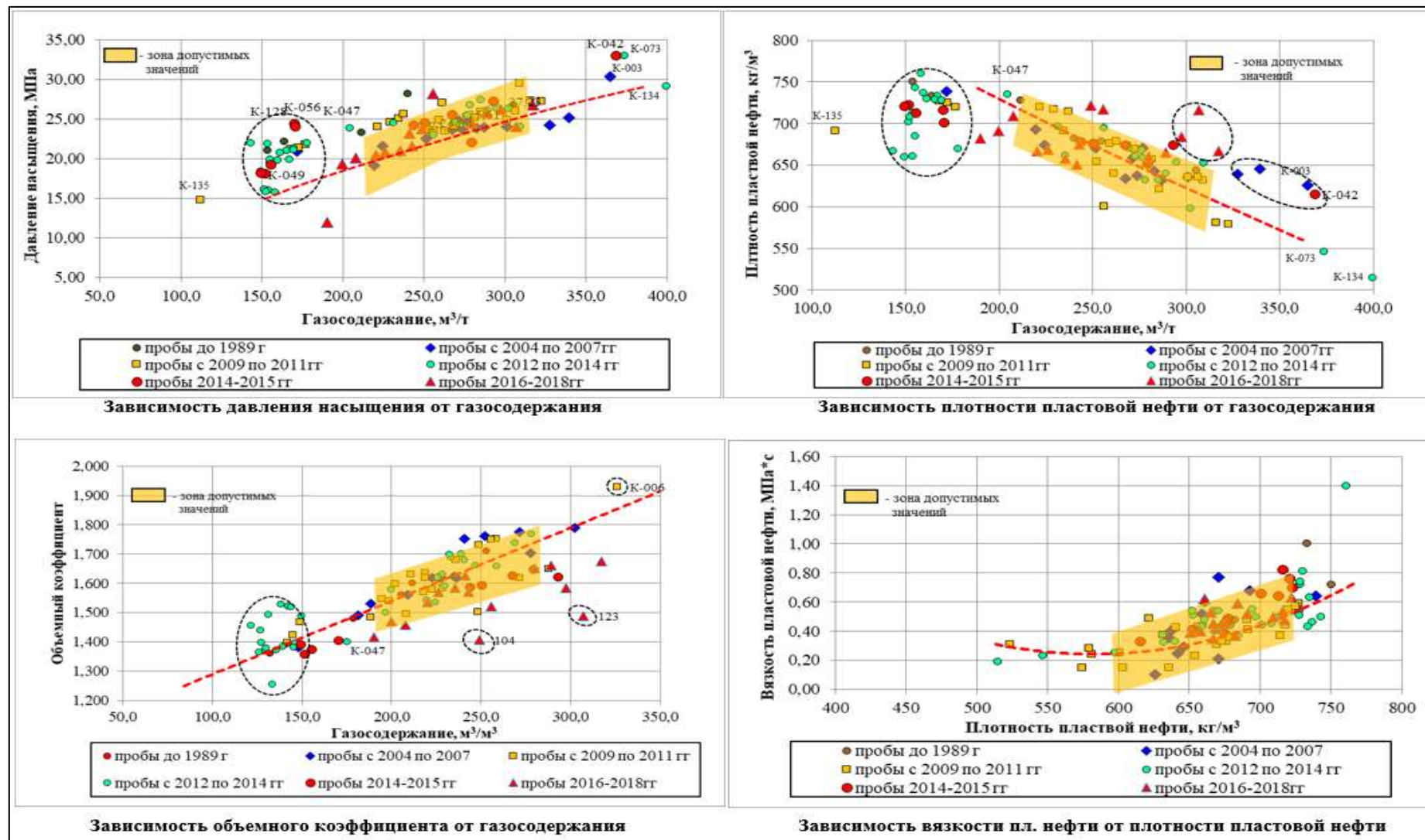
Рисунок 3.3.4 – Анализ зависимости флюидальной модели
