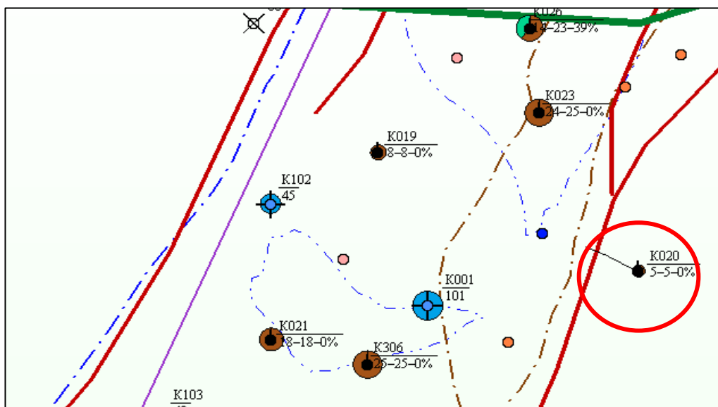
Рисунок 12.1.8 – Схема расположения скважины-кандидата K020
