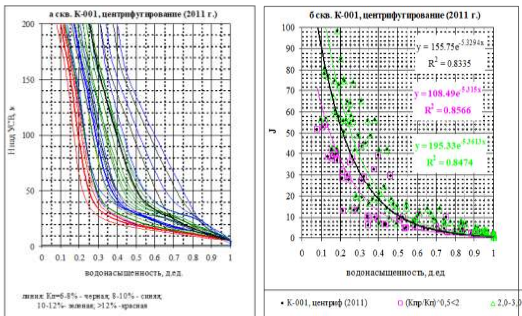
Рисунок 3.3.11 – Определение кривых капиллярного давления
