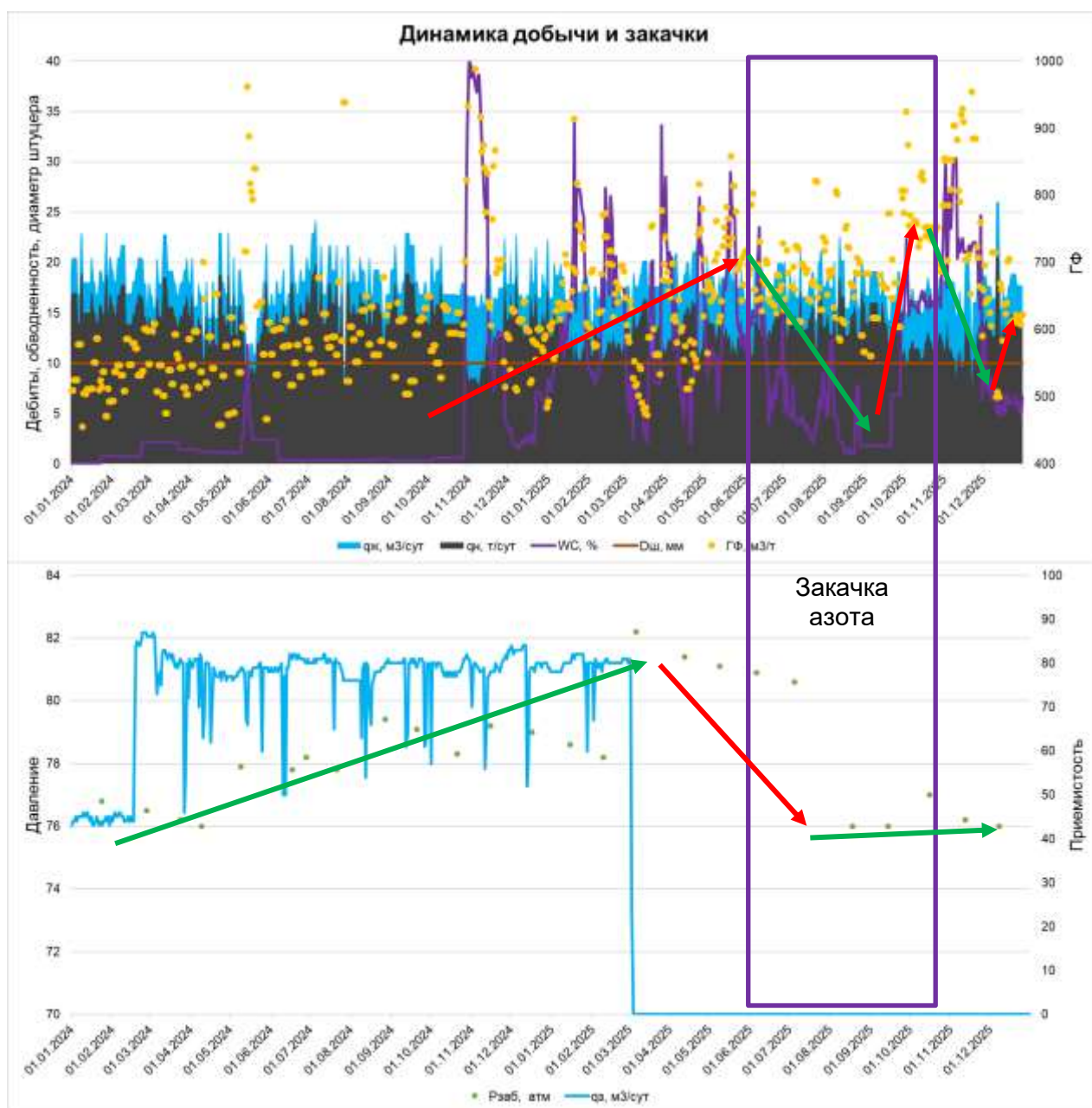
Рисунок 12.1.6 – Динамика добычи и закачки азота на K128
