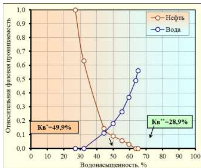
Рисунок 3.3.9 – Определение ОФП по скважине К-001, образец 2808
