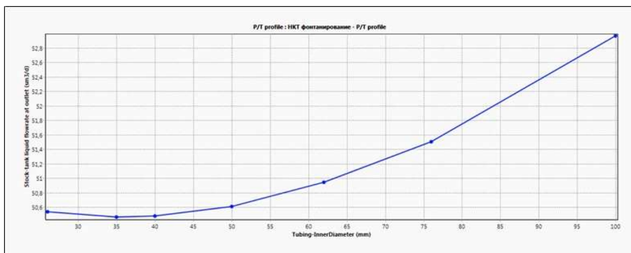
Рисунок 6.1.3 – Зависимость дебита жидкости и внутреннего диаметра НКТ
