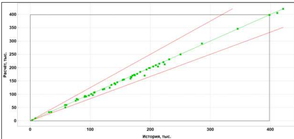
Рисунок 3.3.18 – Кросс-плот накопленной добычи нефти
