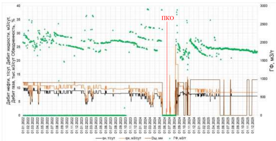
Рисунок 12.1.14 – Основные показатели добычи скважины К098
