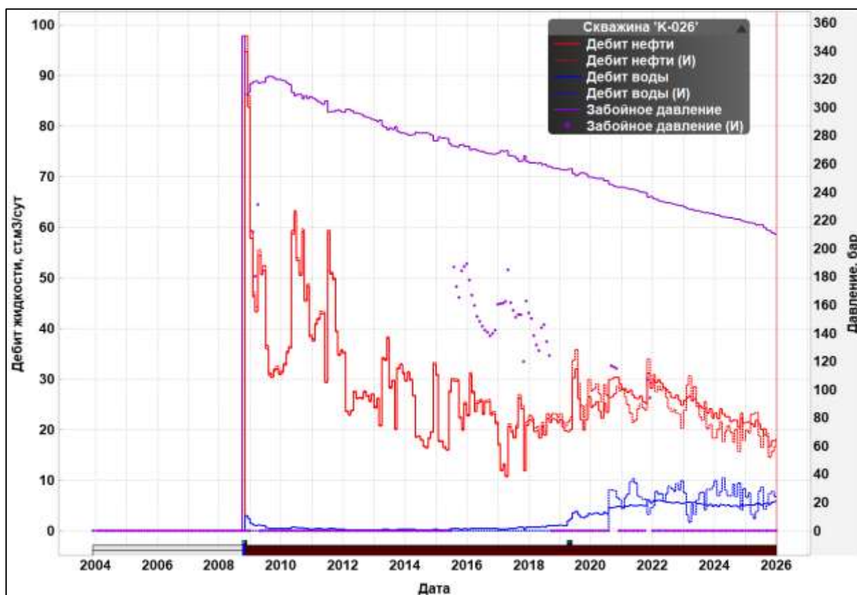
Рисунок 3.3.25 – Дебиты жидкости, нефти и забойное давление – скв №К-026
