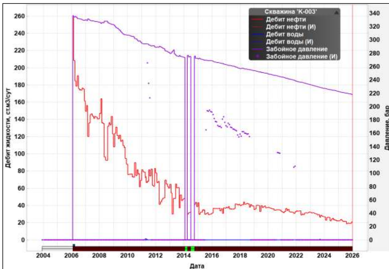
Рисунок 3.3.21 – Дебиты жидкости, нефти и забойное давление – скв №К-003
