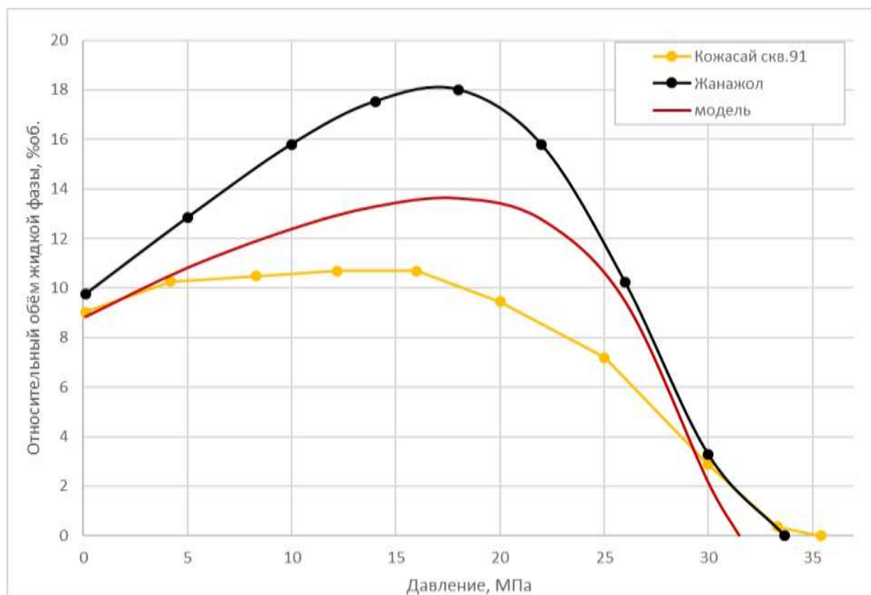
Рисунок 2.3.9 – Изотермы объёма выпавшей жидкой фазы пластового газа скв. 91 (блок 2) при истощении
