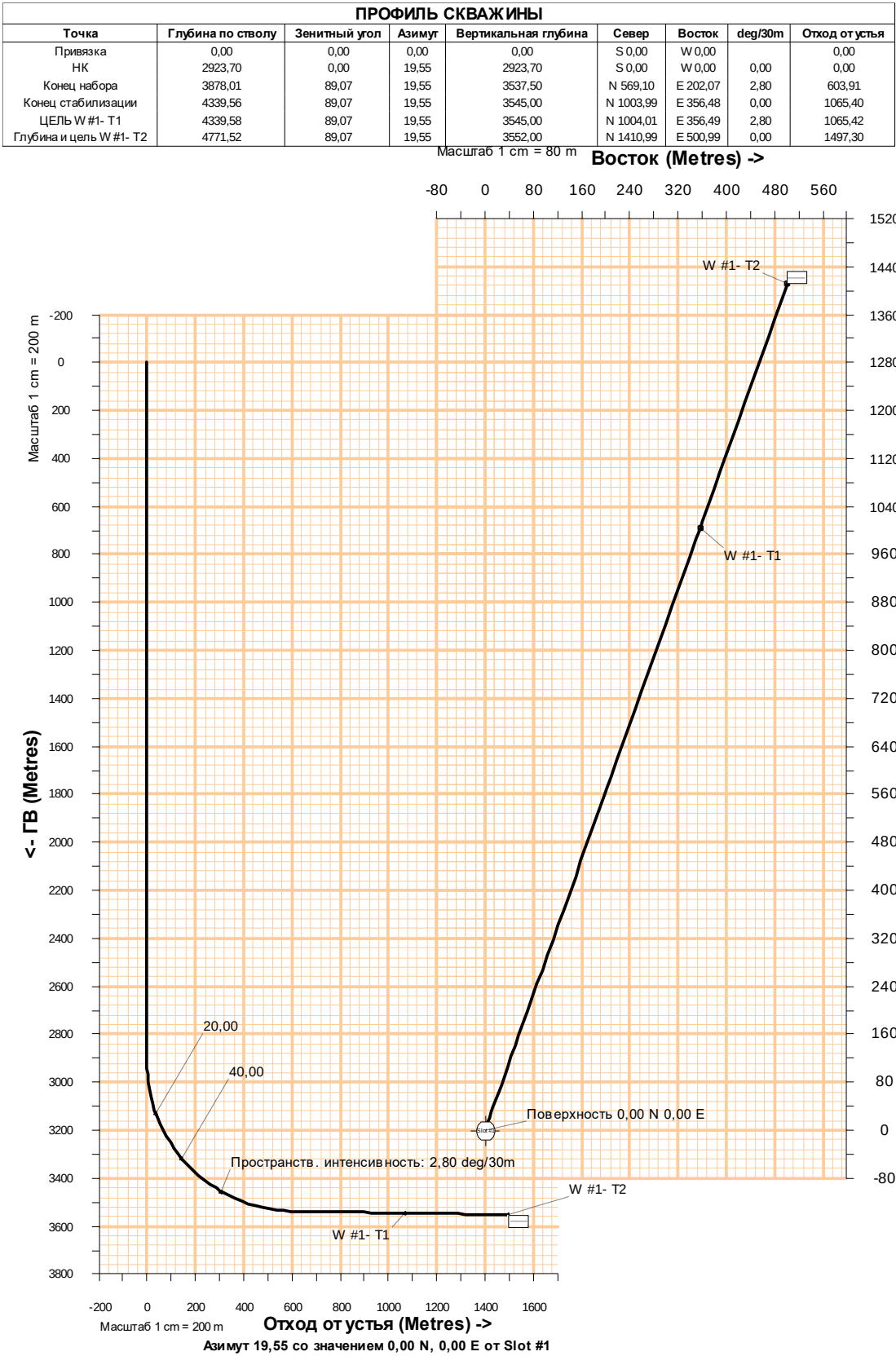
Рисунок 7.1.3 – Профиль горизонтальной скважины ГС-2
