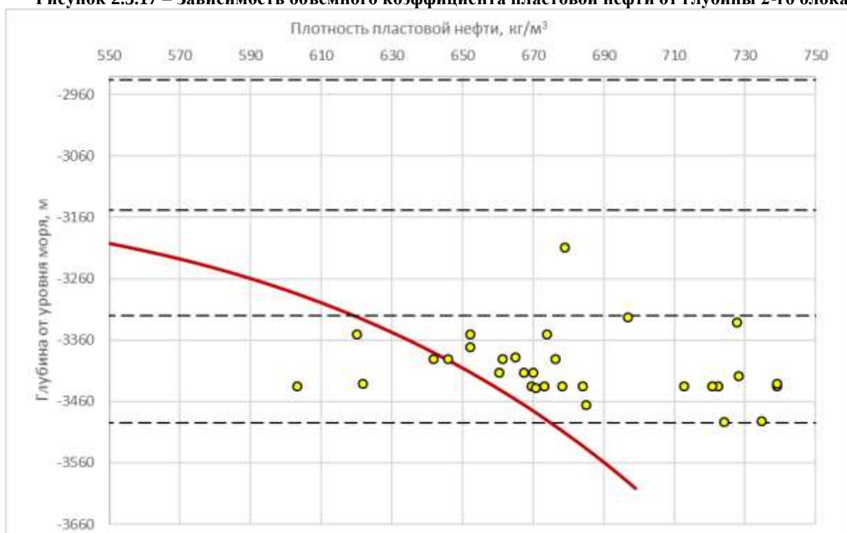
Рисунок 2.3.18 – Зависимость плотности пластовой нефти от глубины 2-го блока
