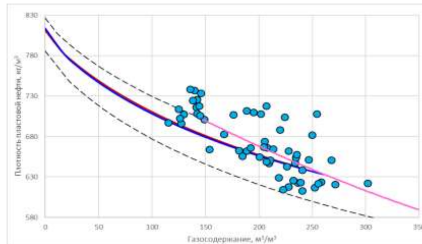
Рисунок 2.3.2 – Плотность от газосодержания пластовой нефти 1-го блока
