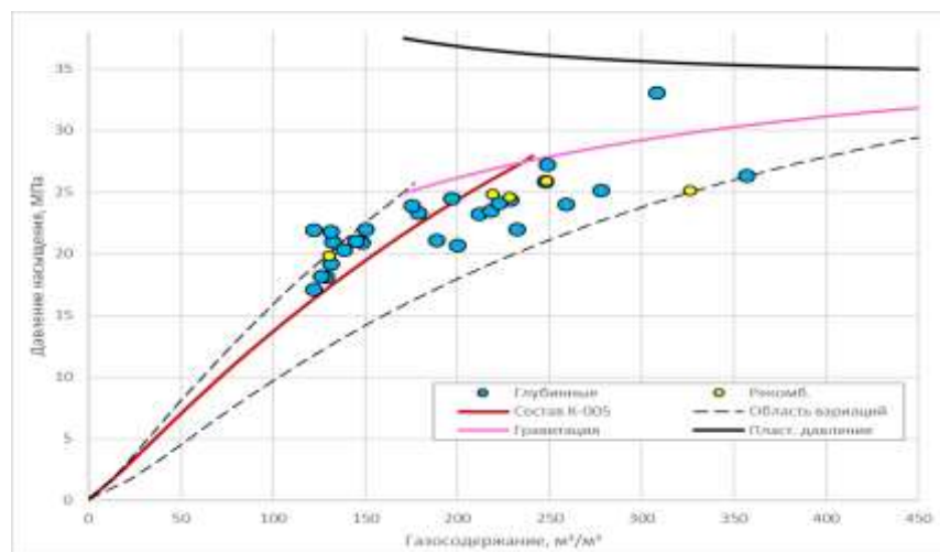
Рисунок 2.3.5 – Давление насыщения от газосодержания пластовой нефти 2-го блока
