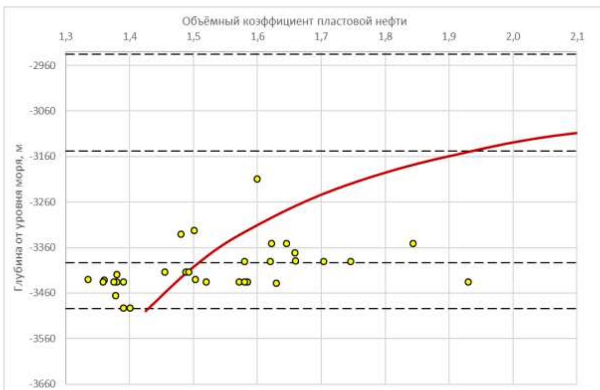
Рисунок 2.3.17 – Зависимость объёмного коэффициента пластовой нефти от глубины 2-го блока
