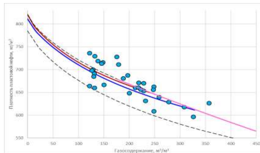
Рисунок 2.3.6 – Плотность от газосодержания пластовой нефти 2-го блока
