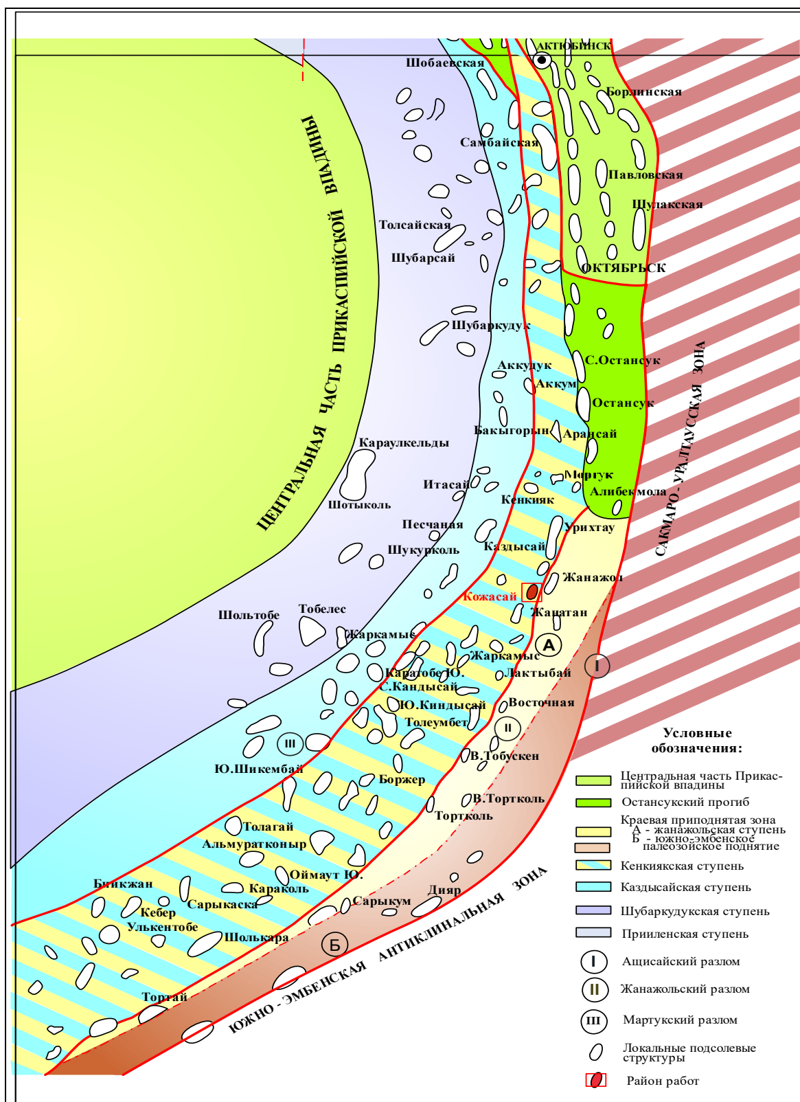
Рисунок 2.1.1 – Тектоническая схема подсолевых отложений Восточной части Прикаспийской впадины
