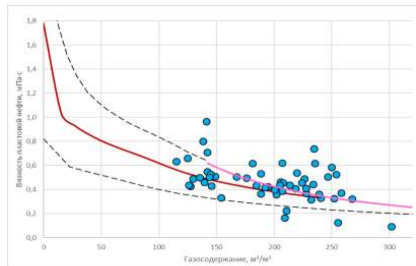
Рисунок 2.3.3 – Вязкость от газосодержания пластовой нефти 1-го блока
