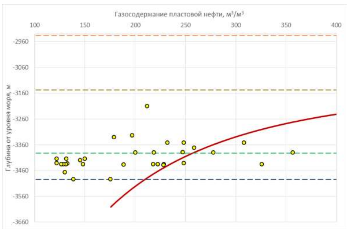
Рисунок 2.3.16 – Зависимость газосодержания пластовой нефти от глубины 2-го блока
