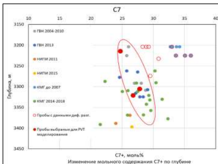
Рисунок 3.3.6 – Расположение выбранных проб по глубине
