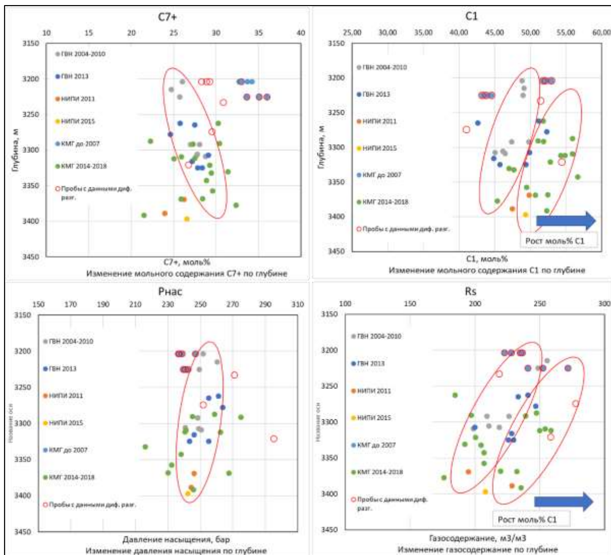
Рисунок 3.3.5 – Анализ зависимости компонентного состава флюидальной модели
