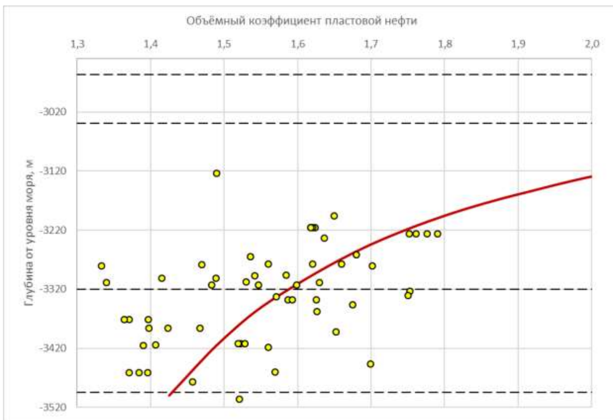
Рисунок 2.3.12 – Зависимость объёмного коэффициента пластовой нефти от глубины 1-го блока
