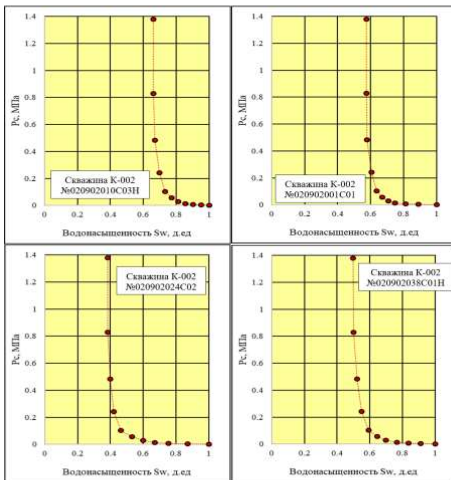
Рисунок 3.3.12 – Кривые капиллярного давления по скважине К-002
