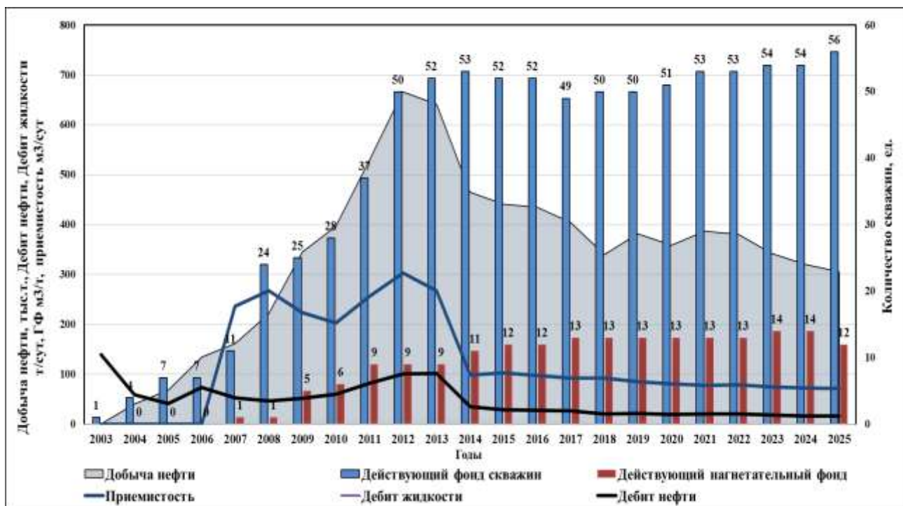
Рисунок 3.2.7 – Технологические показатели разработки месторождения с начала разработки
