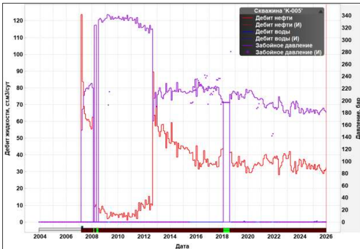
Рисунок 3.3.19 – Дебиты жидкости, нефти и забойное давление – скв №К-005
