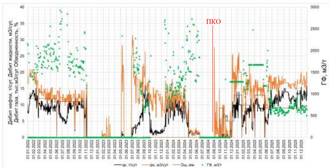
Рисунок 12.1.15 – Основные показатели добычи скважины К135
