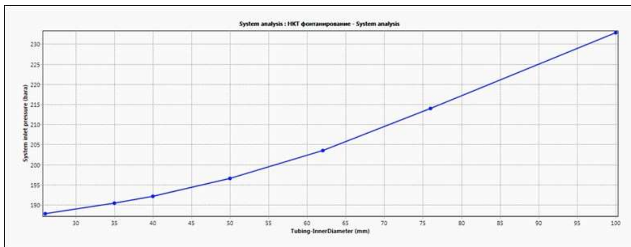
Рисунок 6.1.4 – Зависимость забойного давления и внутреннего диаметра НКТ
