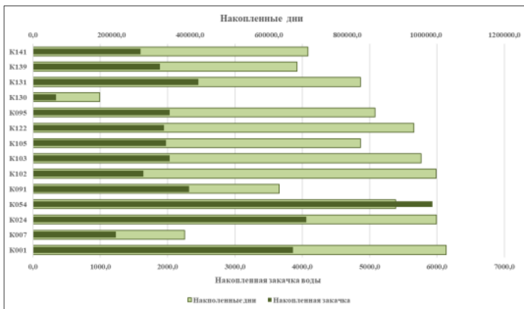
Рисунок 3.2.8 – Накопленное время нагнетания, объемы закачки воды по скважинам на 01.01.2026 г
