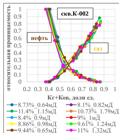
Рисунок 2.4.3 – Кривые относительной проницаемости для системы нефть-газ, толща КТ-II-II
