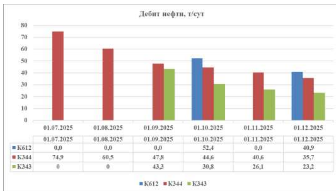
Рисунок 3.2.1 – График дебита нефти в скважинах №К612, К344, К343
