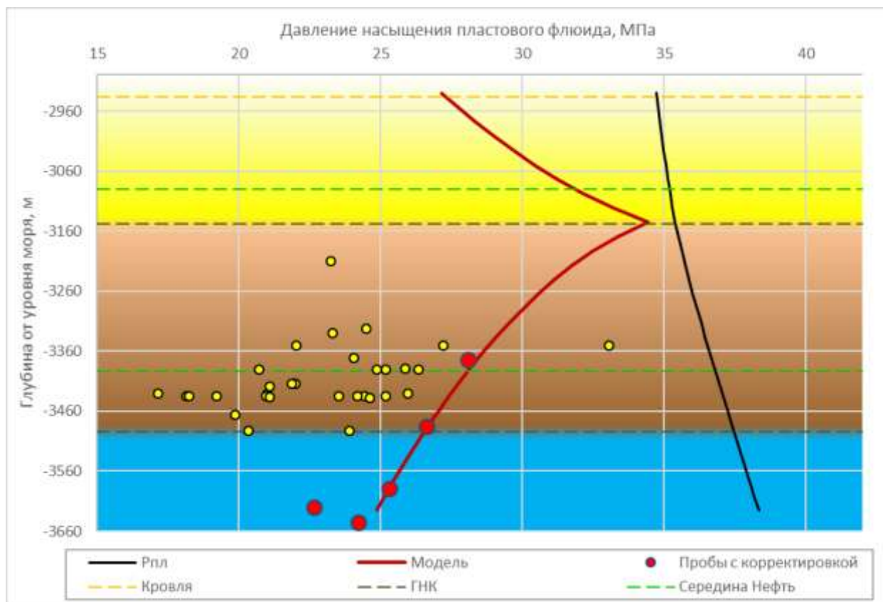
Рисунок 2.3.15 – Зависимость давления насыщения пластовой нефти от глубины 2-го блока
