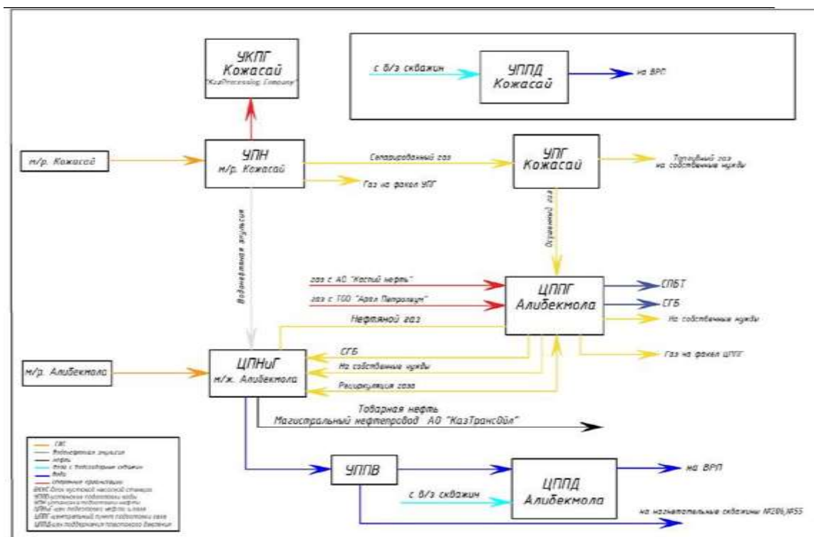
Рисунок 6.4.1 – Блок-схема существующих объектов газопереработки ТОО «Казахойл Актөбе»
