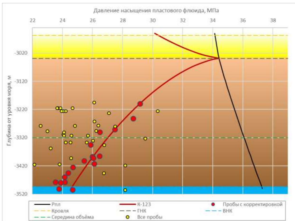
Рисунок 2.3.10 – Зависимость давления насыщения пластовой нефти от глубины 1-го блока
