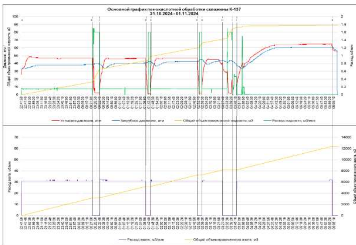
Рисунок 12.1.11 – График пенокислотной обработки скважины К-137
