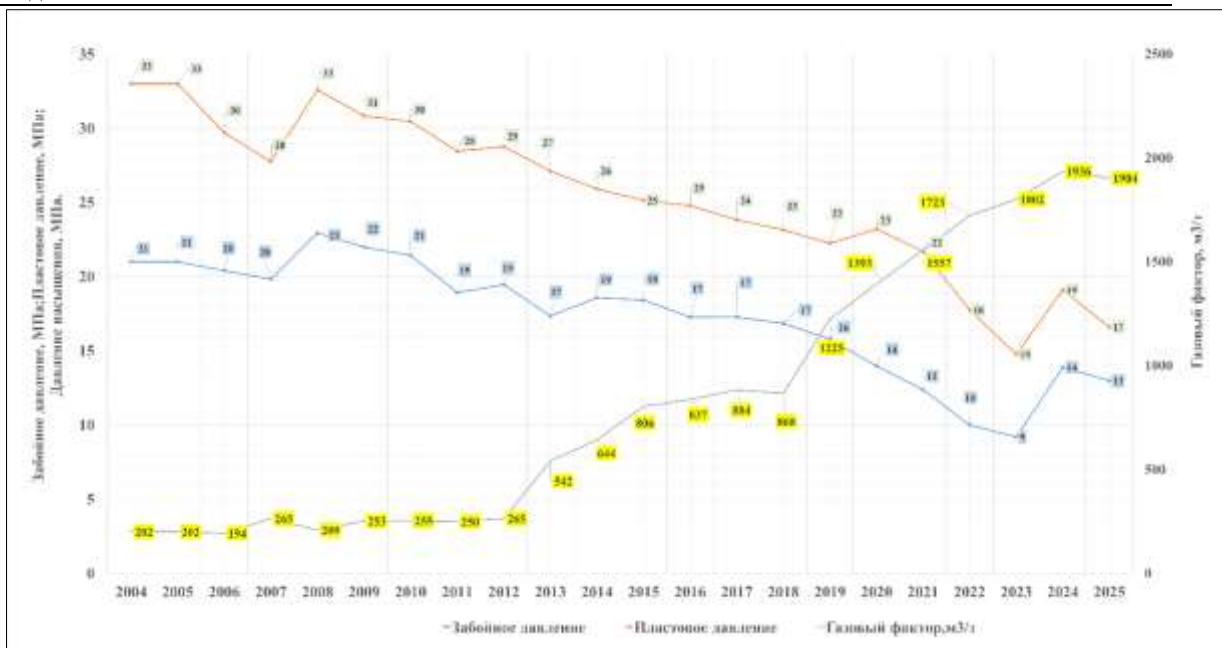
Рисунок 3.1.2 – Динамика пластовых, забойных давлений и газового фактора с начала разработки
