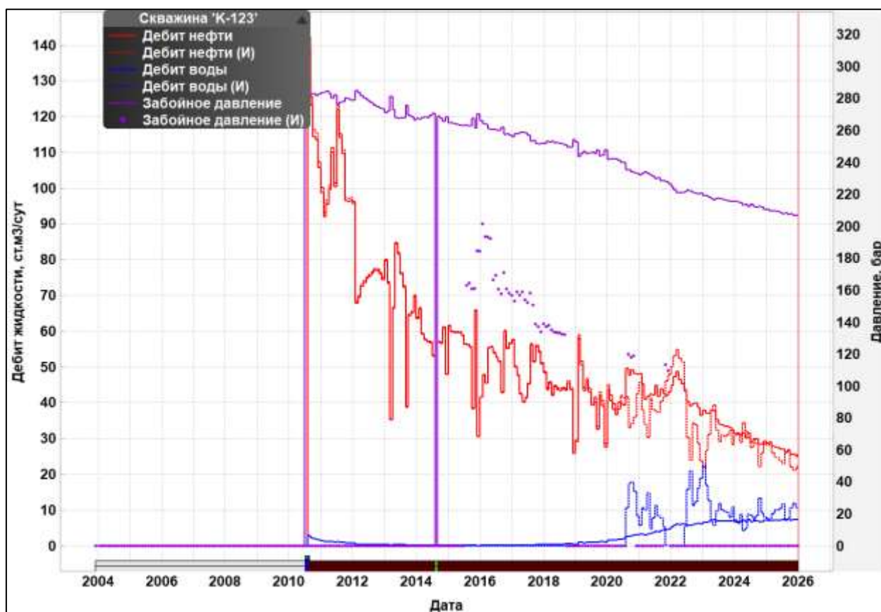
Рисунок 3.3.27 – Дебиты жидкости, нефти и забойное давление – скв №К-123
