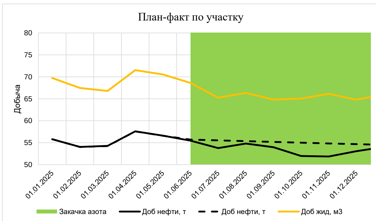
Рисунок 12.1.7 – Динамика добычи жидкости и нефти в ходе реализации технологии закачки азота
