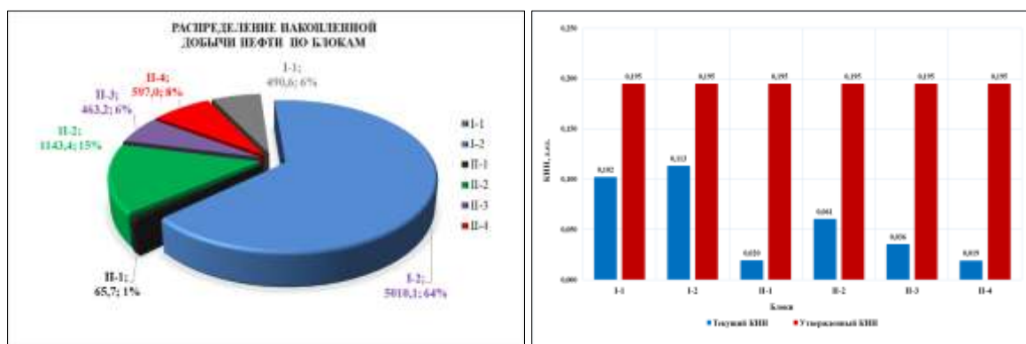
Рисунок 3.2.10 – Распределение накопленной добычи нефти и значений КИН по блокам
