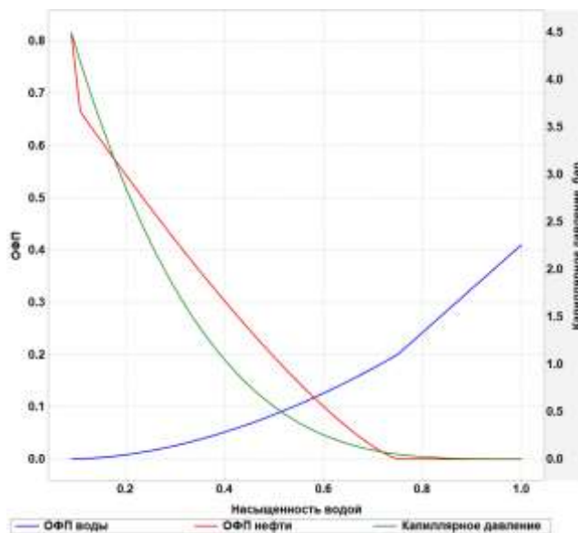
Рисунок 3.3.13 – ОФП в системе нефть-вода
