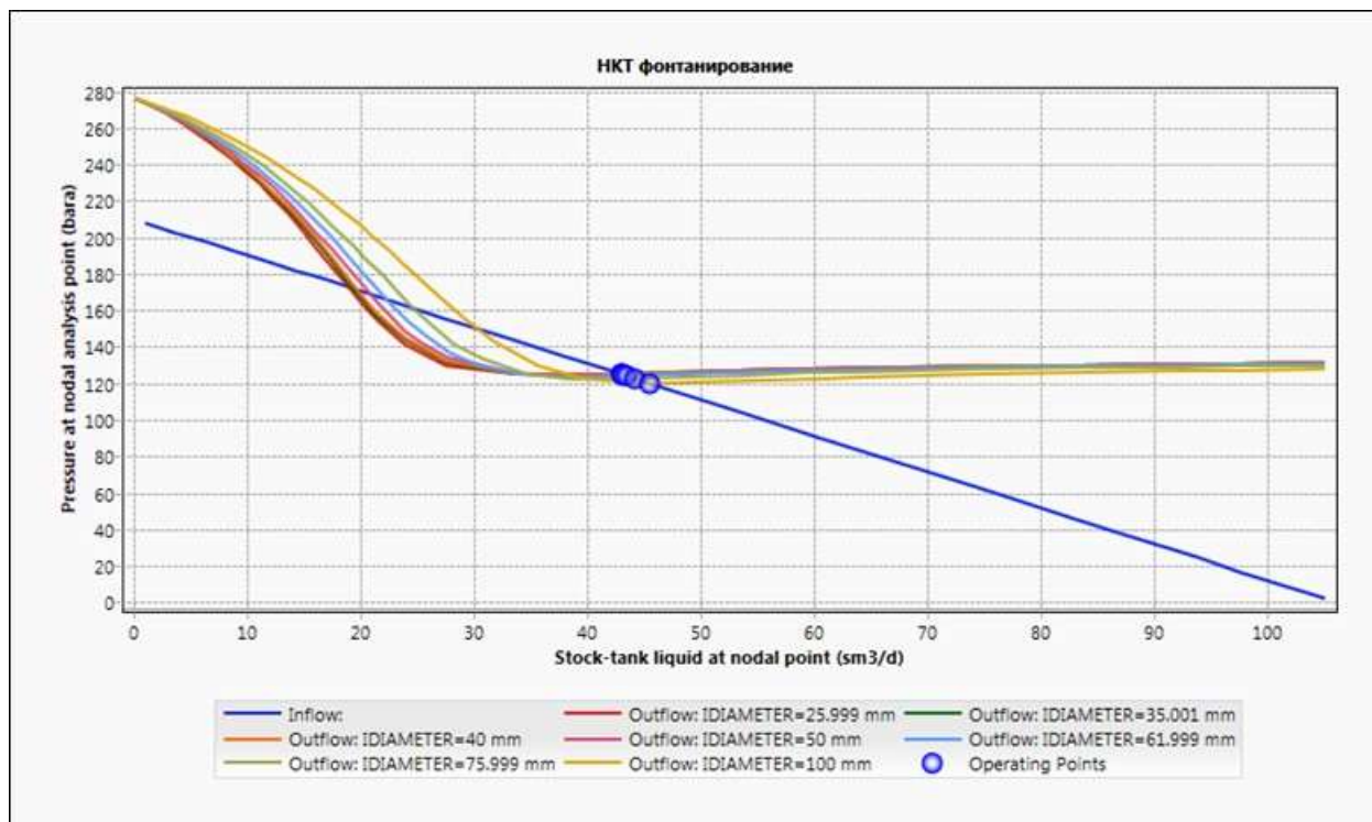
Рисунок 6.1.2 – Сравнение условий работы подъёмников при разных диаметрах
