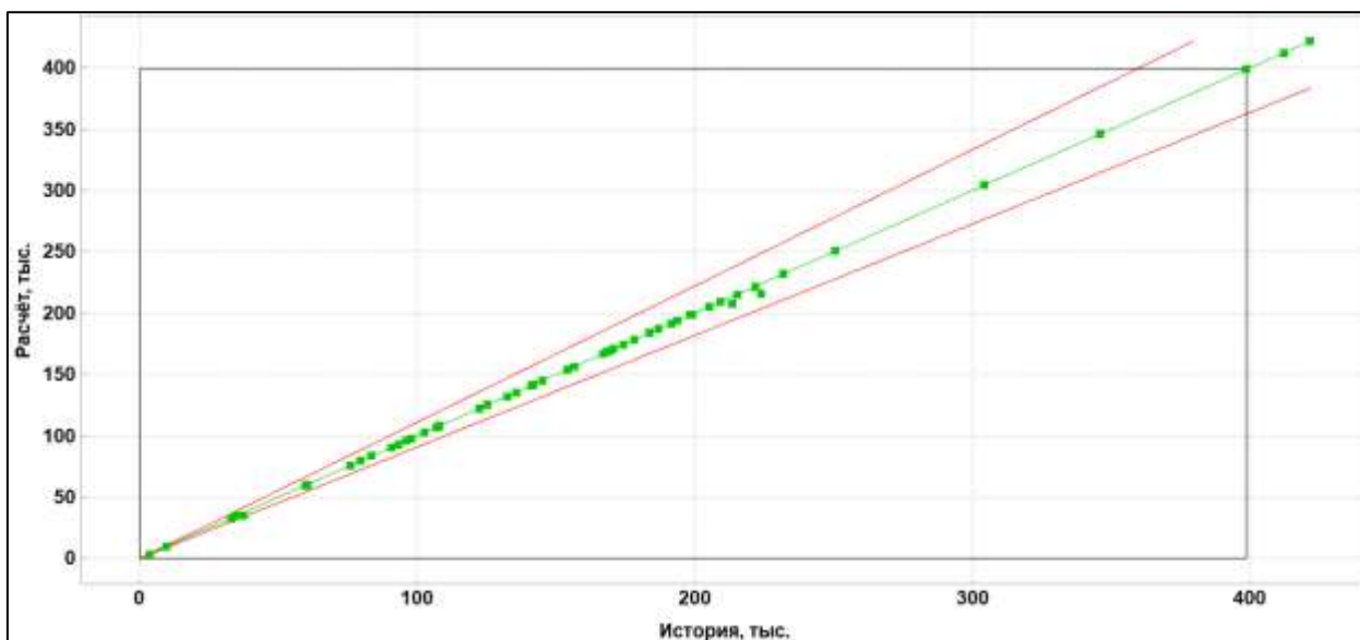
Рисунок 3.3.17 – Кросс-плот накопленной добычи жидкости
