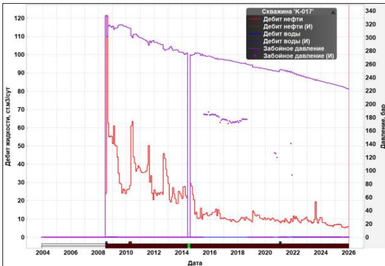
Рисунок 3.3.23 – Дебиты жидкости, нефти и забойное давление – скв №К-017
