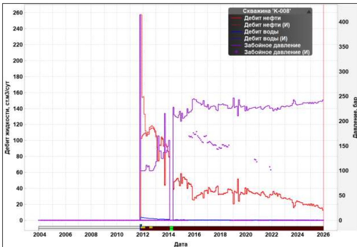
Рисунок 3.3.22 – Дебиты жидкости, нефти и забойное давление – скв №К-008
