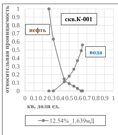
Рисунок 2.4.1 – Кривые относительной проницаемости для системы нефть-вода, толща КТ-II-I
