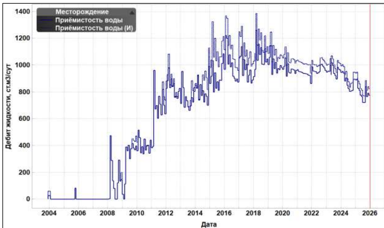
Рисунок 3.3.16 – График адаптации приемистости воды (линии-расчет, точки-факт)
