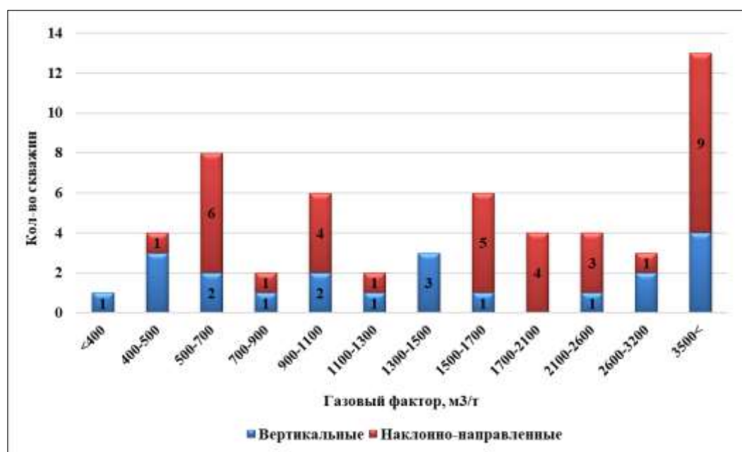
Рисунок 3.2.2 – Распределение действующего фонда добывающих скважин по газовому фактору на 01.01.2026г
