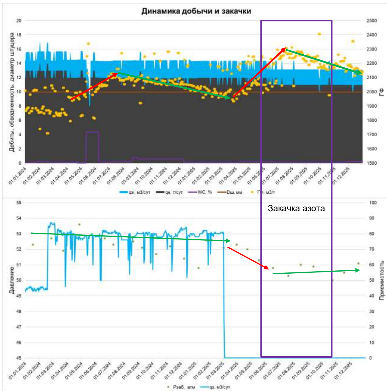
Рисунок 12.1.5 – Динамика добычи и закачки азота на K071
