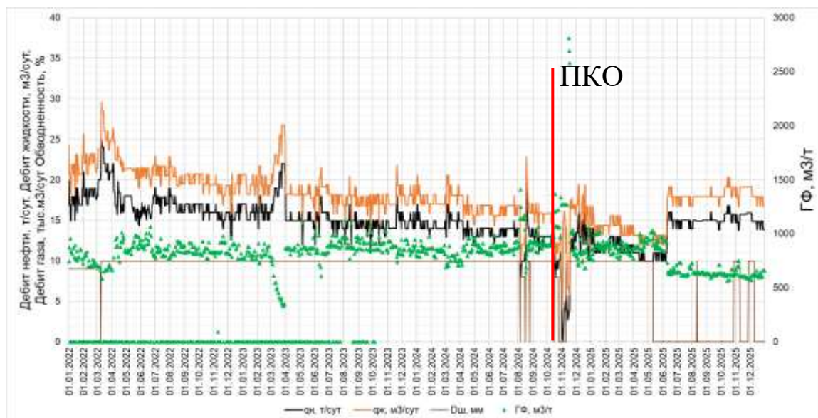
Рисунок 12.1.12 – График добычи после ПКО скв. К-137
