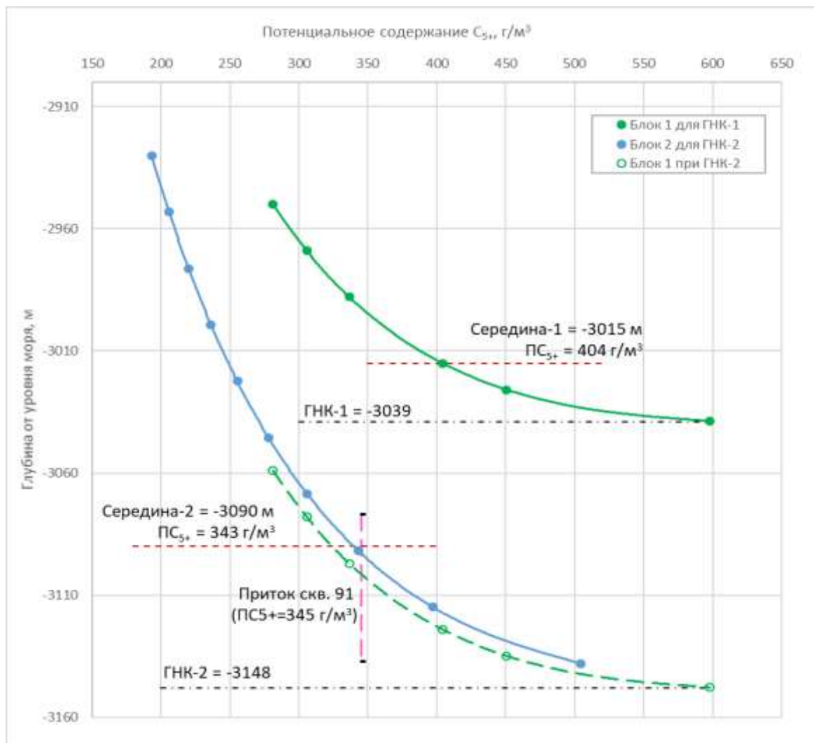
Рисунок 2.3.20 – Изменение потенциальное содержание C_{5+} на пластовый газ от глубины
