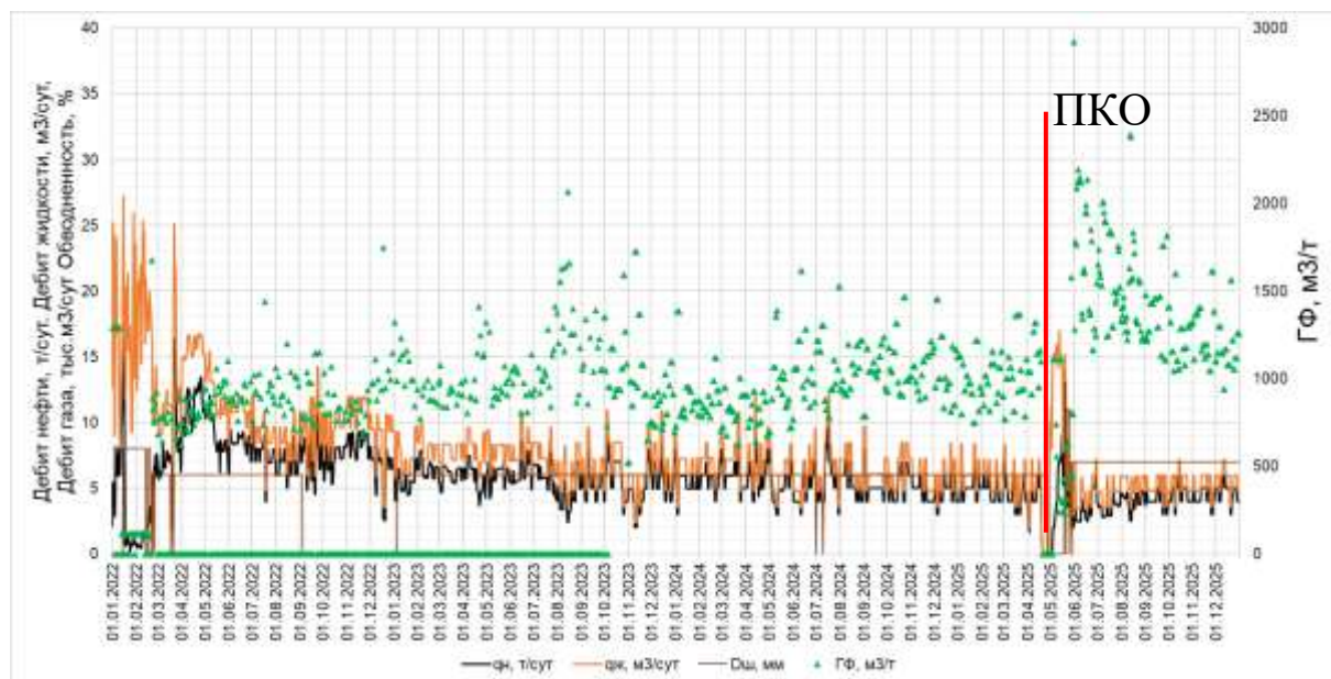
Рисунок 12.1.13 – График добычи после ПКО скв. К-086
