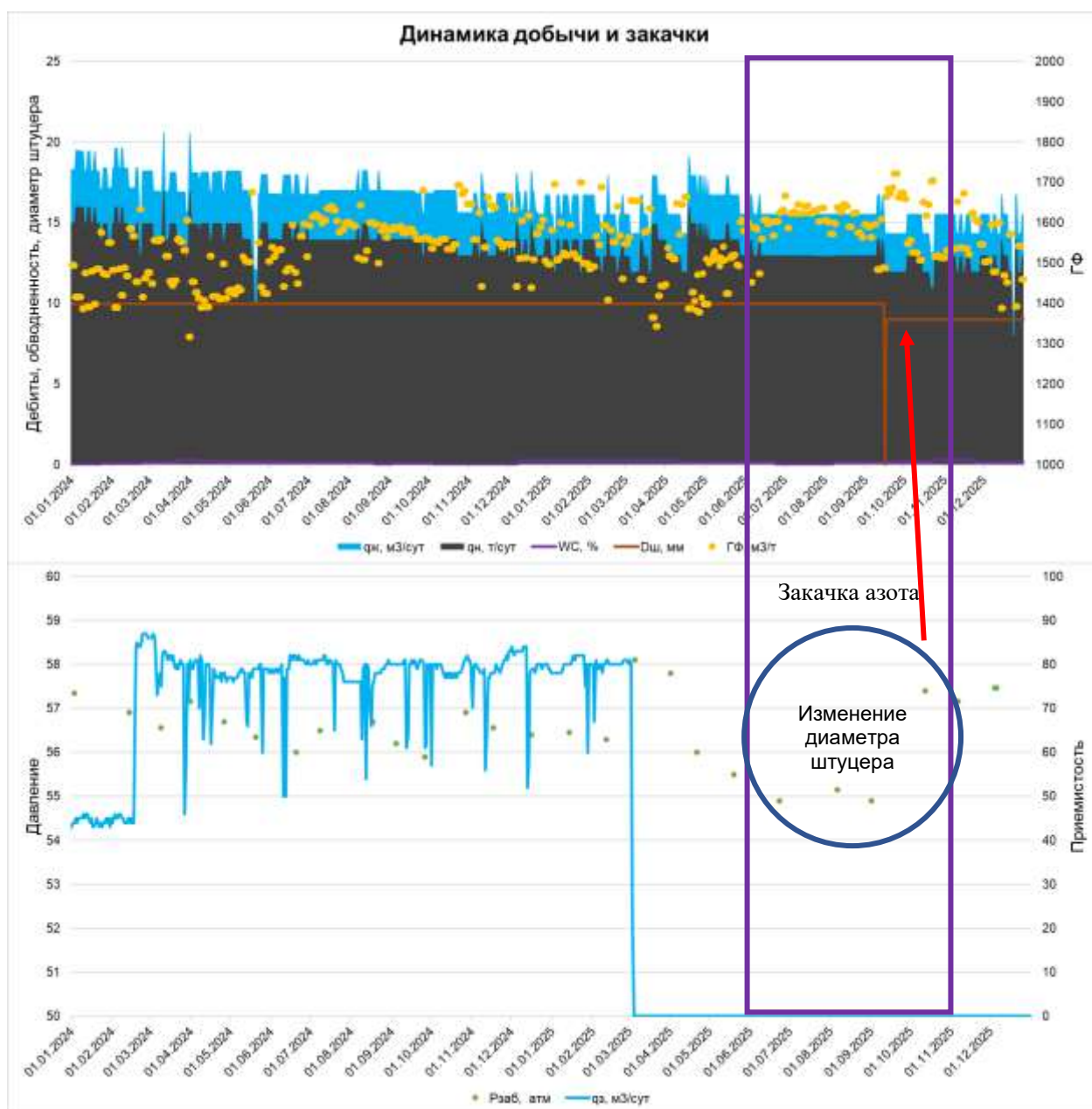
Рисунок 12.1.3 – Динамика добычи и закачки азота на K104
