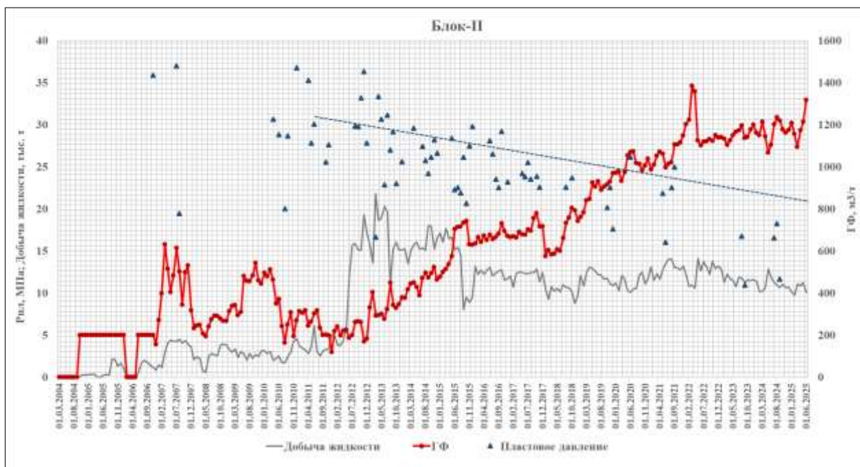
Рисунок 3.1.4 – Динамика пластового давления, ГФ, добычи жидкости по блоку II
