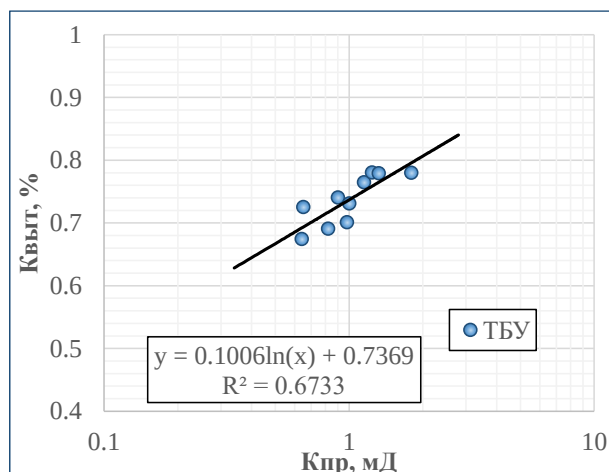
Рисунок 2.4.6 – Зависимость коэффициента вытеснения от проницаемости
