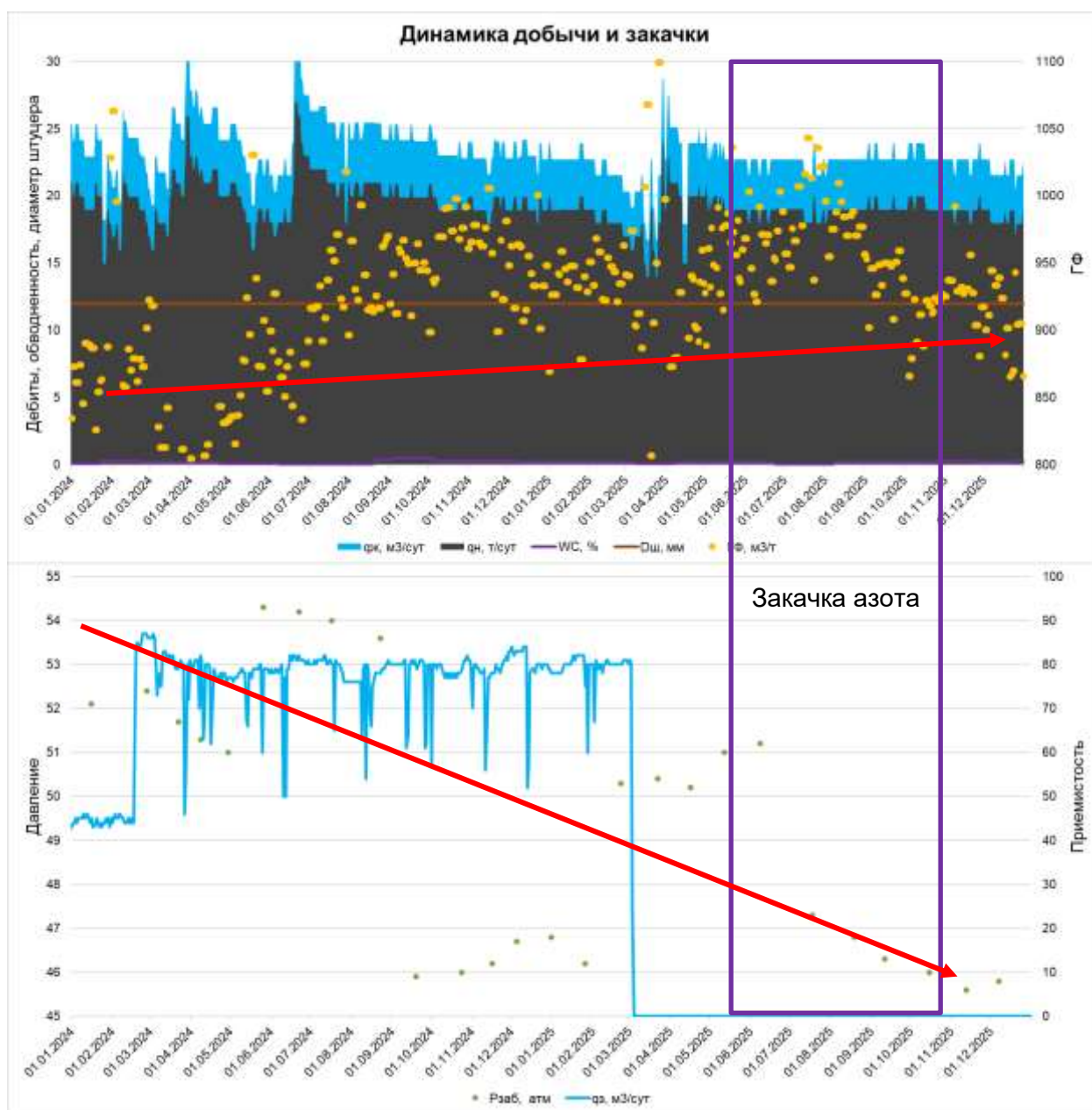
Рисунок 12.1.4 – Динамика добычи и закачки азота на К126
