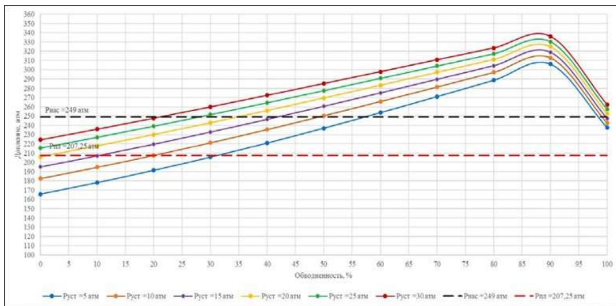
Рисунок 6.1.1 – Минимальные забойные давления для фонтанирования при различных устьевых давлениях и обводненности объекта КТ-II
