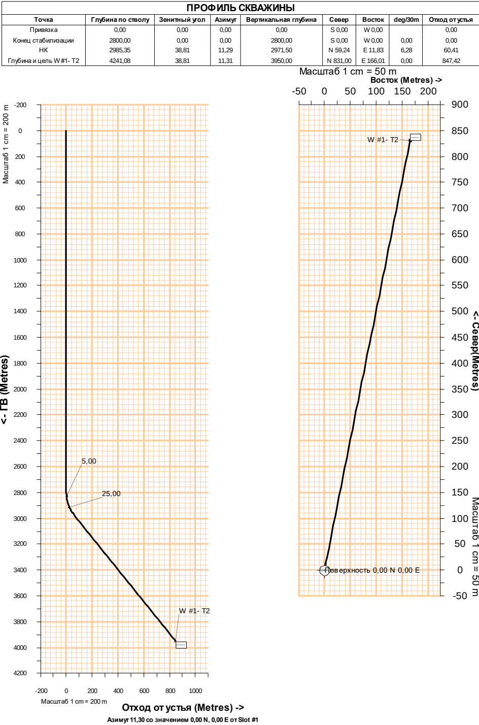
Рисунок 7.1.1 – Профиль наклонно-направленной скважины
