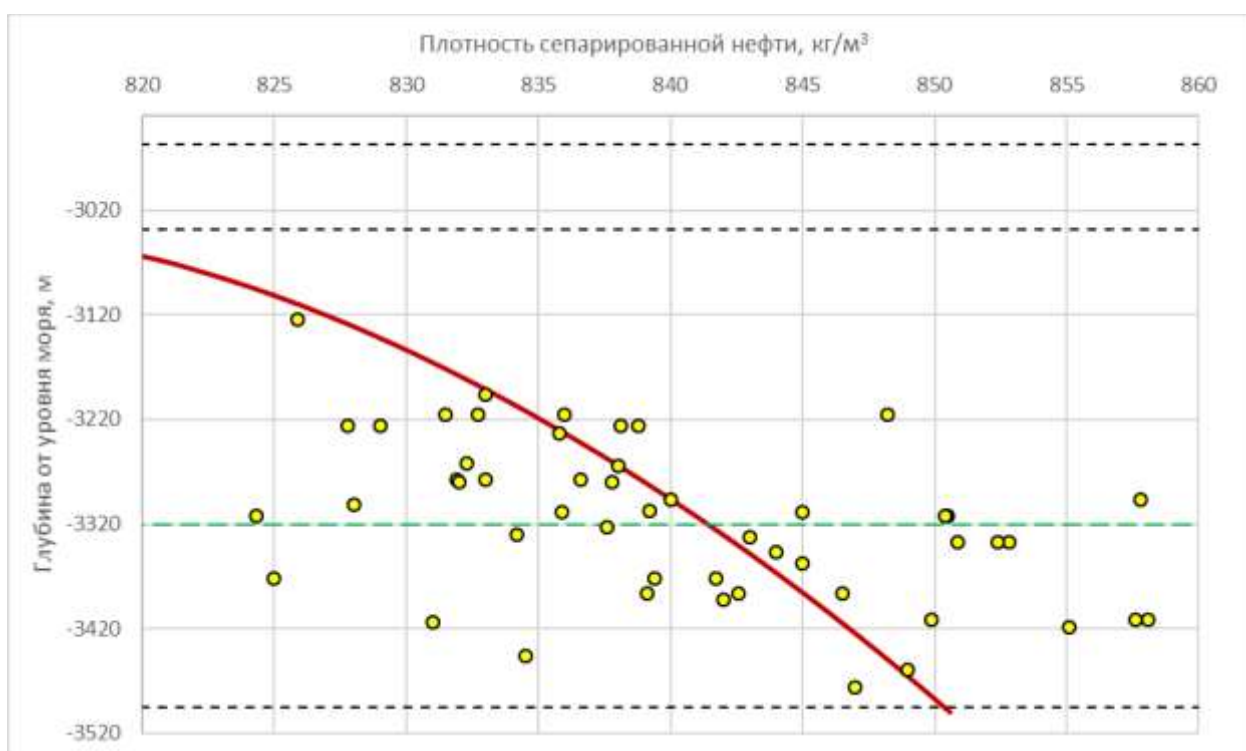
Рисунок 2.3.14 – Зависимость плотности сепарированной нефти от глубины 1-го блока
