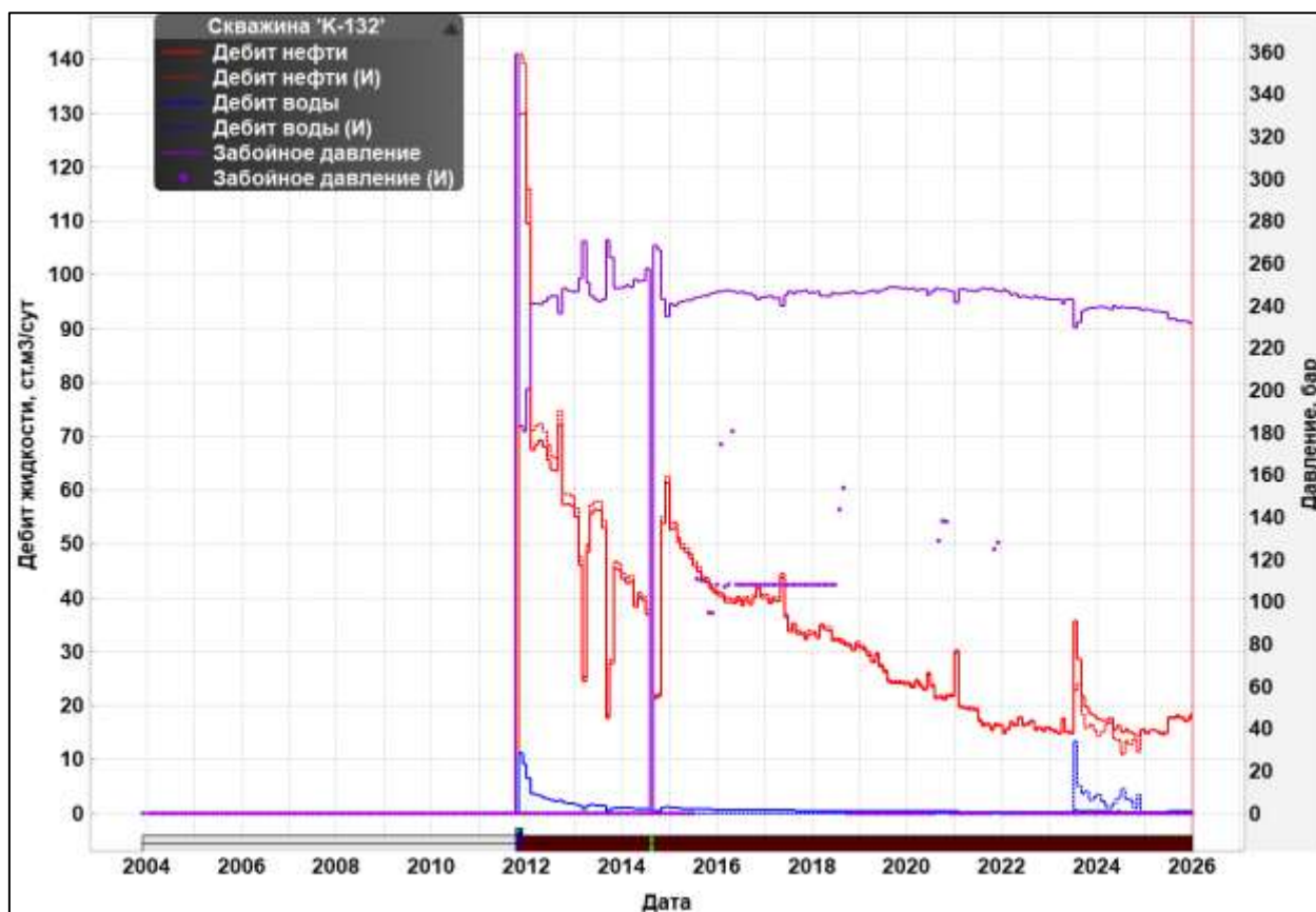
Рисунок 3.3.26 – Дебиты жидкости, нефти и забойное давление – скв №К-132
