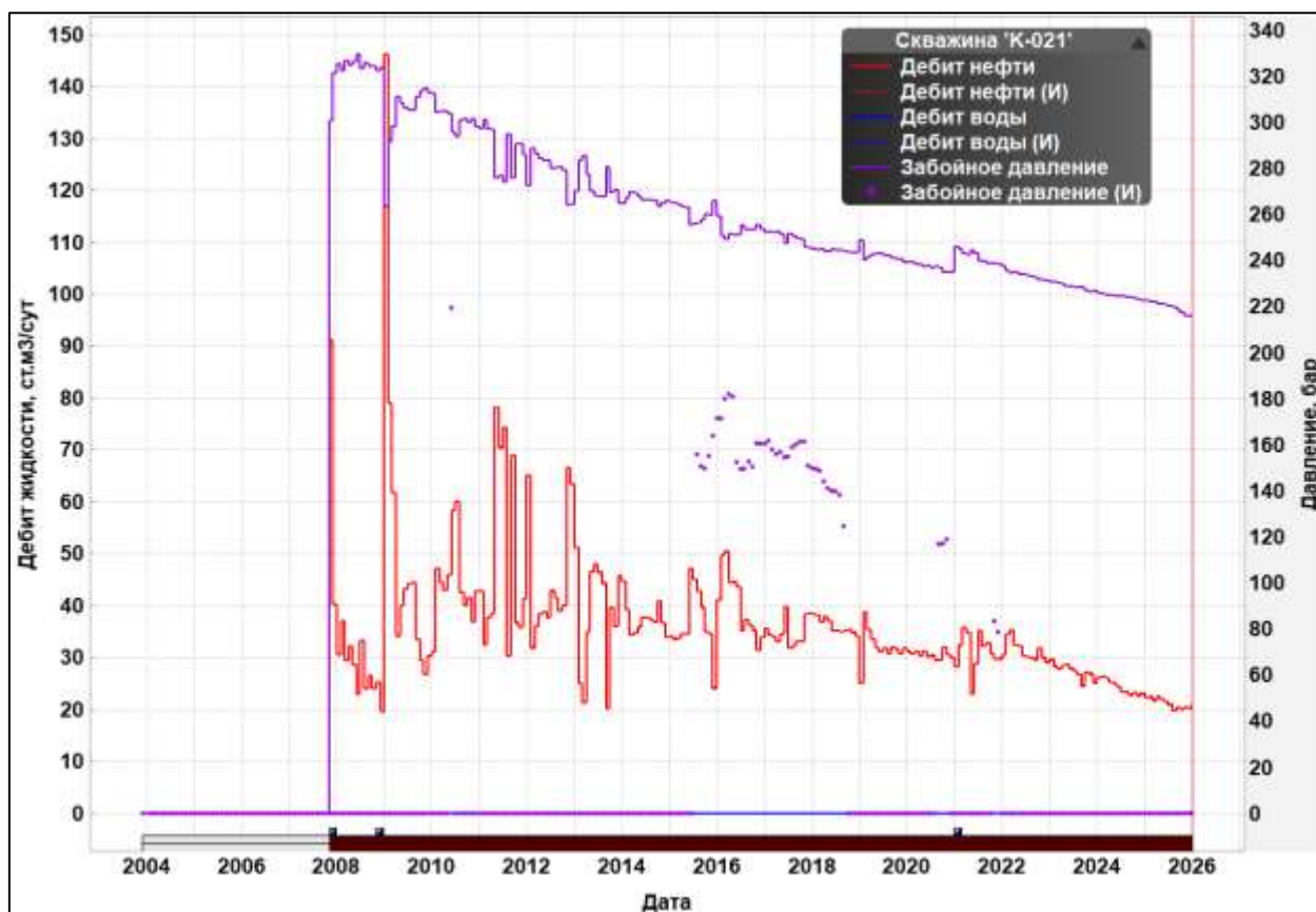
Рисунок 3.3.24 – Дебиты жидкости, нефти и забойное давление – скв №К-021
