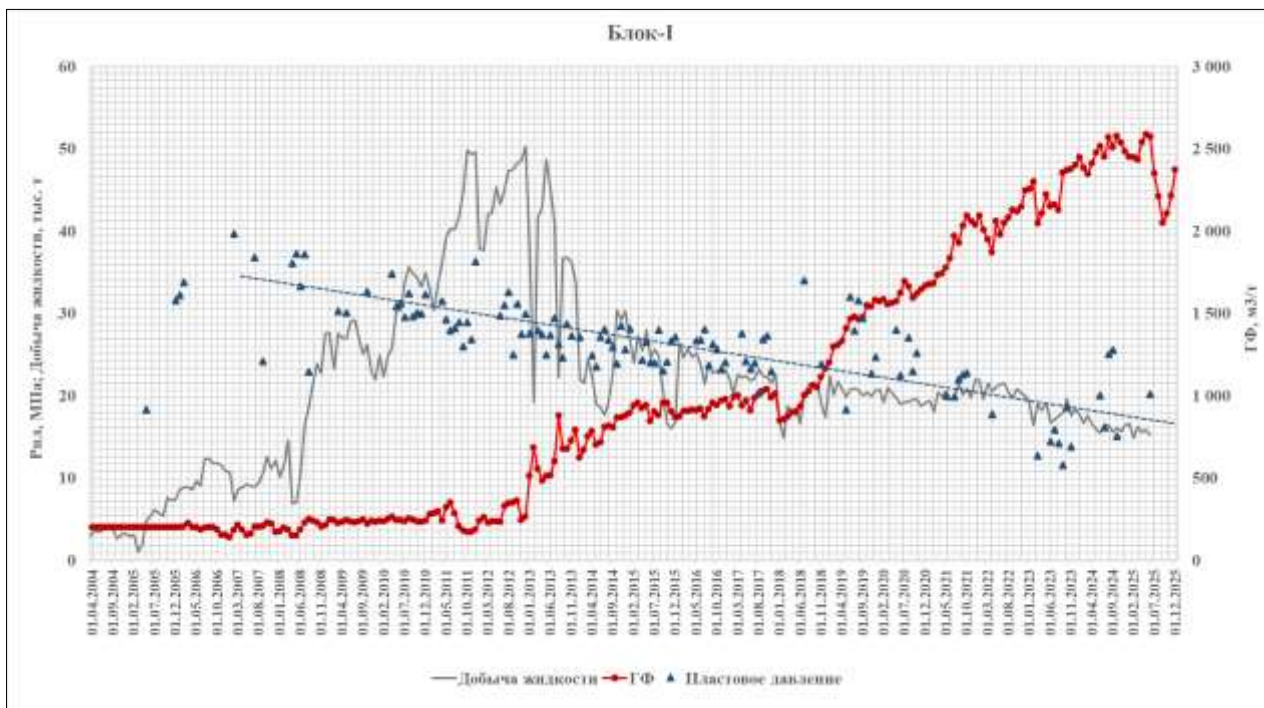
Рисунок 3.1.3 – Динамика пластового давления, ГФ, добычи жидкости по блоку I
