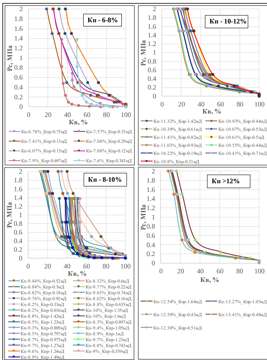
Рисунок 2.4.4 – Кривые капиллярного давления по классам пористости K_p = 6-8, 8-10, 10-12 и >12\%
