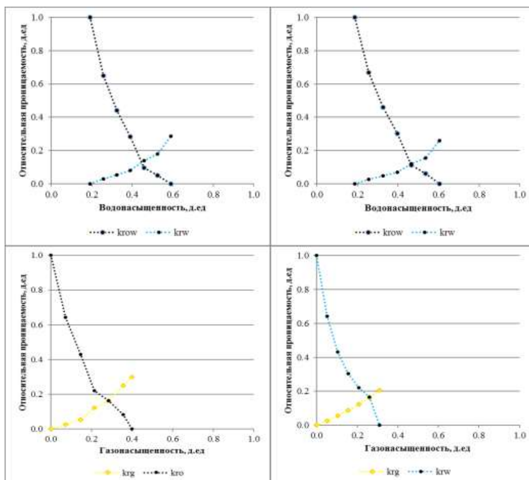
Рисунок 3.3.10 – Определение ОФП по скважине К-002
