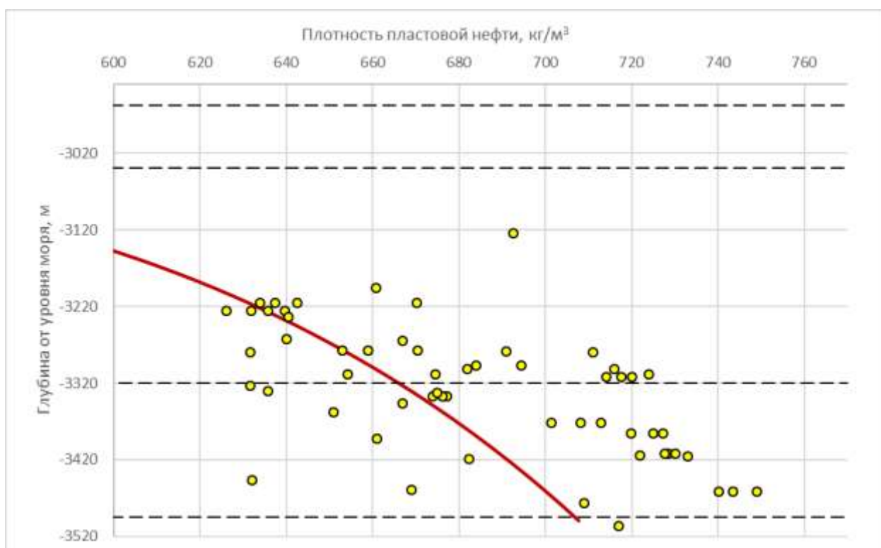
Рисунок 2.3.13 – Зависимость плотности пластовой нефти от глубины 1-го блока
