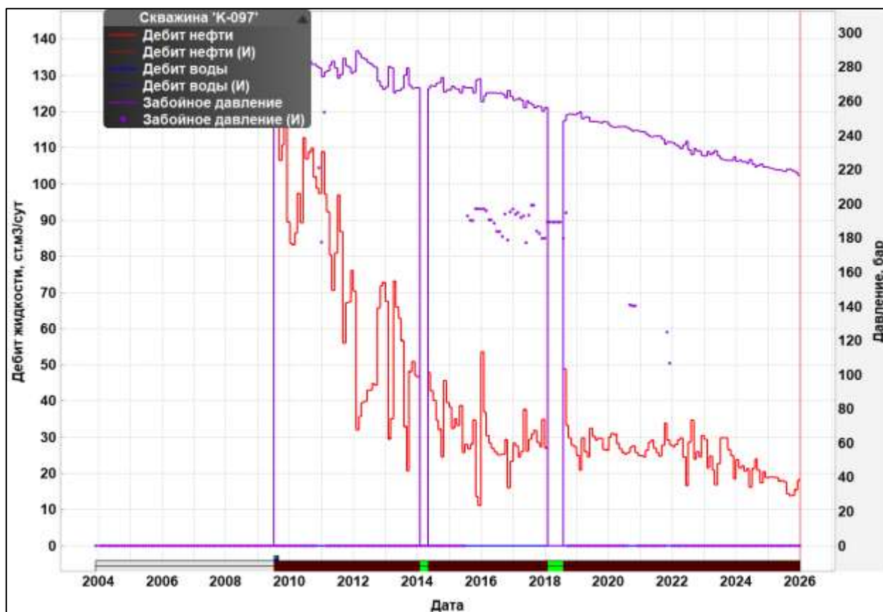
Рисунок 3.3.28 – Дебиты жидкости, нефти и забойное давление – скв №К-097
