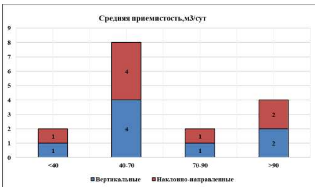
Рисунок 3.2.6 – Распределение фонда нагнетательных скважин по приемистости (по состоянию на 01.01.2026г)
