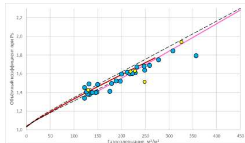
Рисунок 2.3.8 – Объёмный коэффициент от газосодержания пластовой нефти 2-го блока
