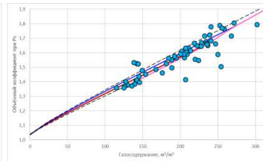
Рисунок 2.3.4 – Объёмный коэффициент от газосодержания пластовой нефти 1-го блока
