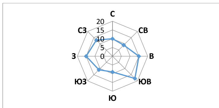
Рисунок 10.1.1 – Роза ветров
