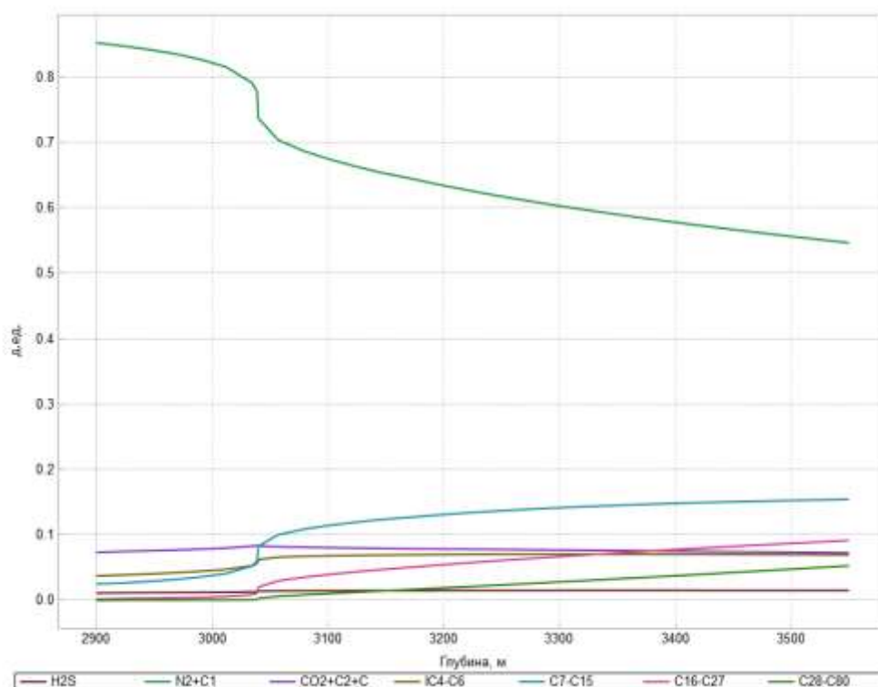
Рисунок 3.3.7 – Компонентное содержание по глубине
