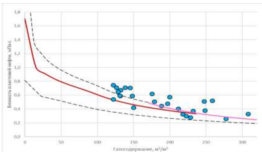
Рисунок 2.3.7 – Вязкость от газосодержания пластовой нефти 2-го блока
