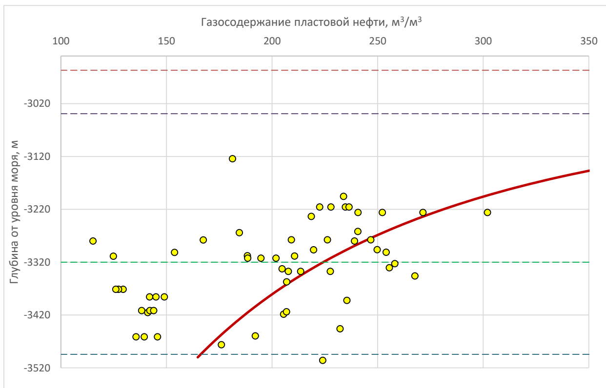
Рисунок 2.3.11 – Зависимость газосодержания пластовой нефти от глубины 1-го блока
