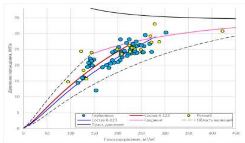
Рисунок 2.3.1 – Давление насыщения от газосодержания пластовой нефти 1-го блока
