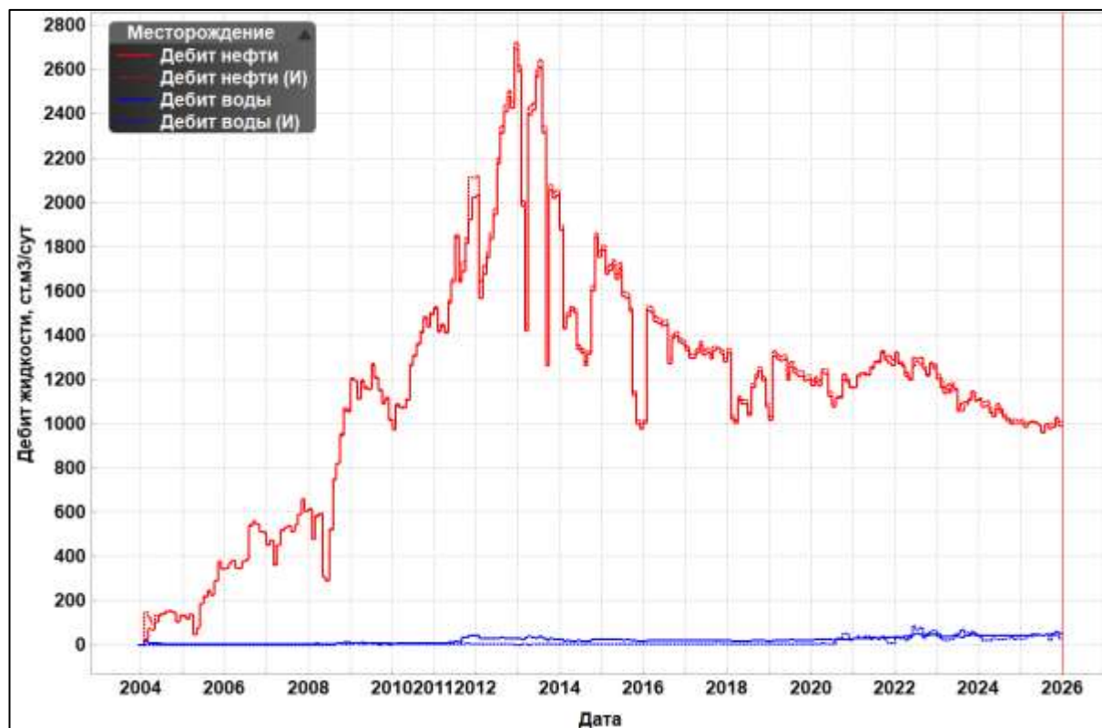
Рисунок 3.3.14 – График адаптации дебита нефти (линии-расчет, точки-факт)
