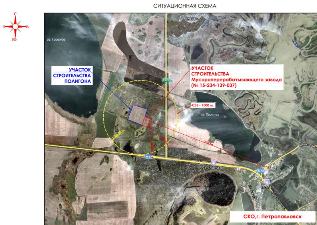
Ситуационная карта площадки
