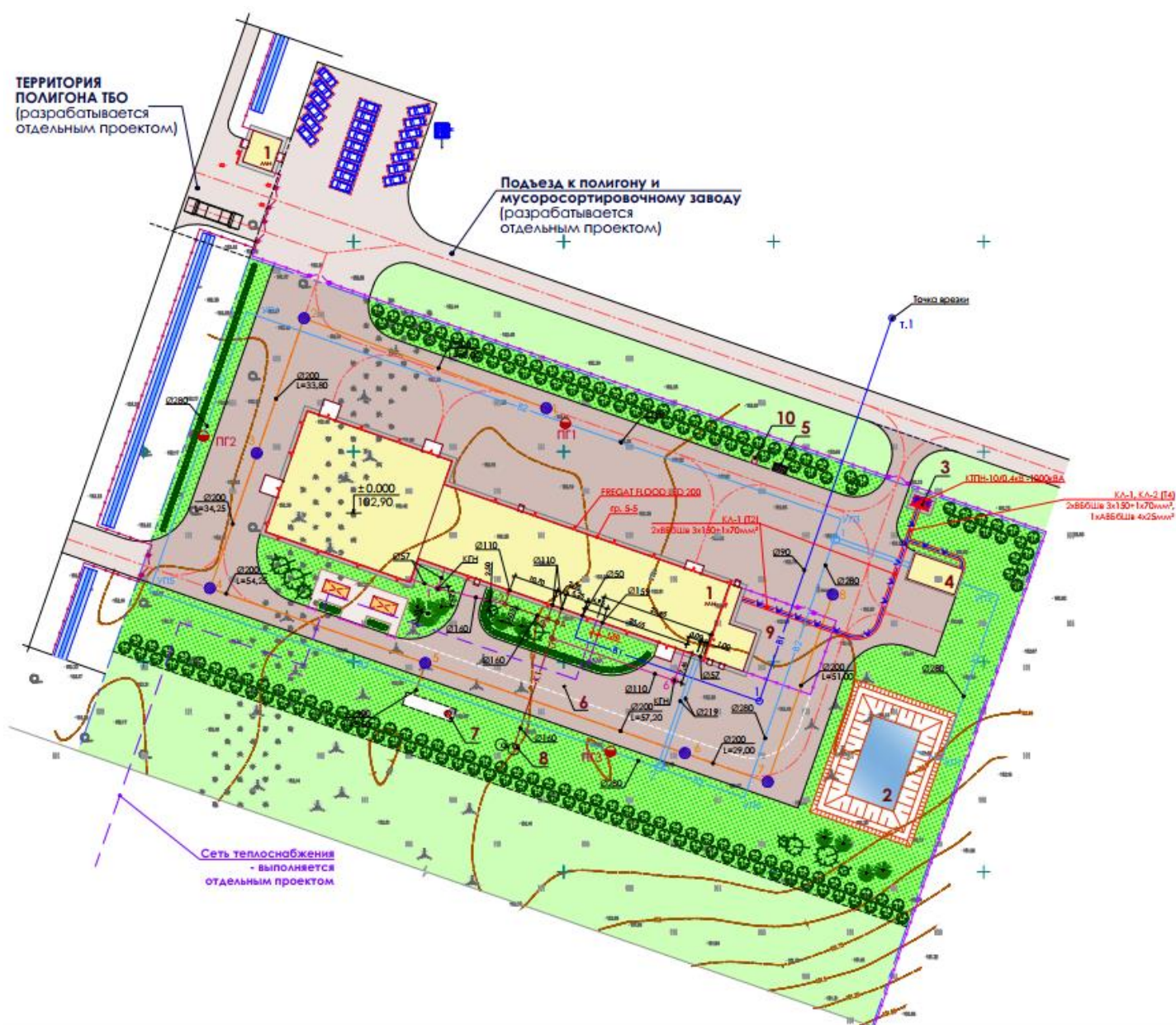
Рис. 2 Карта-схема объекта с указанием границ существующих объектов и указанием проектируемых зданий, сооружений
