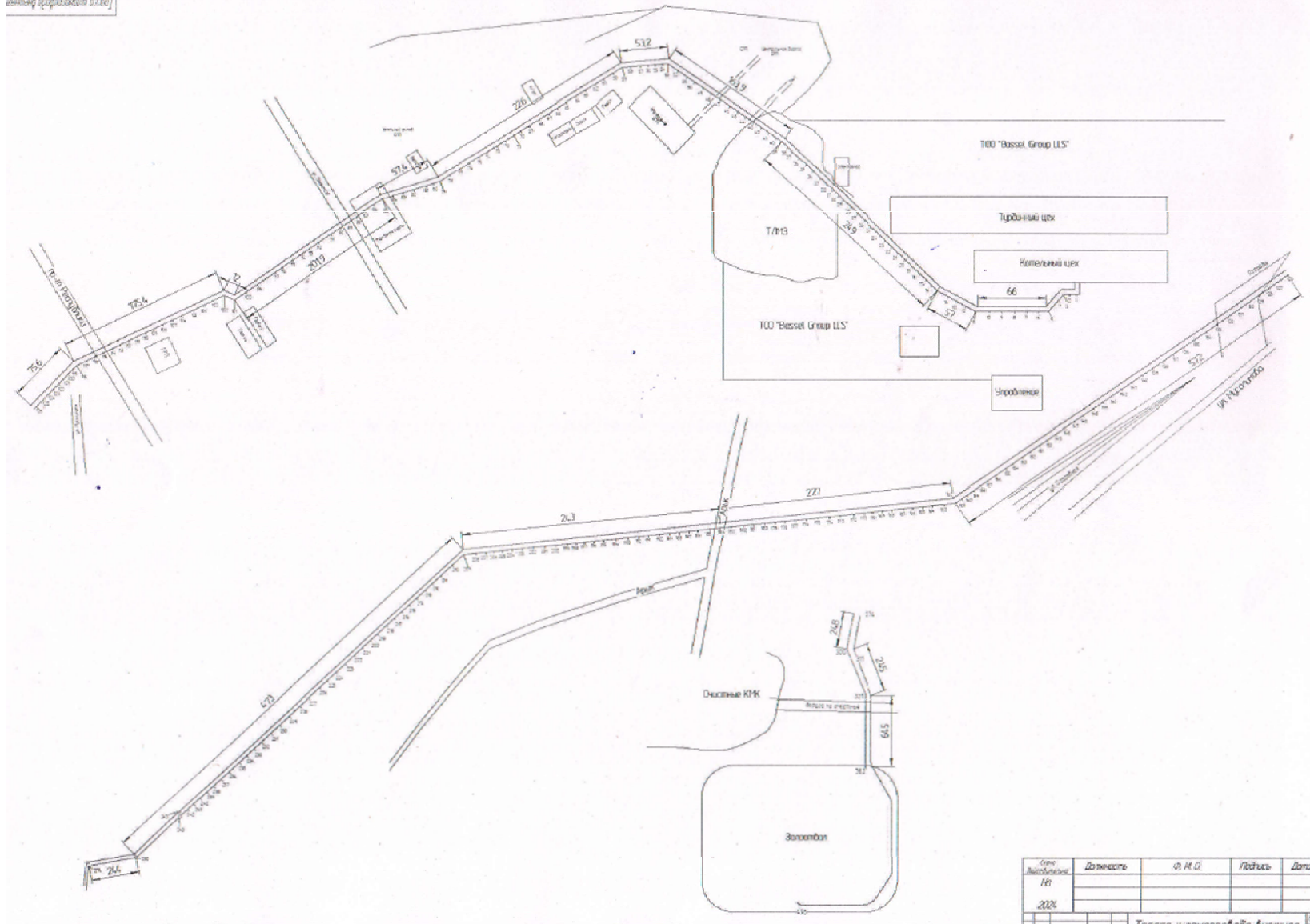
Рисунок 3.2. Схема водовыпусков
