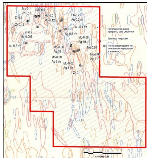
Схема планируемых профилей литогеохимической съемки по вторичным ореолам рассеяния (основа – схема геохимических аномалий по результатам предшествующих работ)
