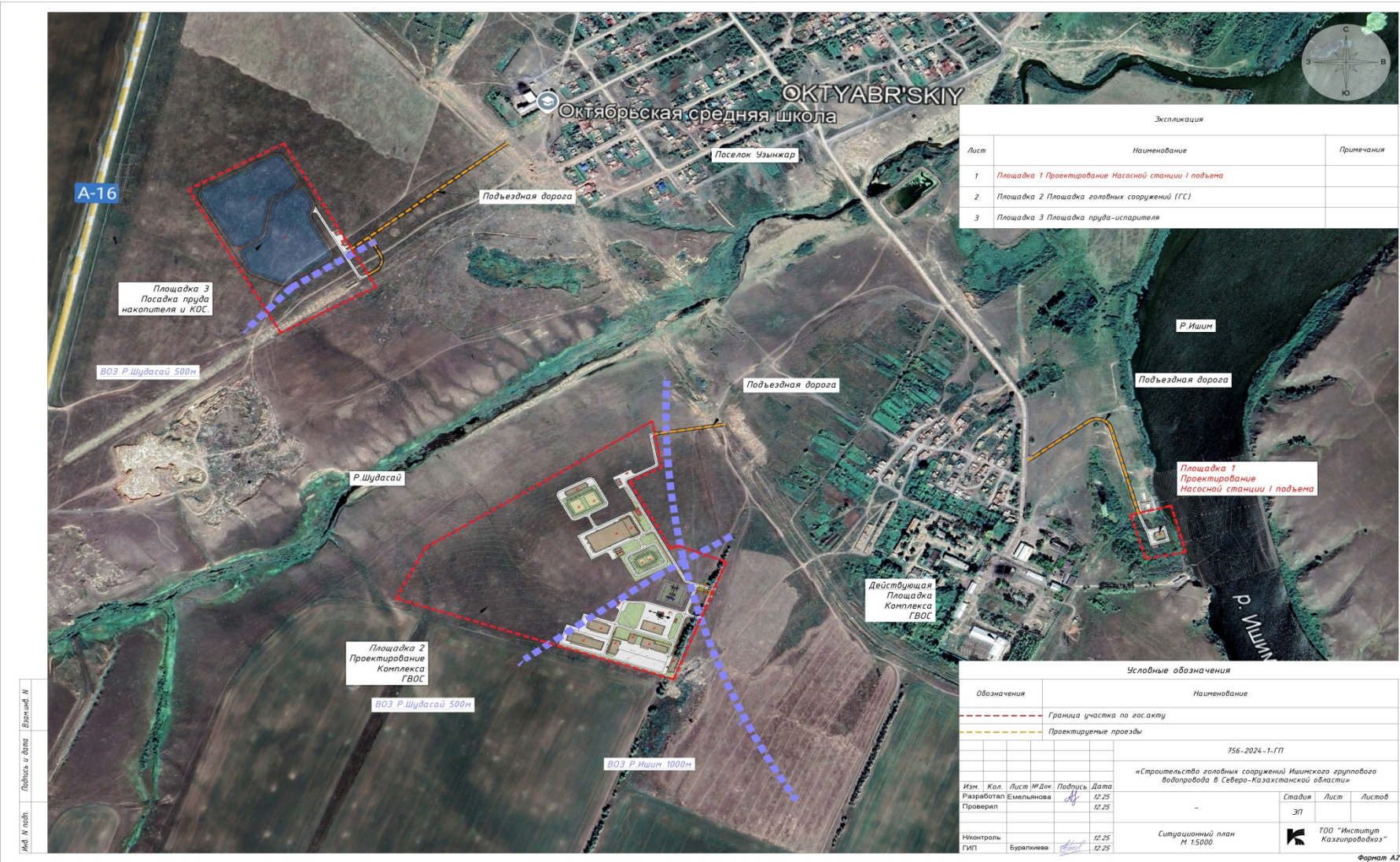
Рисунок 1 - Ситуационная карта-схема расположения проектируемого ВОС Ишим
