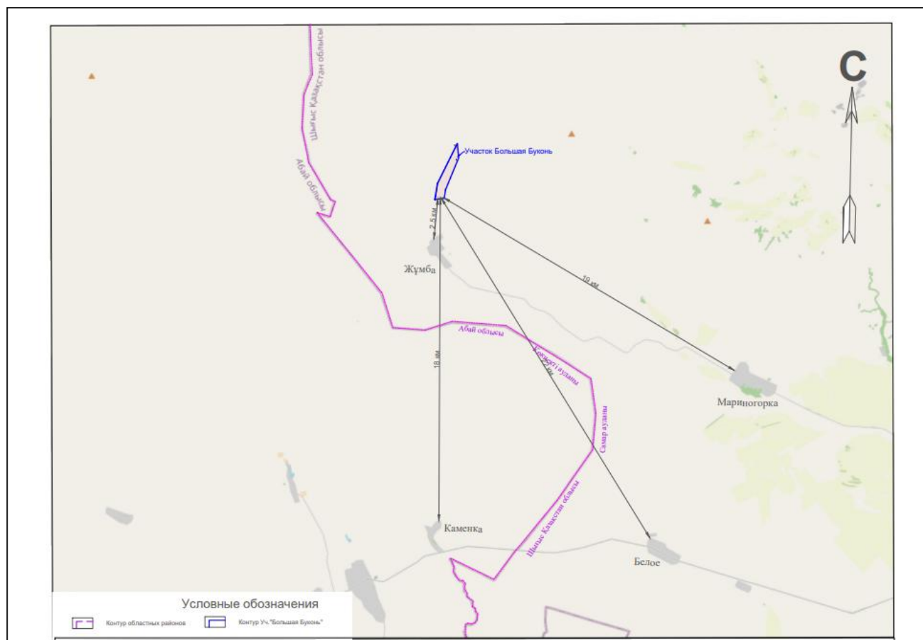
Рис. 1 Ситуационная карта-схема месторождения «Большая Буконь». Масштаб 1:400 000.
