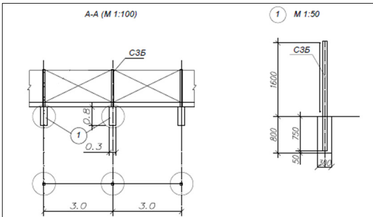
Рисунок 5.1 – Типовая конструкция ограждающего забора.
