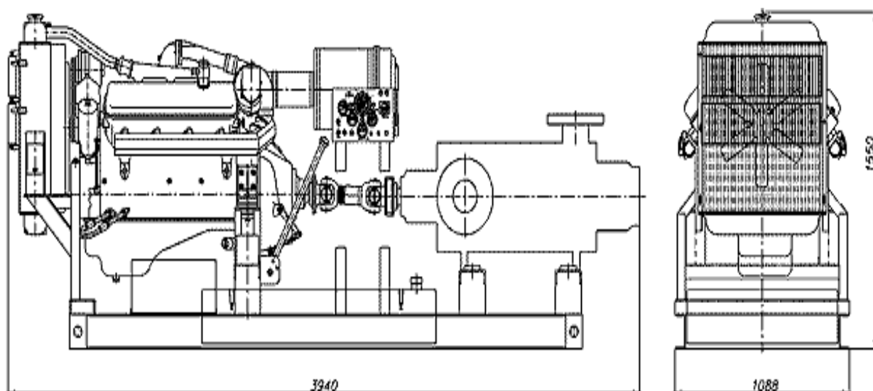
Рисунок 3.3 - Дизельная насосная установка ДНУ – 180/255
