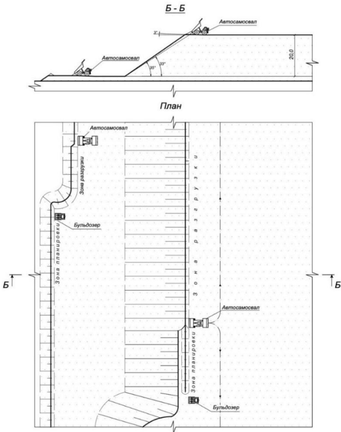
Рисунок 5.1 – Технологическая схема бульдозерного отвалообразования
