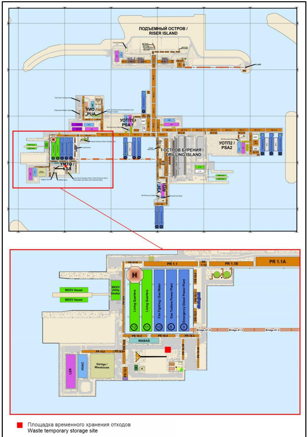
Рисунок 3.4 Схема расположения площадки временного накопления отходов
