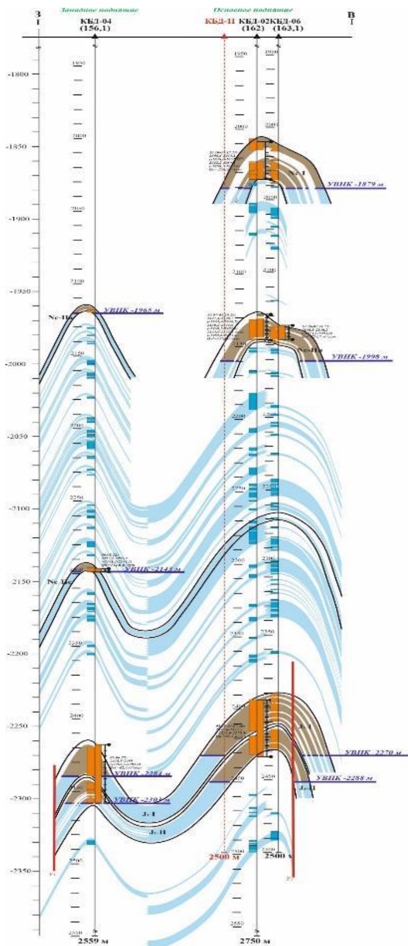
Рисунок 3.1.1 - Геологический профиль с проектной скважиной КБД-1i
