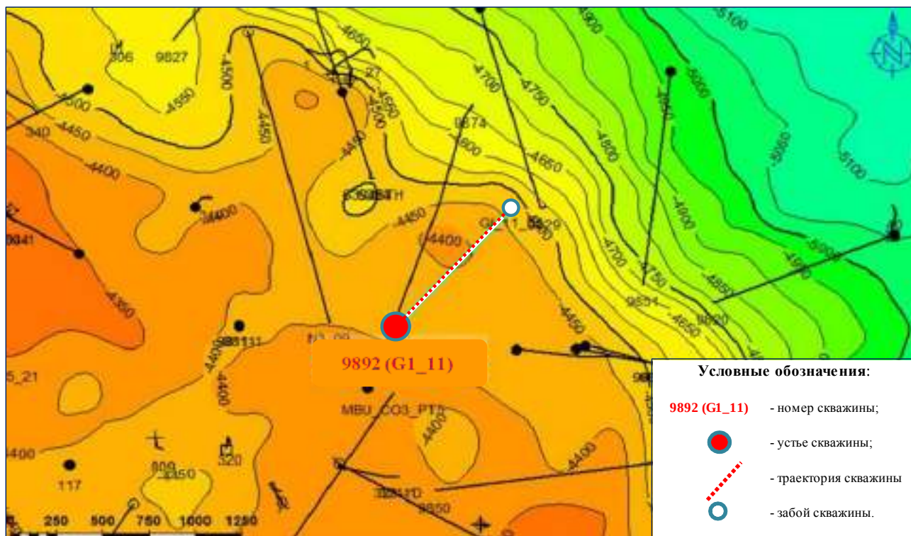
Рисунок 3.2 – Карта-схема расположения проектируемой скважины 9892 (GI_11)
