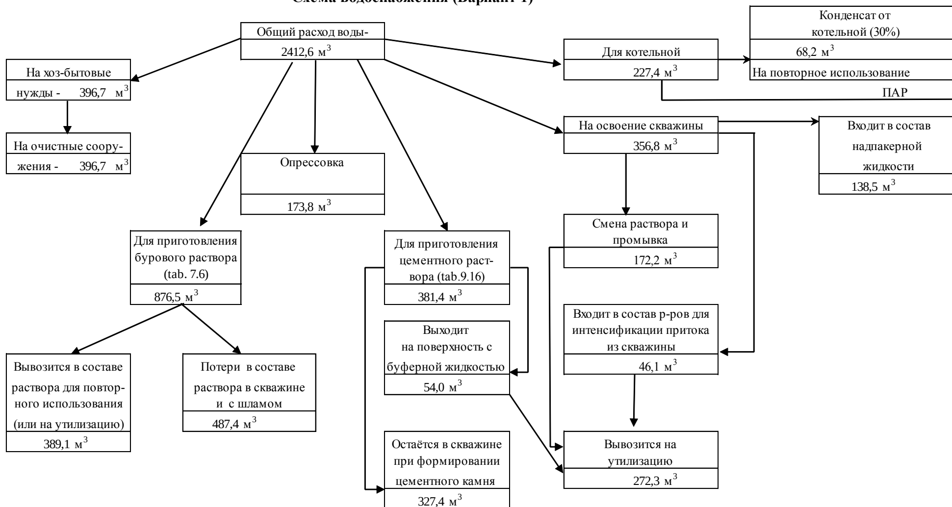
Рисунок 3.5 – Схема водопотребления и водоотведения при строительстве скважины 9892 (GI_11) вариант 1
