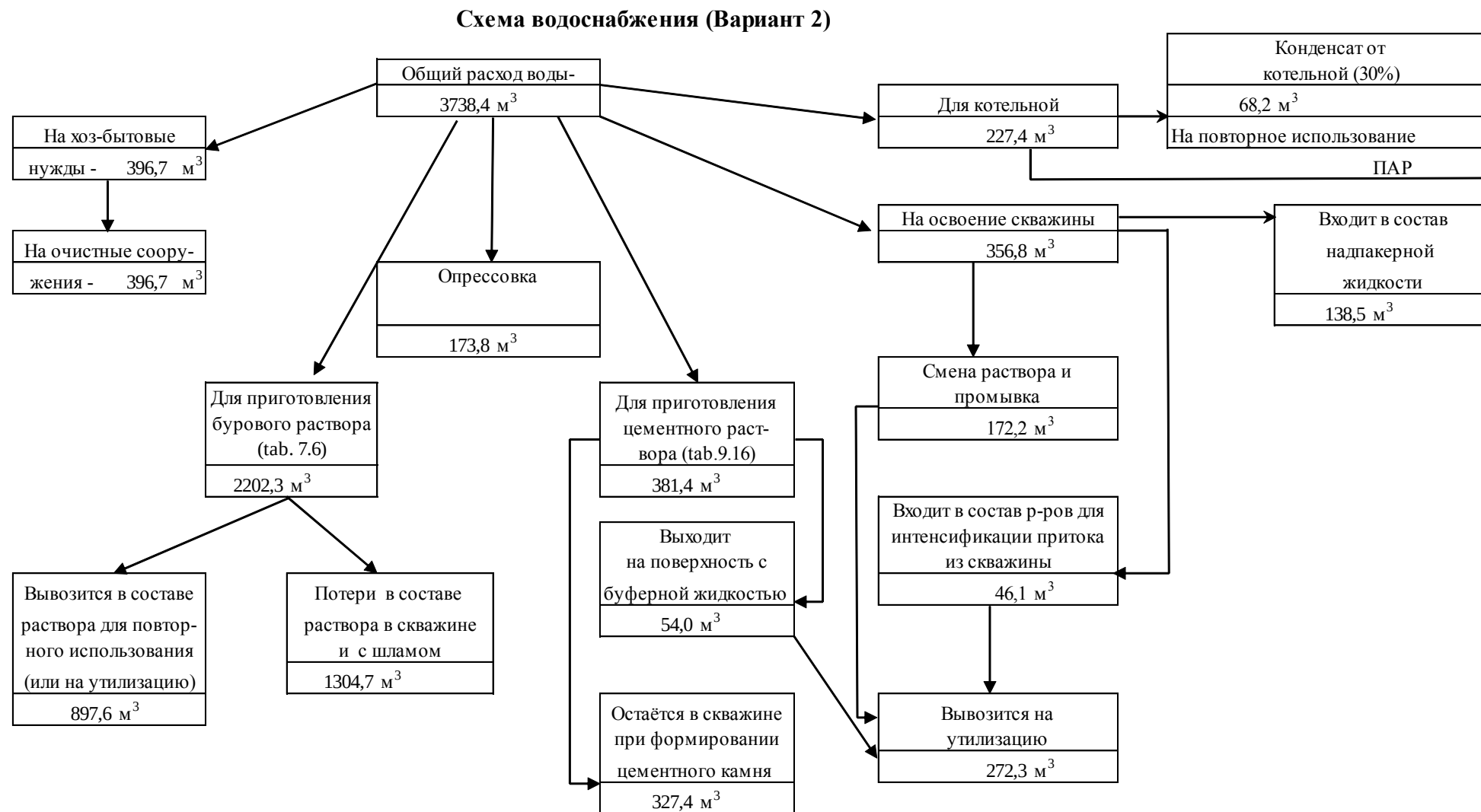
Рисунок 3.6 – Схема водопотребления и водоотведения при строительстве скважины 9892 (GI_11) вариант 2
