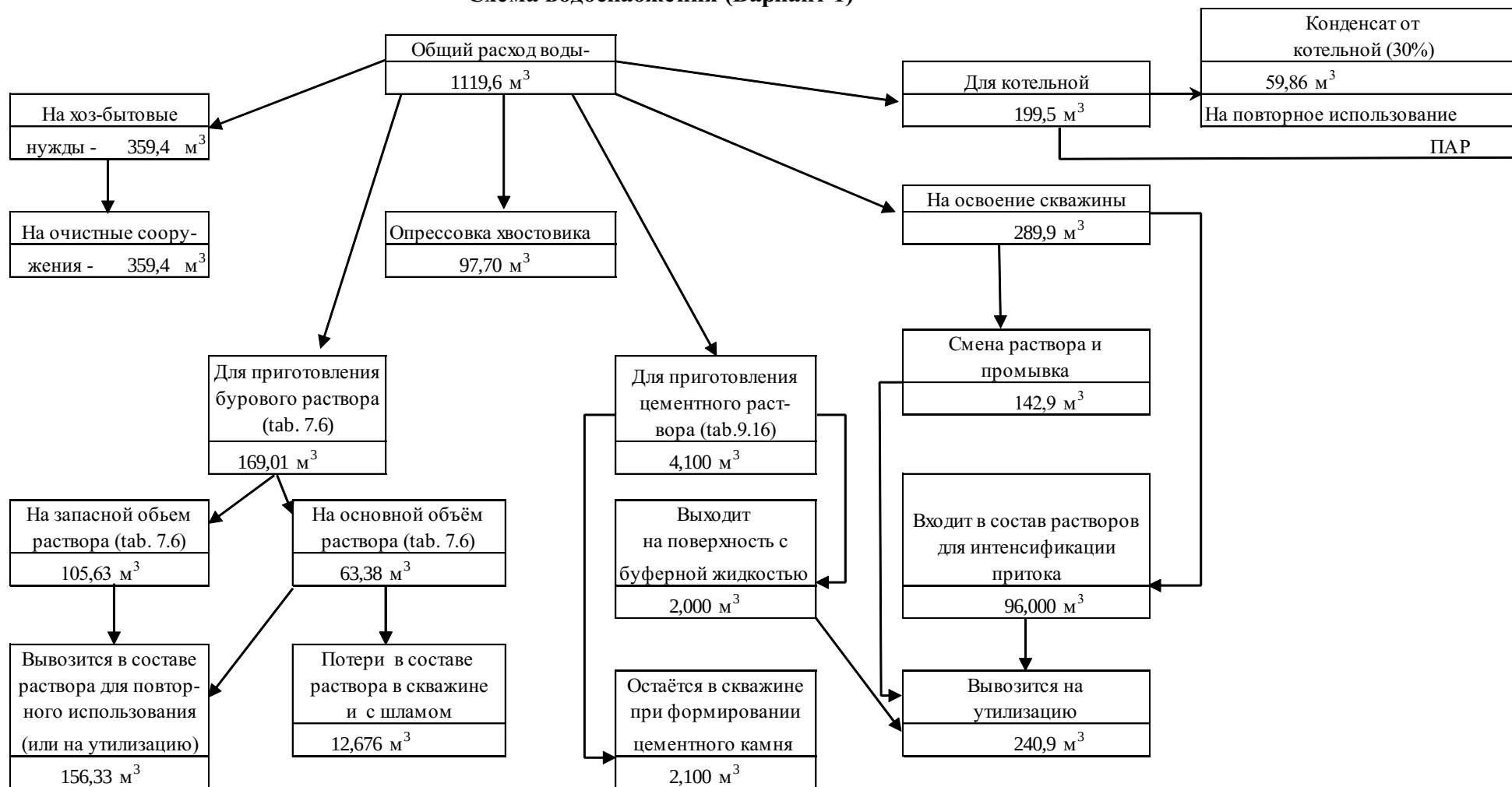
Рисунок 3.5 – Схема водопотребления и водоотведения при бурении горизонтального бокового ствола 6394-2 в скважине 6394 вариант 1
