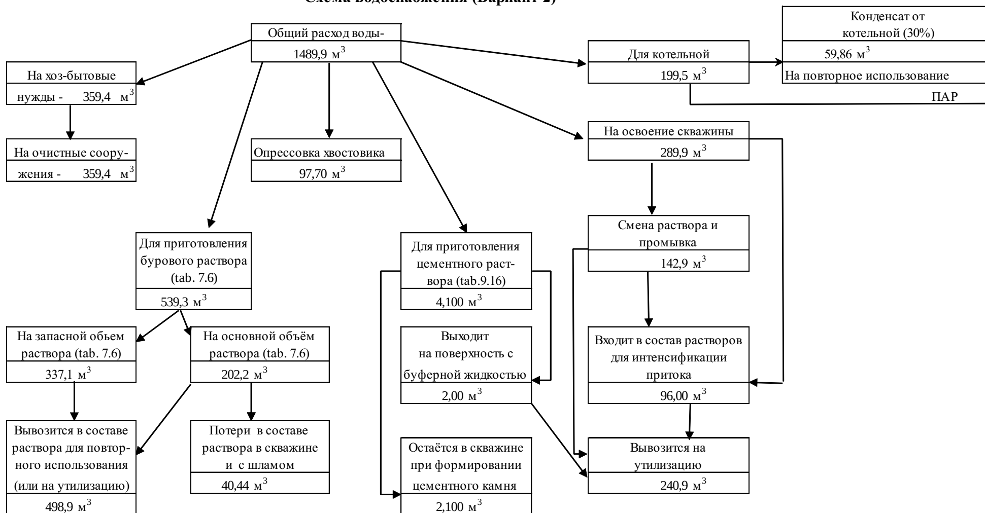
Рисунок 3.6 – Схема водопотребления и водоотведения при бурении горизонтального бокового ствола 6394-2 в скважине 6394 вариант 2
