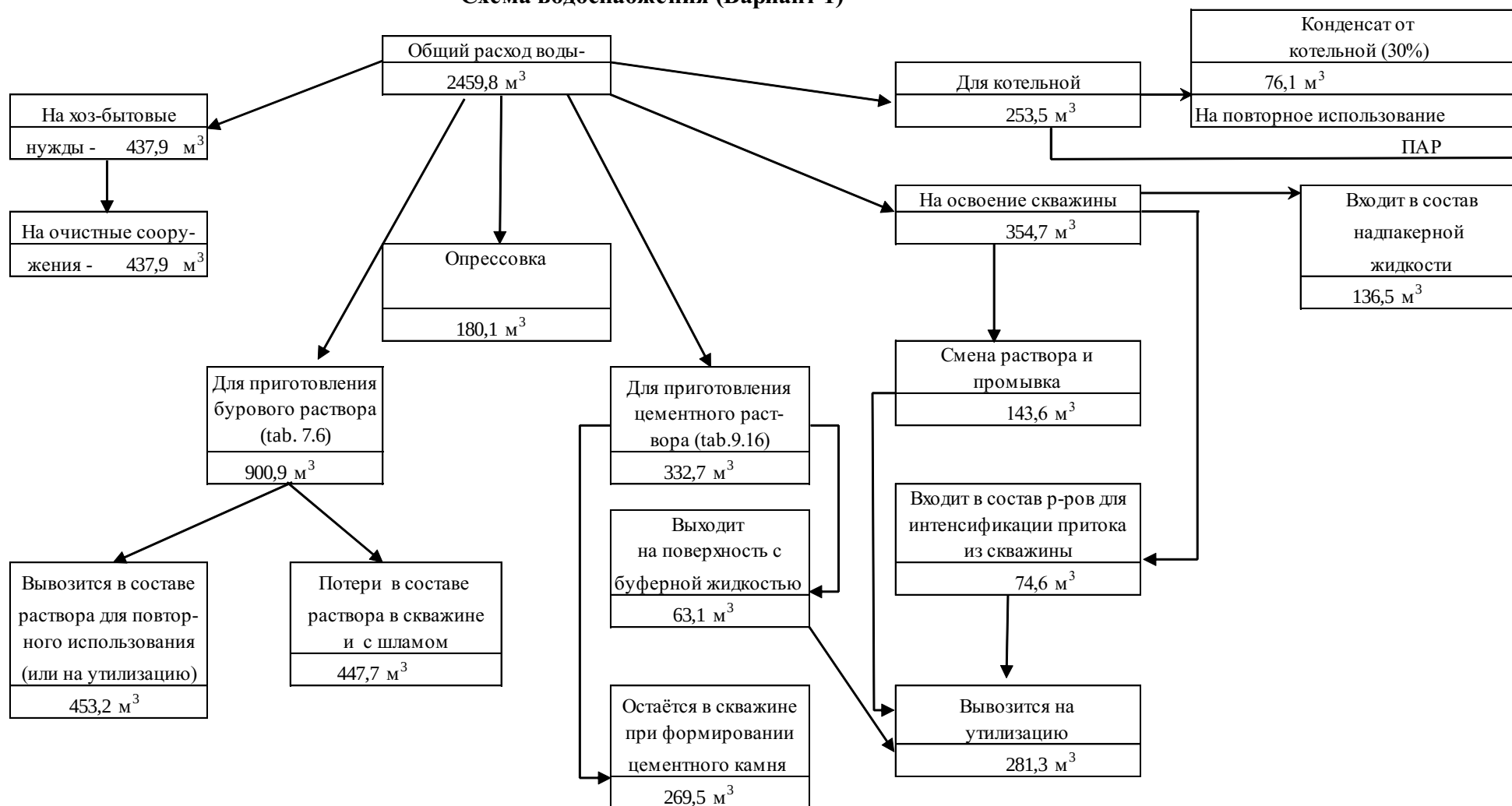
Рисунок 3.5 – Схема водопотребления и водоотведения при бурении добывающей скважины 98107 (C2_64)
