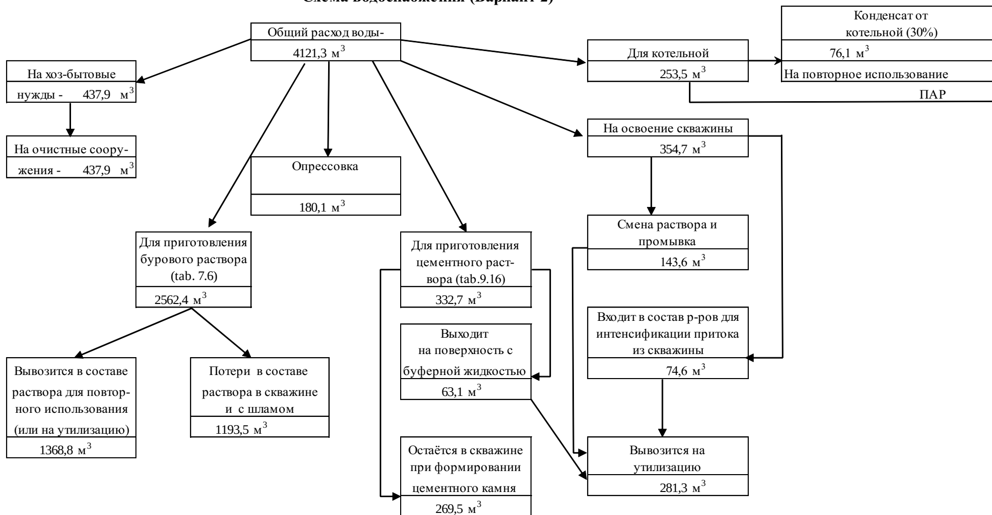
Рисунок 3.6 – Схема водопотребления и водоотведения при бурении добывающей скважины 98107 (C2_64)
