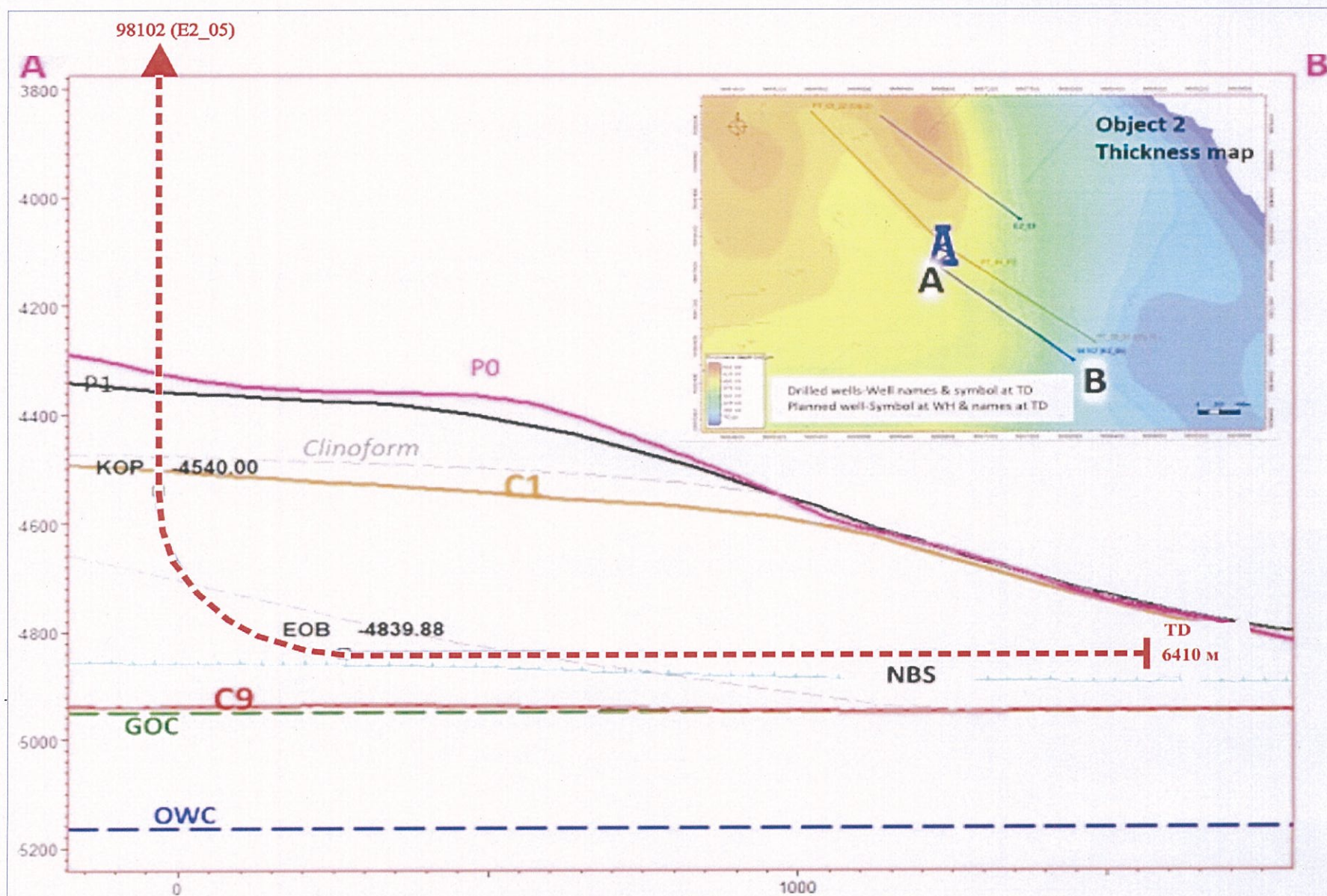
Рис. 4.1 - Профиль скважины
