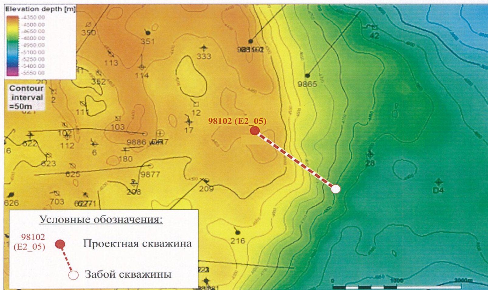
Рис. 4.2 - Структурная карта по кровле C_1
