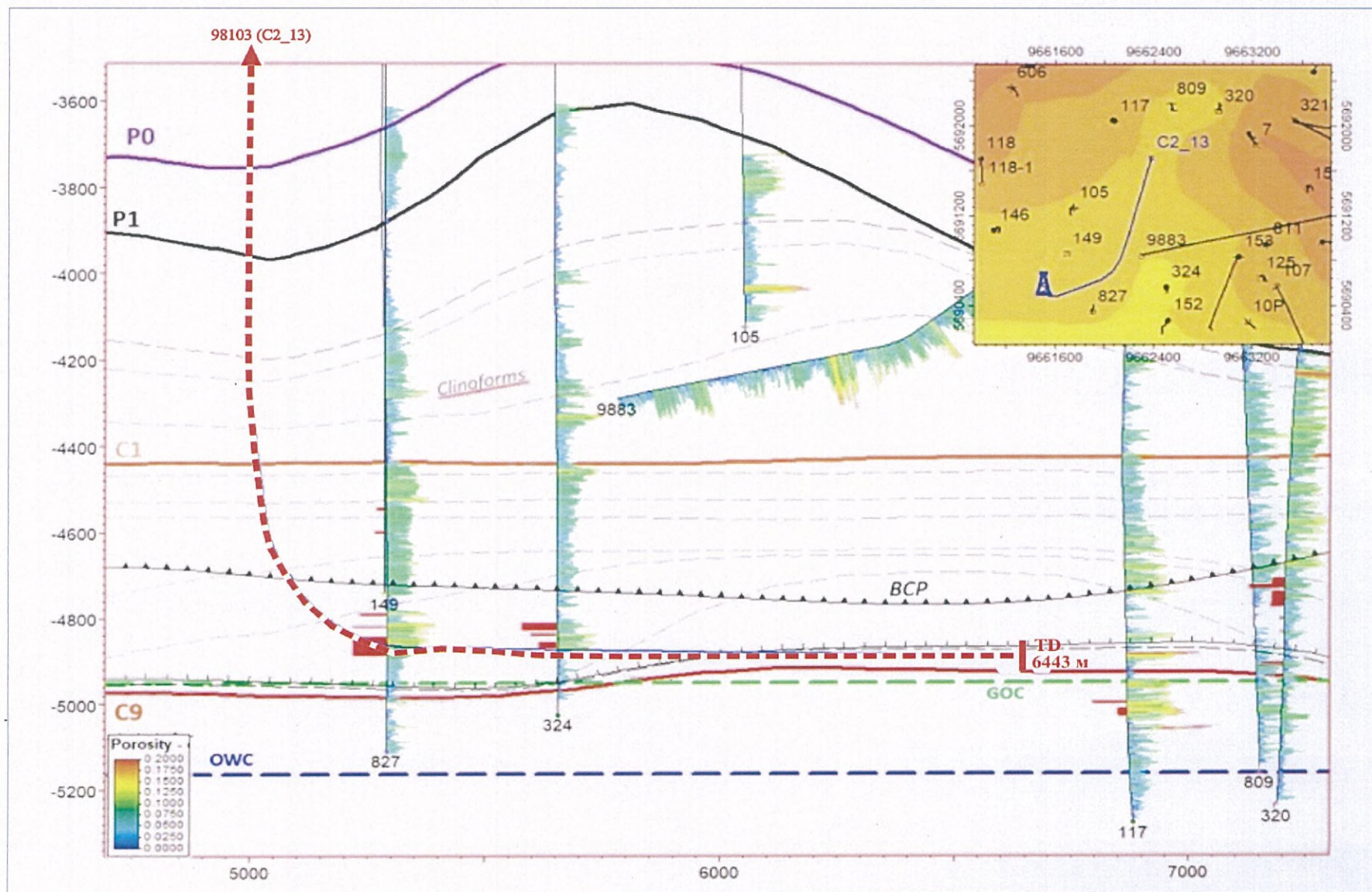
Рис. 4.1 - Профиль скважины
