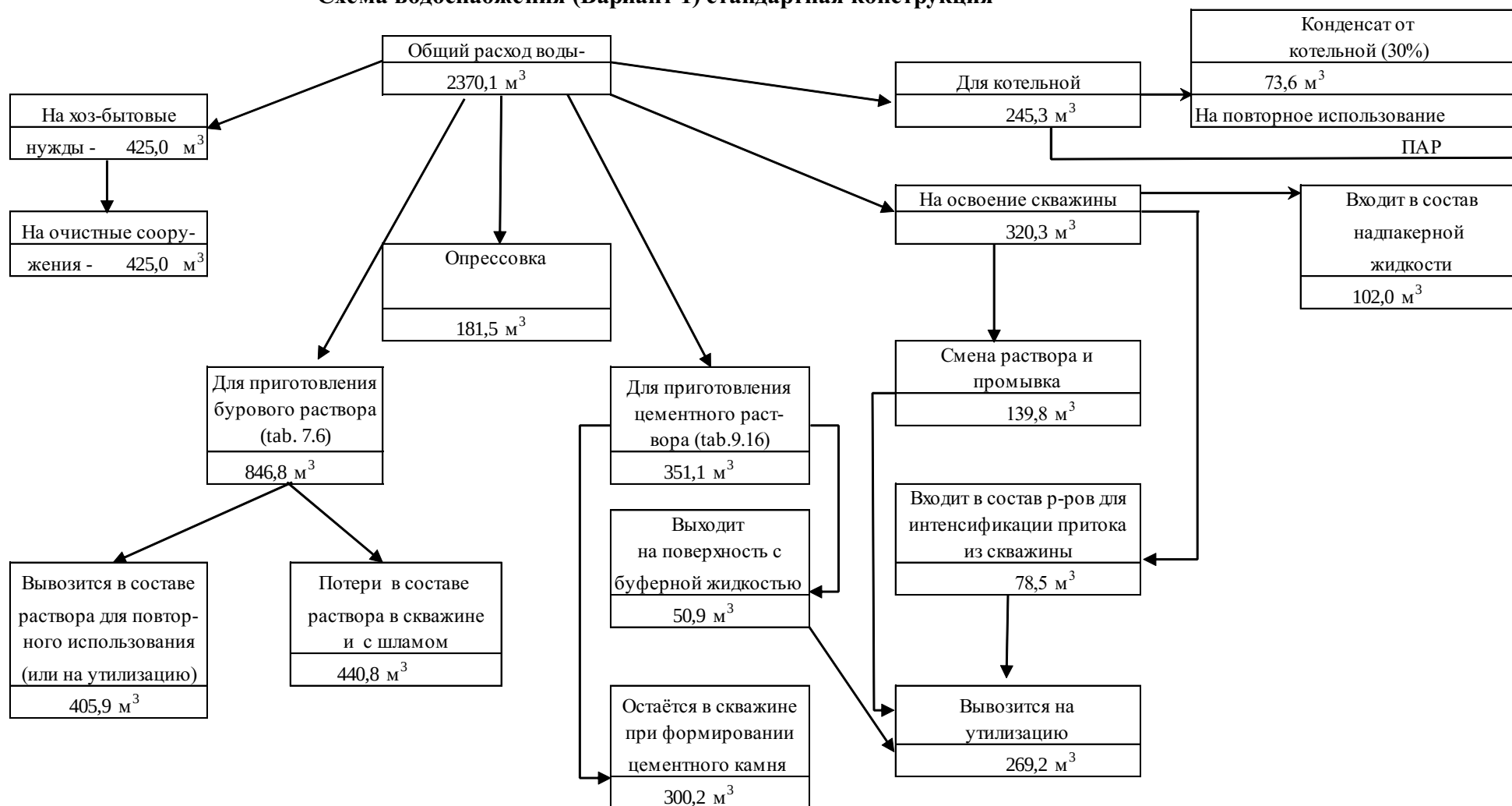
Рисунок 3.5 – Схема водопотребления и водоотведения при бурении добывающей скважины 98109 (Z3_02)
