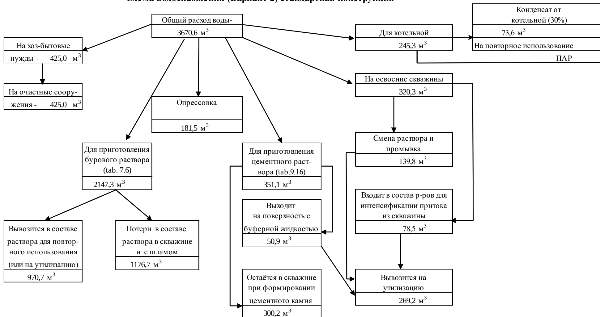
Рисунок 3.6 – Схема водопотребления и водоотведения при бурении добывающей скважины 98109 (Z3_02)
