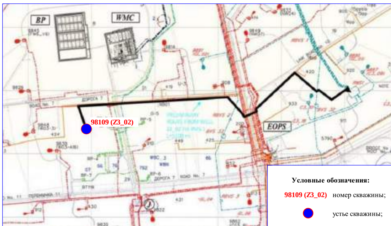
Рисунок 3.2 – Карта-схема расположения проектируемой добывающей скважины 98109 (Z3_02)
